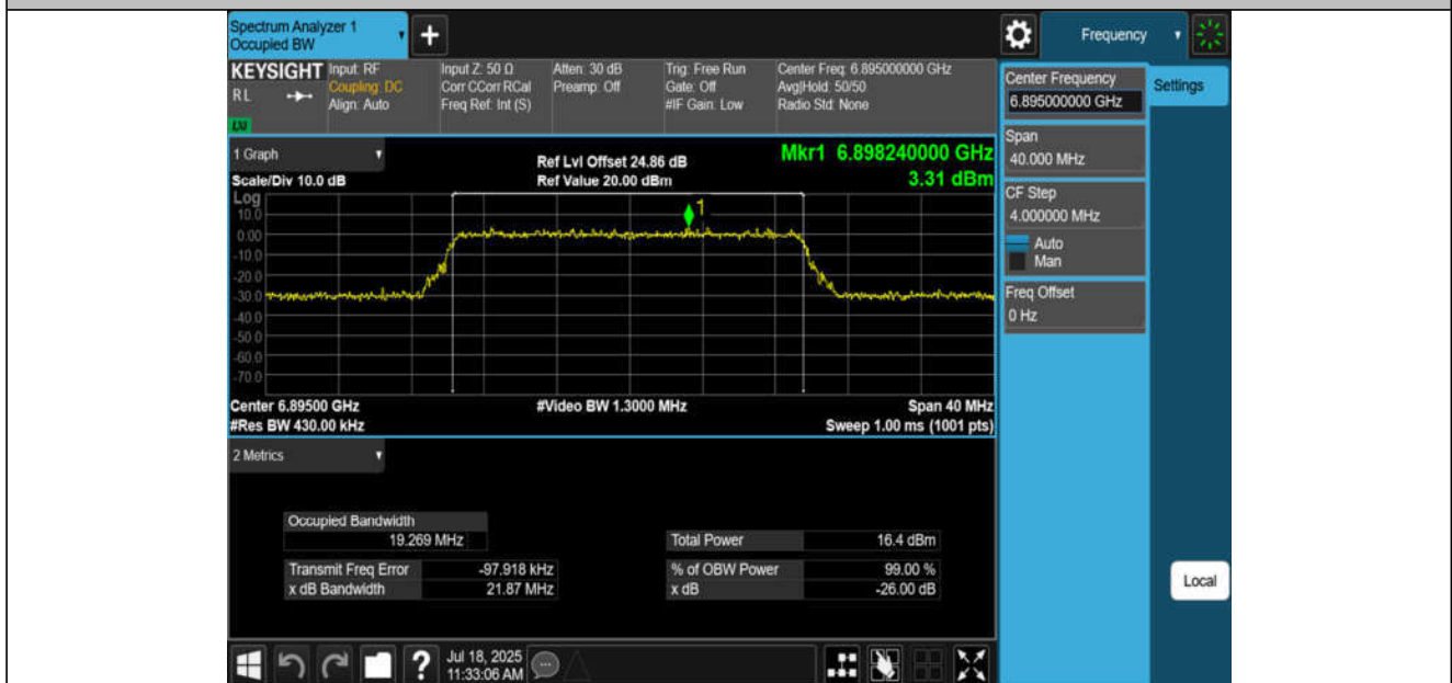
11AX20MIMO-Ant4-6895-PASS
