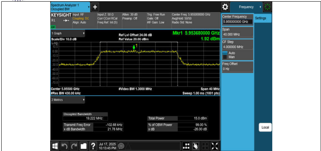
11AX20MIMO-Ant1-5955-PASS
