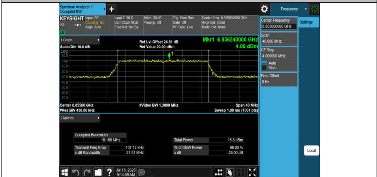
11AX20MIMO-Ant4-6855-PASS
