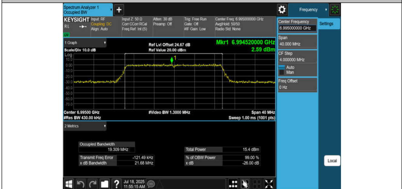
11AX20MIMO-Ant4-6995-PASS
