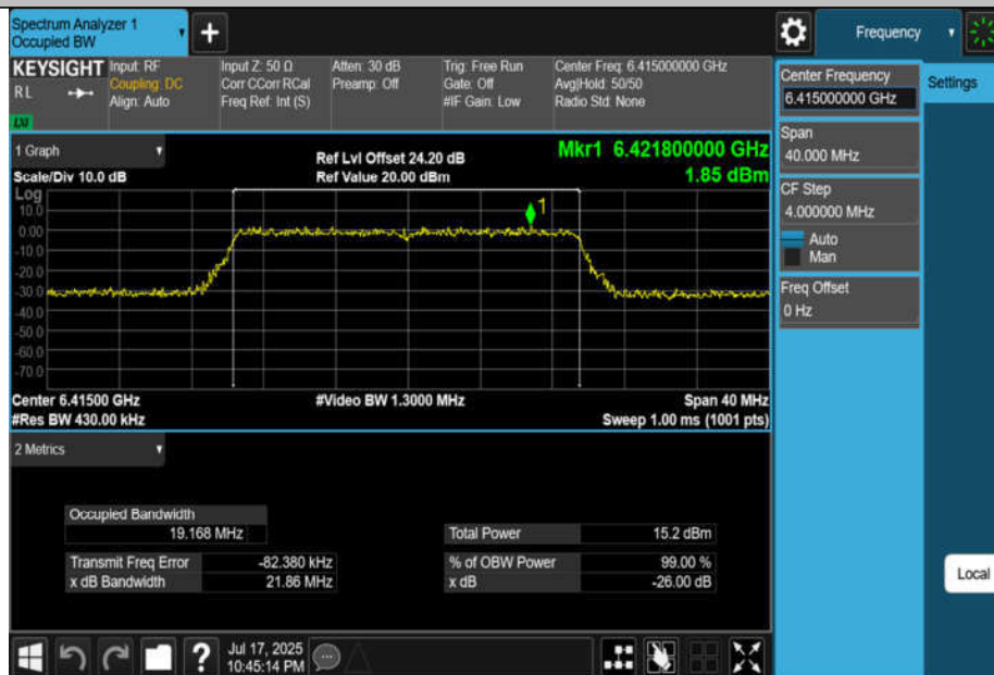
11AX20MIMO-Ant4-6415-PASS
