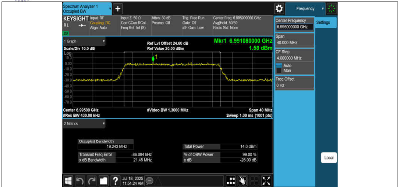
11AX20MIMO-Ant3-6995-PASS
