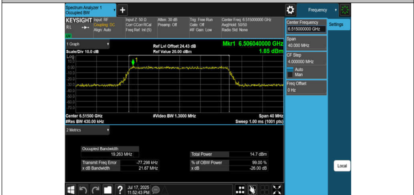
11AX20MIMO-Ant4-6515-PASS
