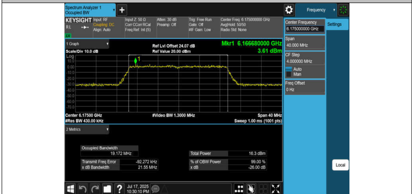
11AX20MIMO-Ant4-6175-PASS
