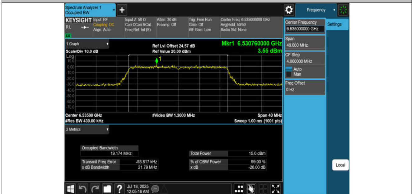
11AX20MIMO-Ant4-6535-PASS
