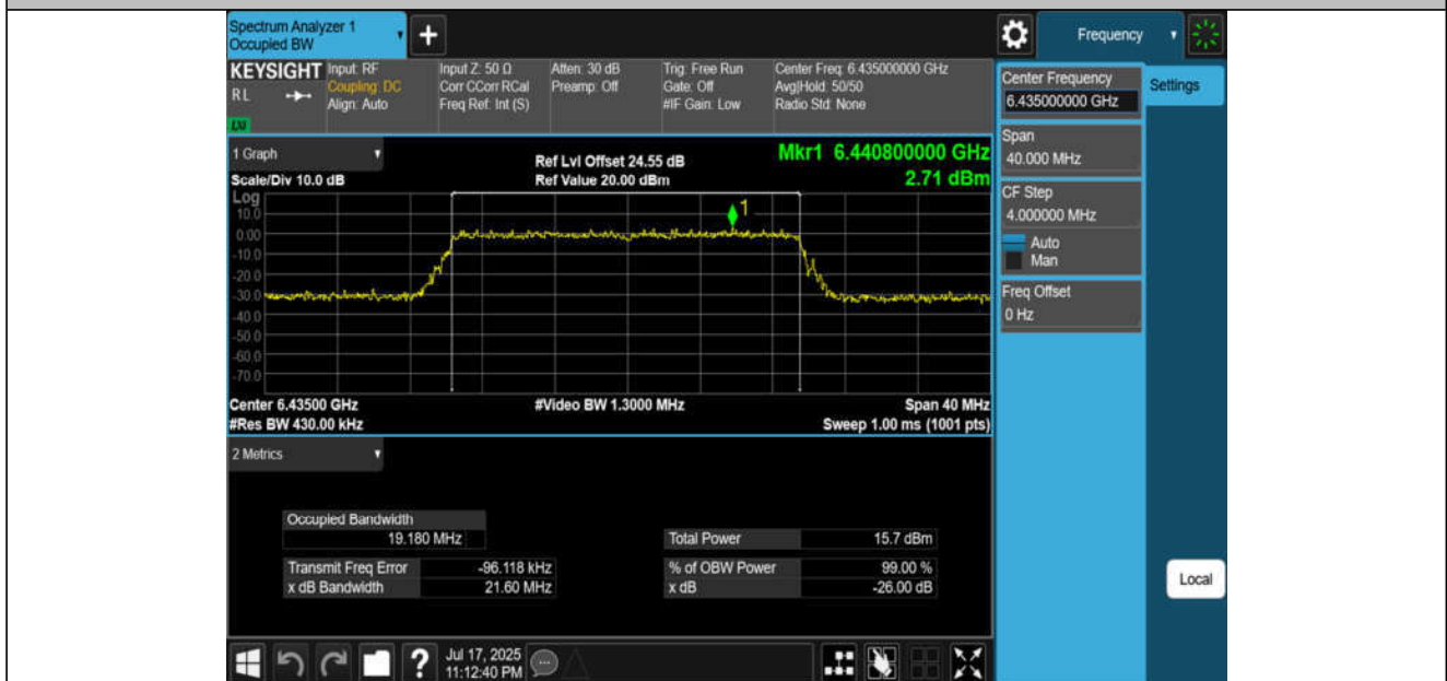
11AX20MIMO-Ant4-6435-PASS
