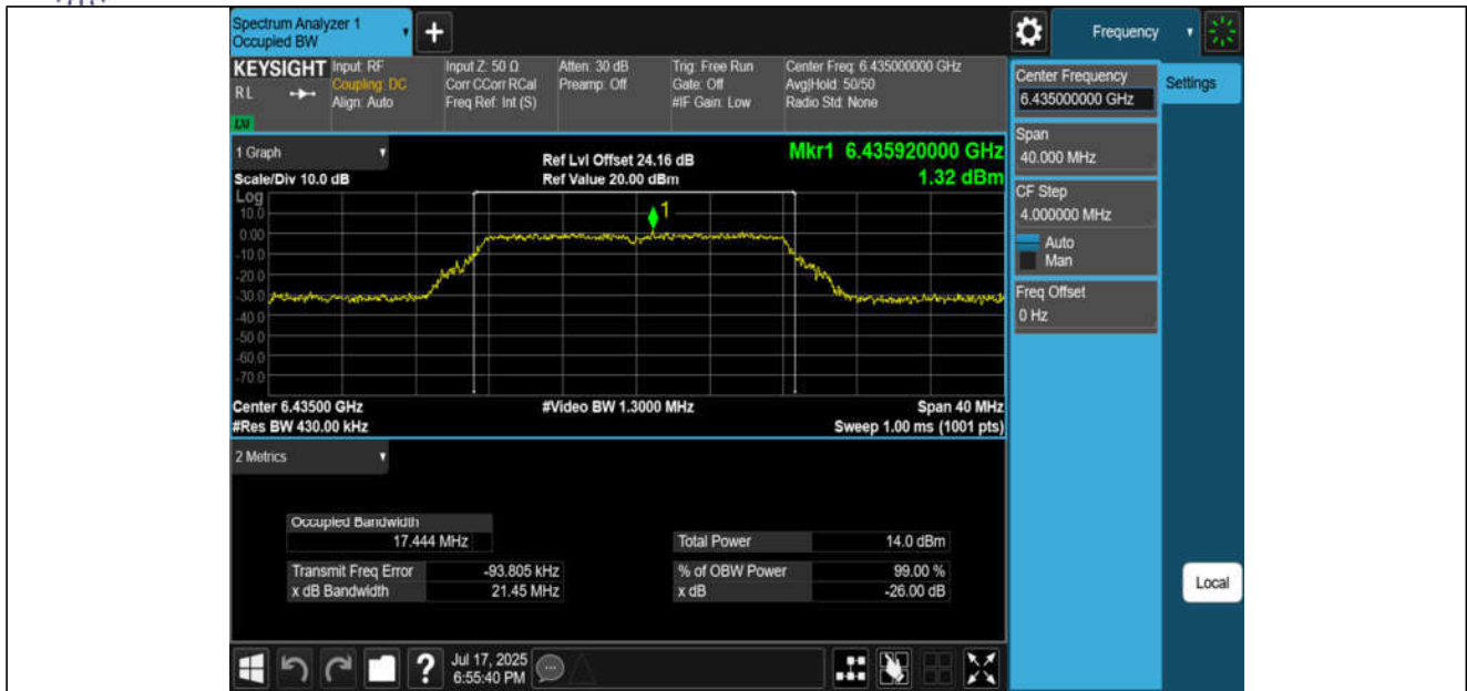
11A-CDD-Ant1-6435-PASS
