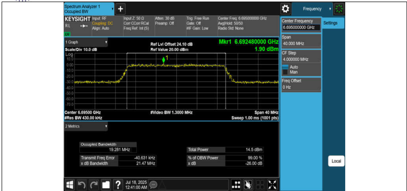
11AX20MIMO-Ant1-6695-PASS
