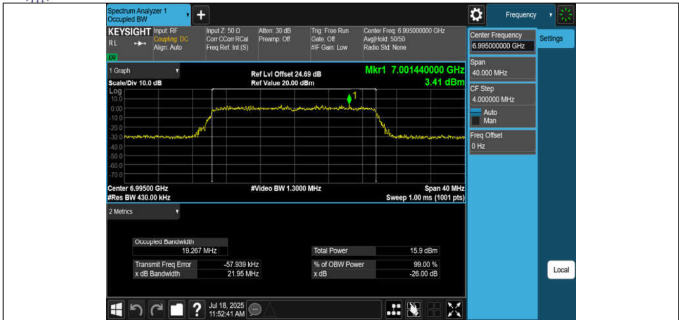
11AX20MIMO-Ant1-6995-PASS
