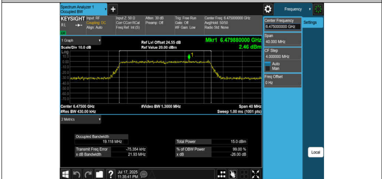
11AX20MIMO-Ant4-6475-PASS
