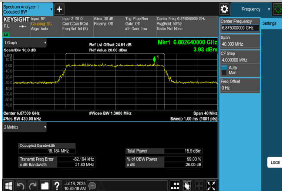
11AX20MIMO-Ant4-6875-PASS
