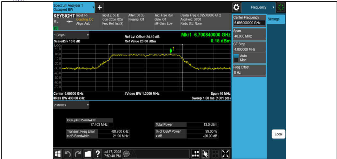
11A-CDD-Ant1-6695-PASS
