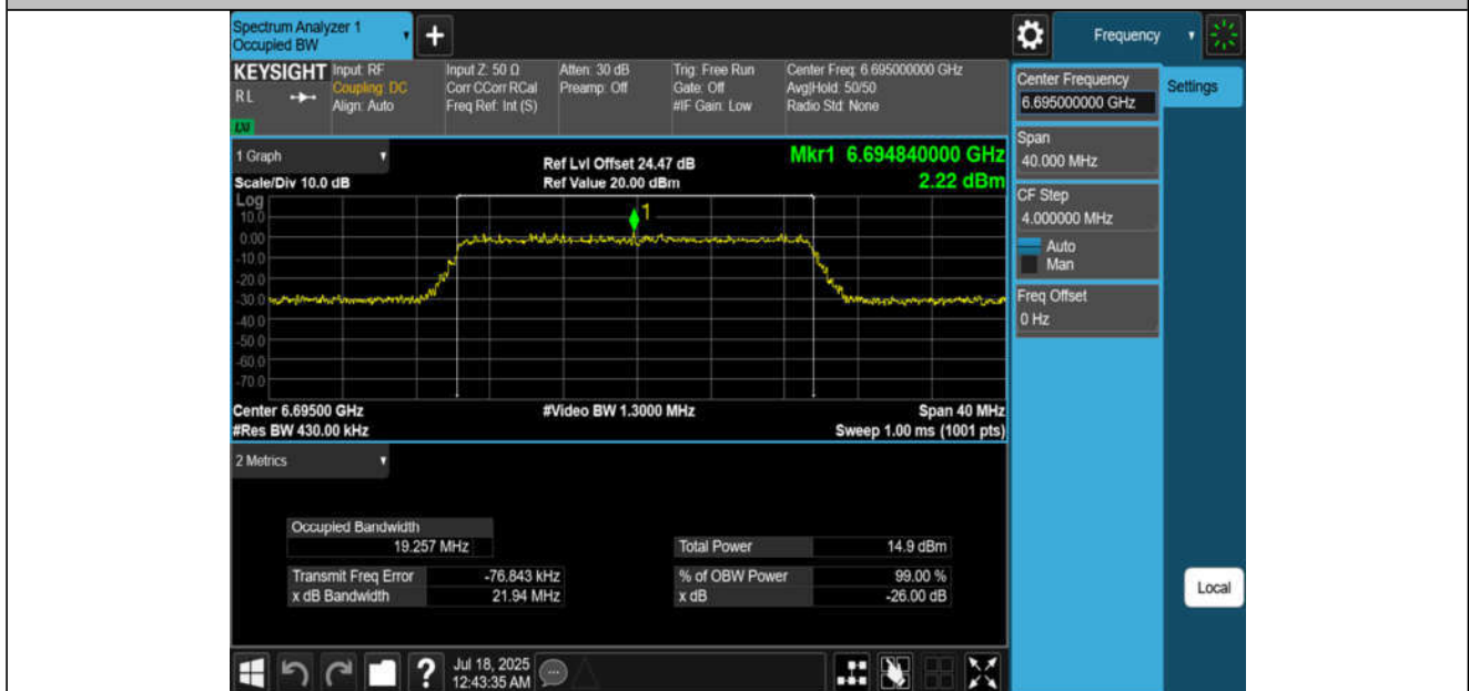
11AX20MIMO-Ant4-6695-PASS
