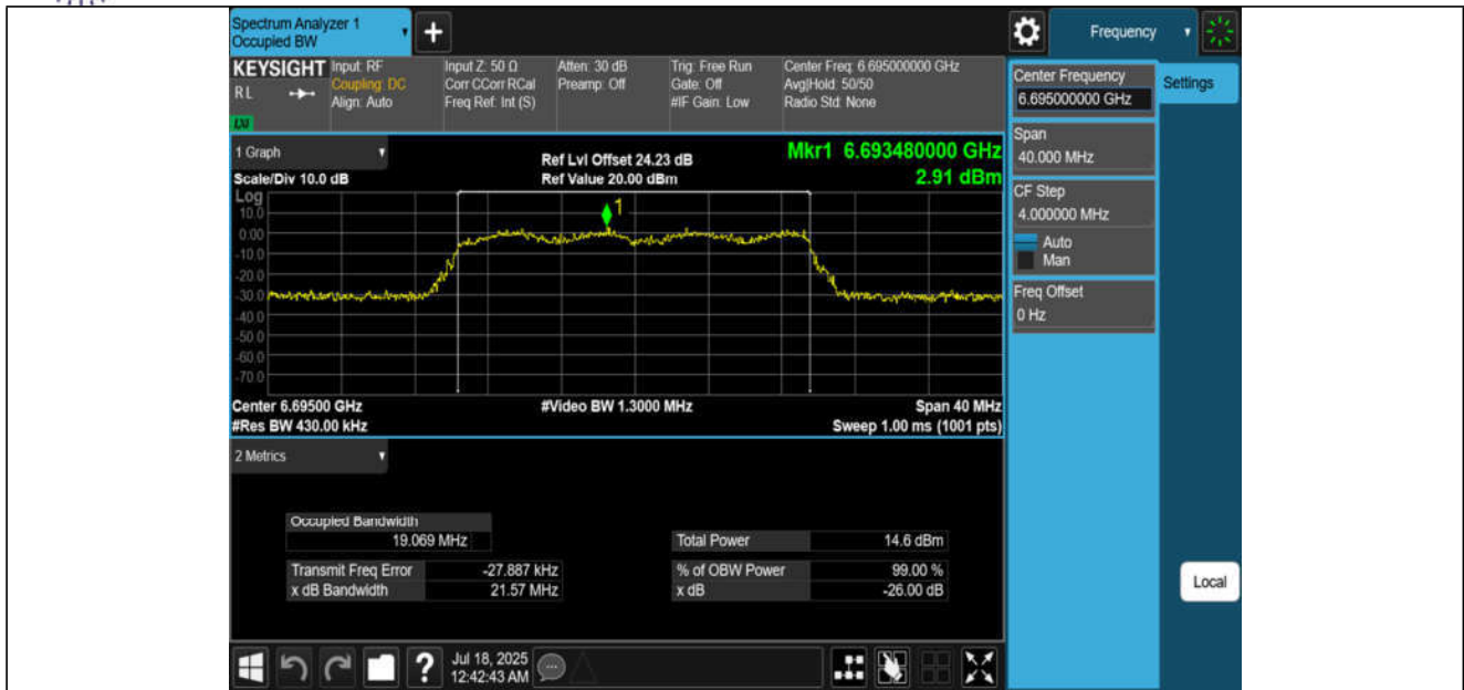
11AX20MIMO-Ant3-6695-PASS
