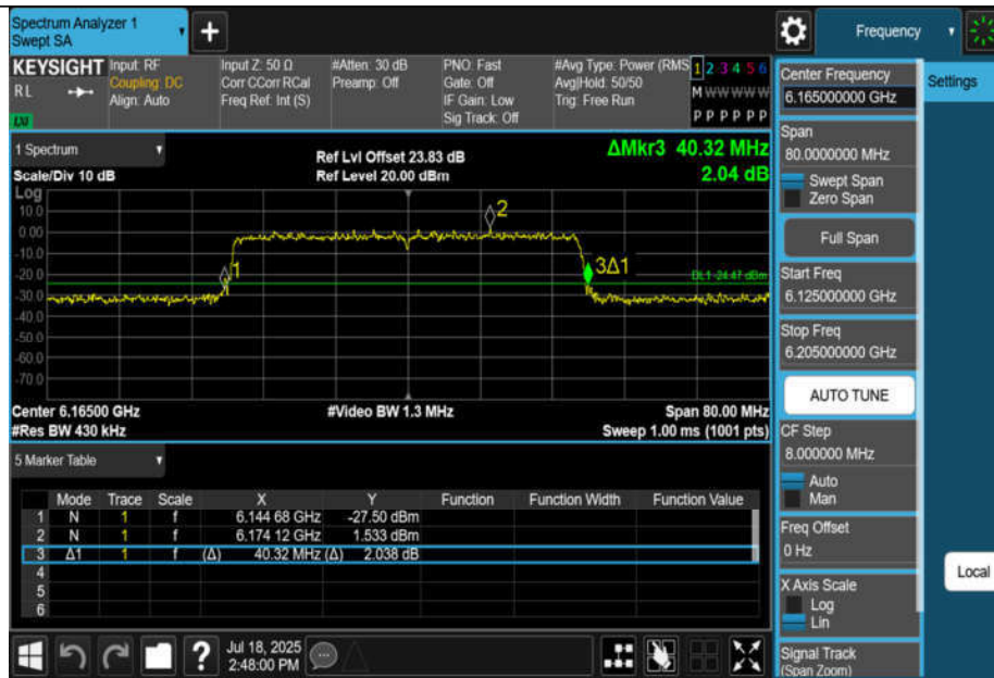
11AX40MIMO-Ant1-6165
