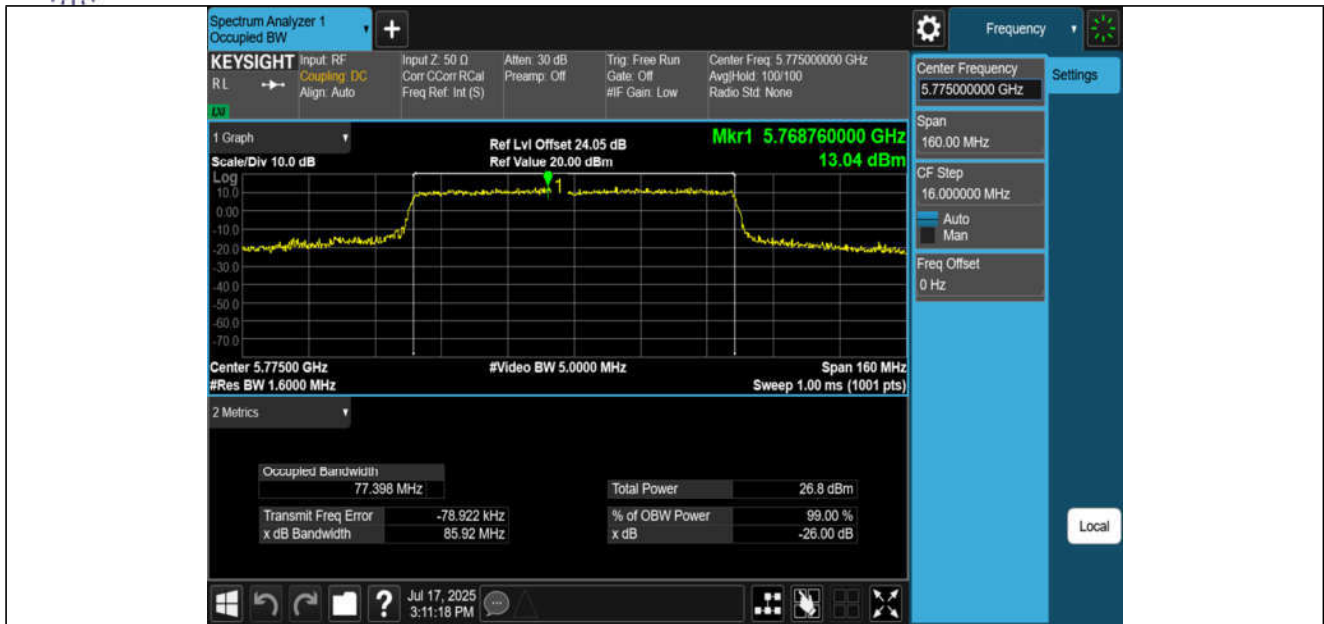
11BE80MIMO-Ant1-5775
