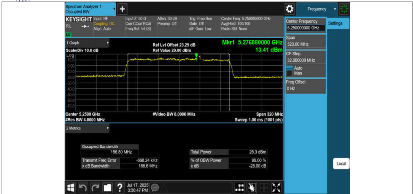
11BE160MIMO-Ant3-5250
