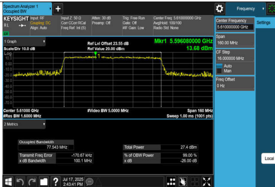
11BE80MIMO-Ant1-5610
