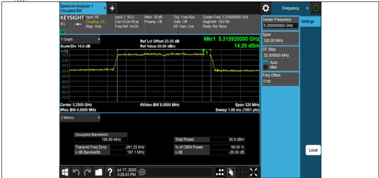
11BE160MIMO-Ant1-5250
