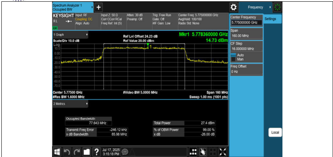
11BE80MIMO-Ant3-5775
