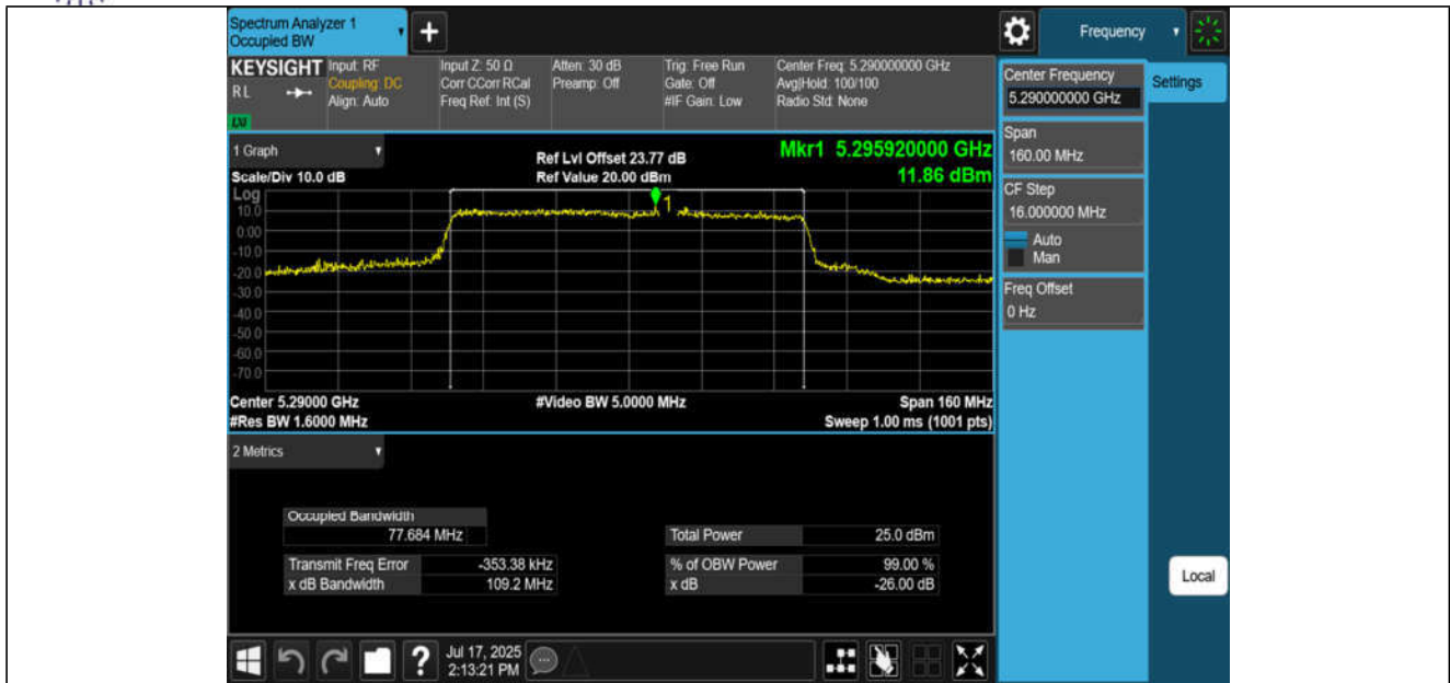
11BE80MIMO-Ant3-5290
