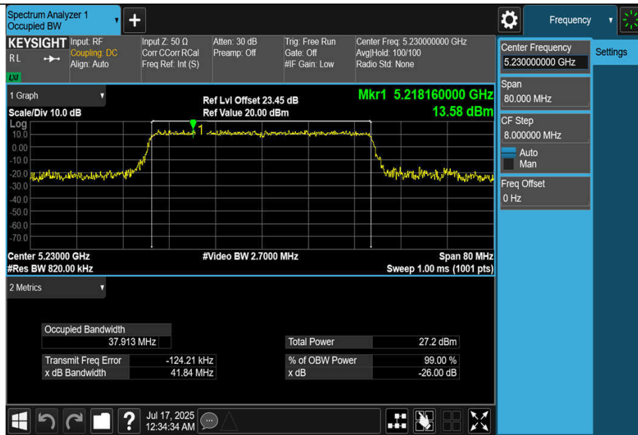
11BE40MIMO-Ant1-5230
