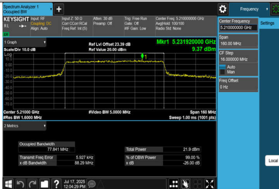
11BE80MIMO-Ant4-5210
