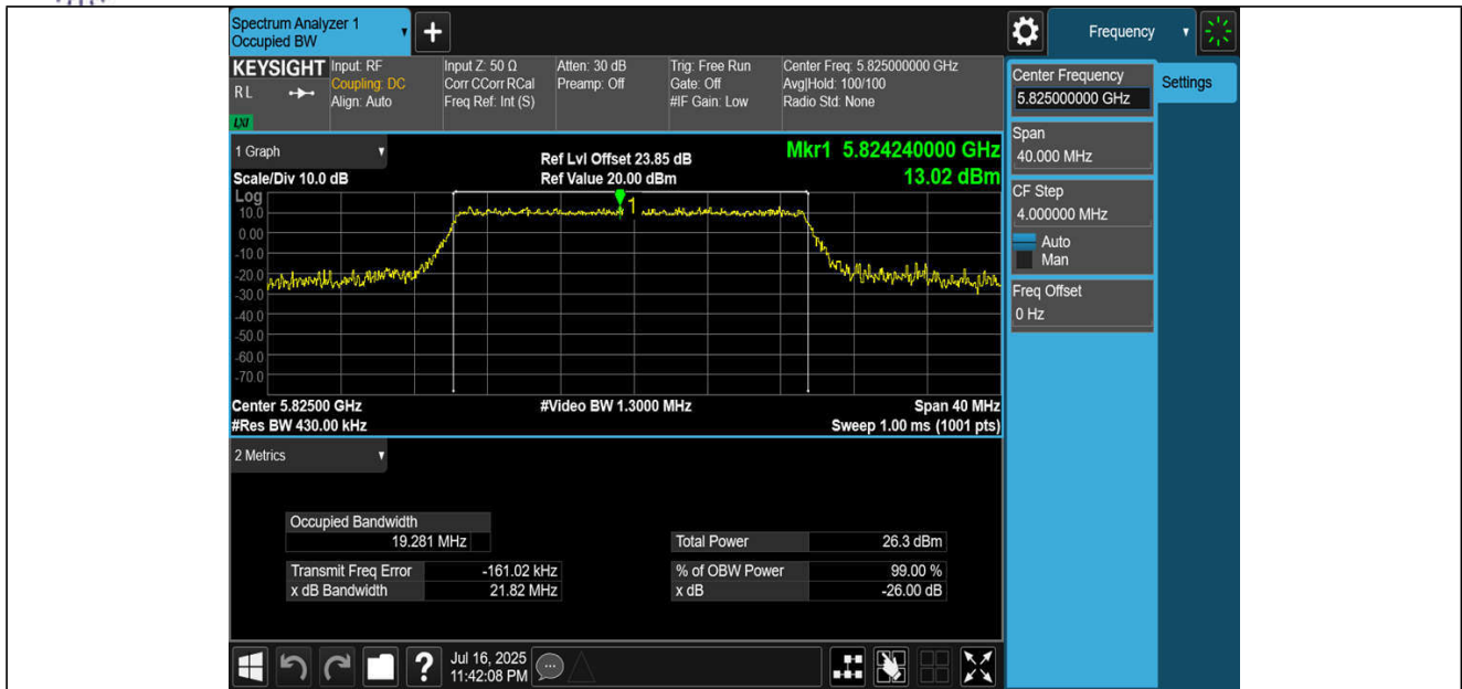
11BE20MIMO-Ant3-5825
