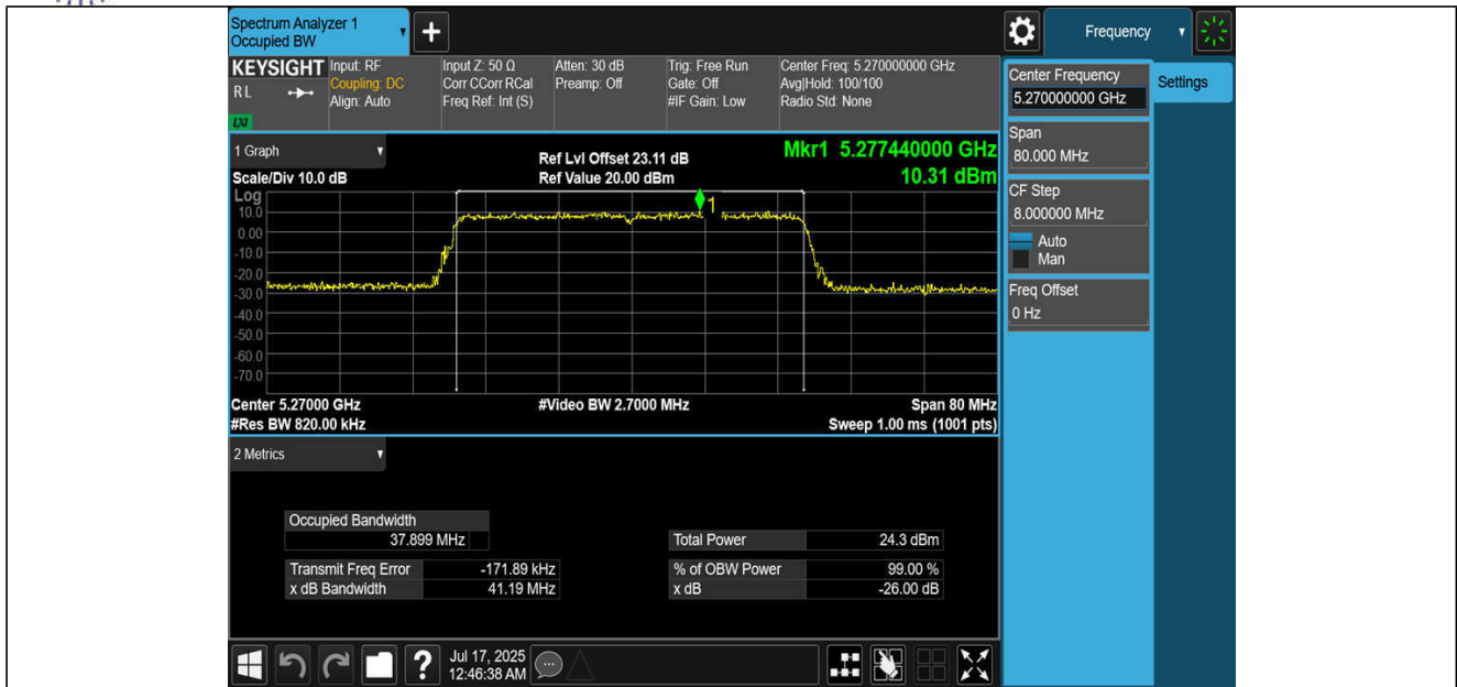
11BE40MIMO-Ant1-5270
