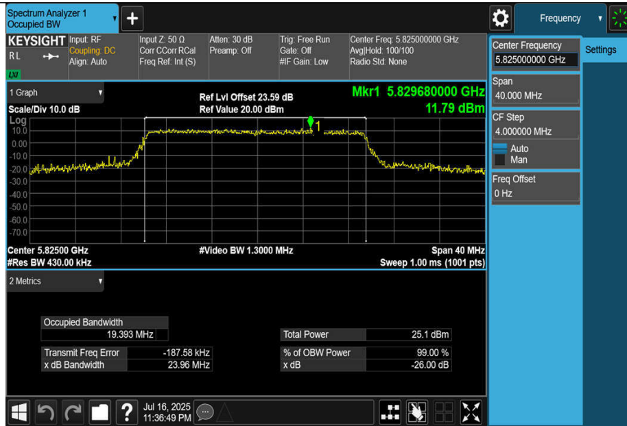
11BE20MIMO-Ant1-5825
