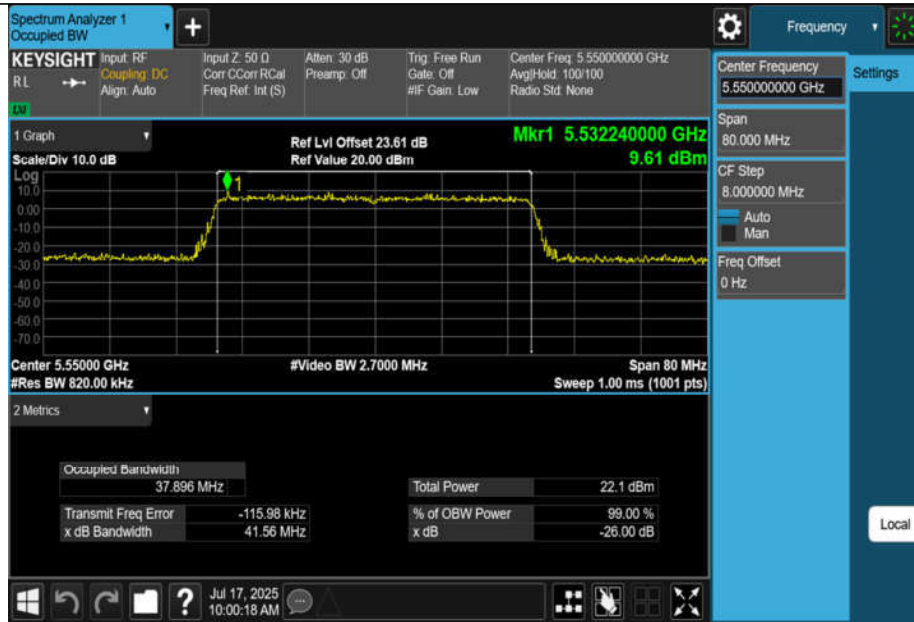
11BE40MIMO-Ant1-5550
