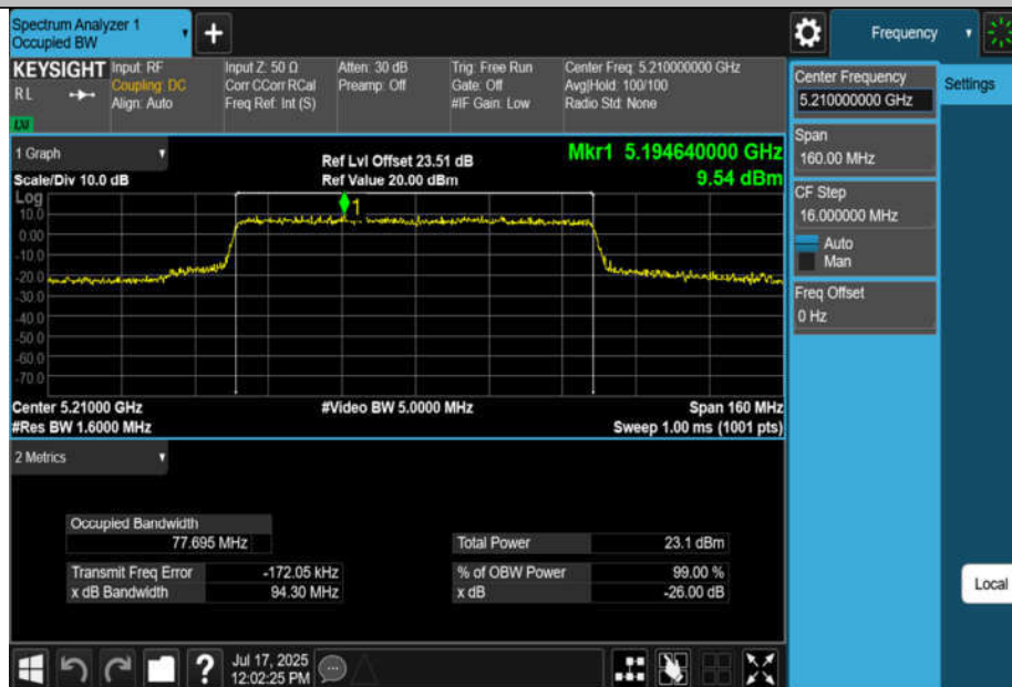
11BE80MIMO-Ant2-5210
