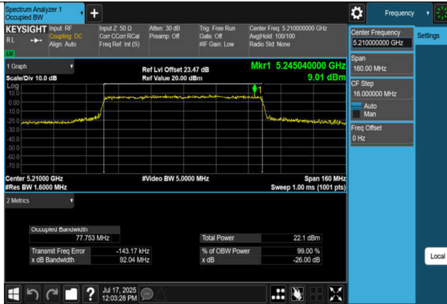
11BE80MIMO-Ant3-5210
