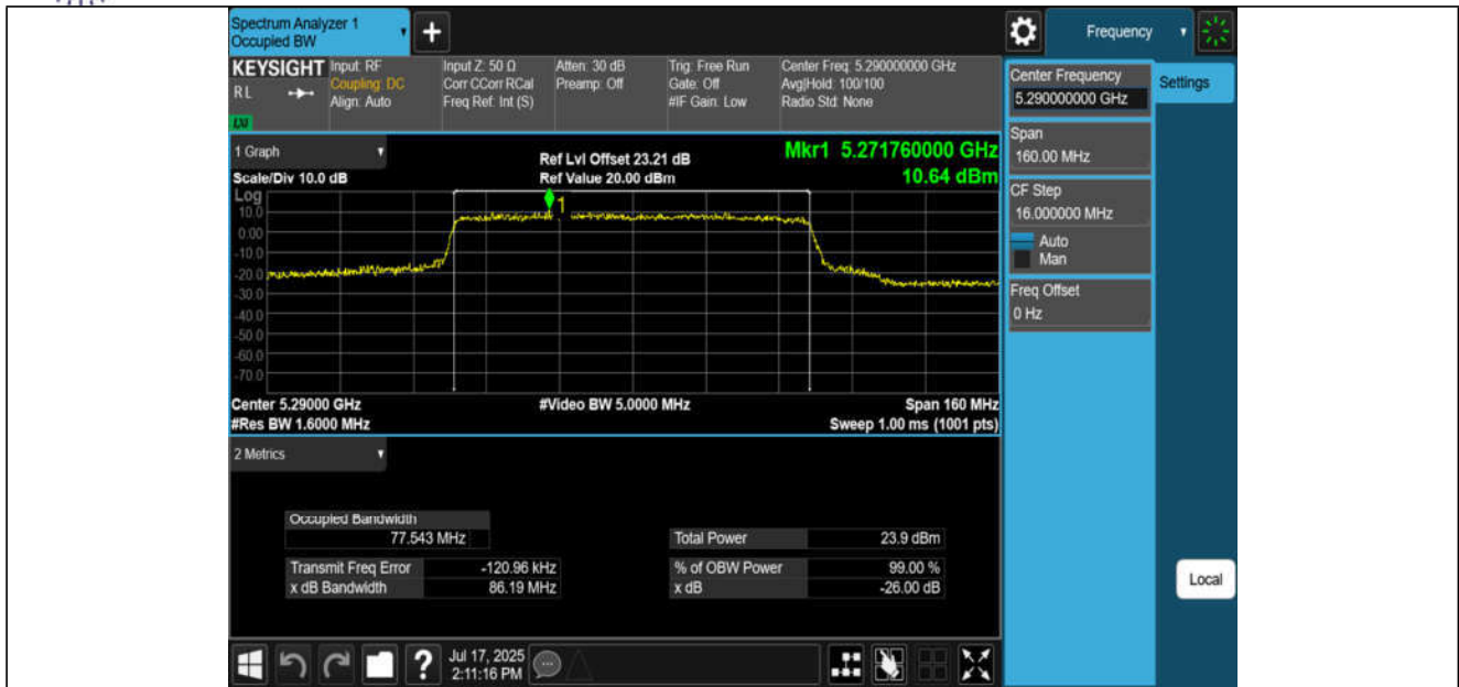
11BE80MIMO-Ant1-5290
