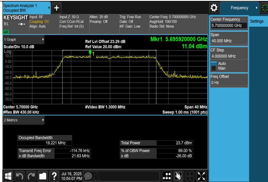
11BE20MIMO-Ant1-5700
