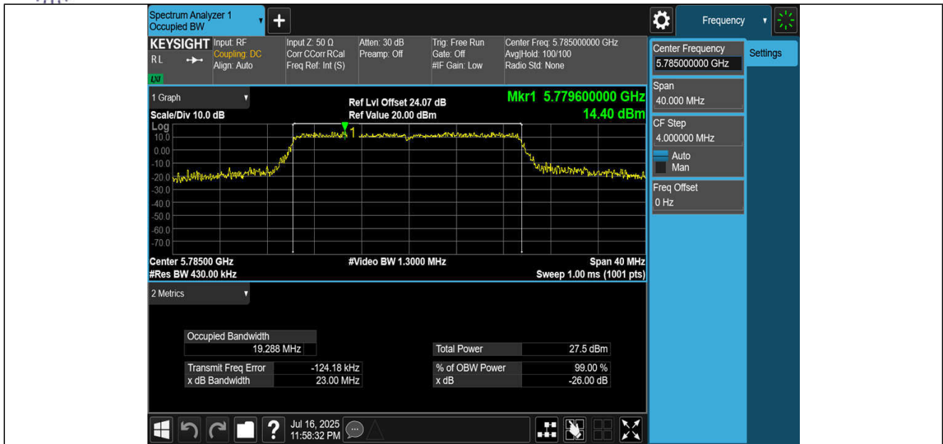
11BE20MIMO-Ant1-5785
