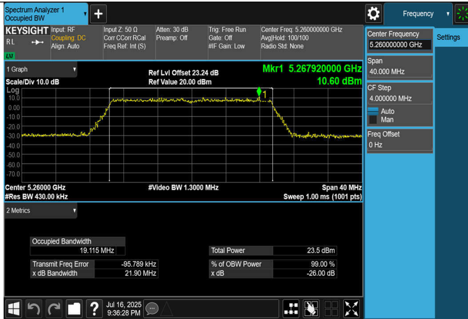
11BE20MIMO-Ant1-5260
