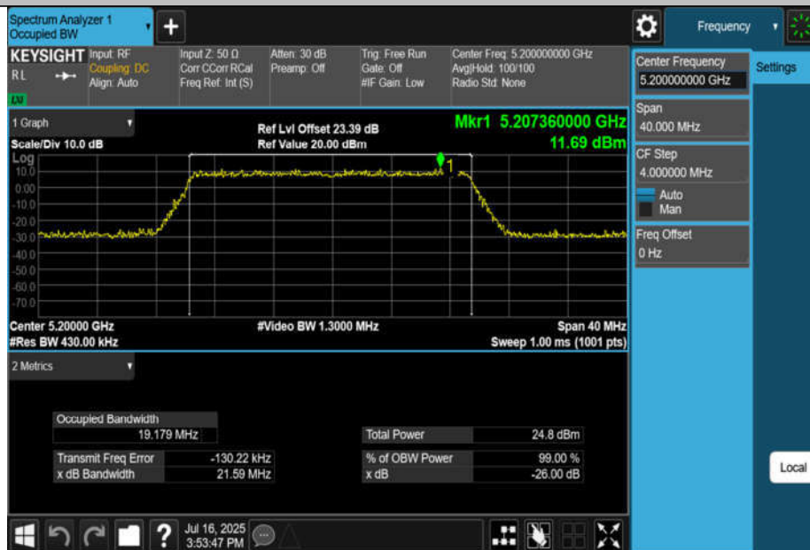
11BE20MIMO-Ant4-5200
