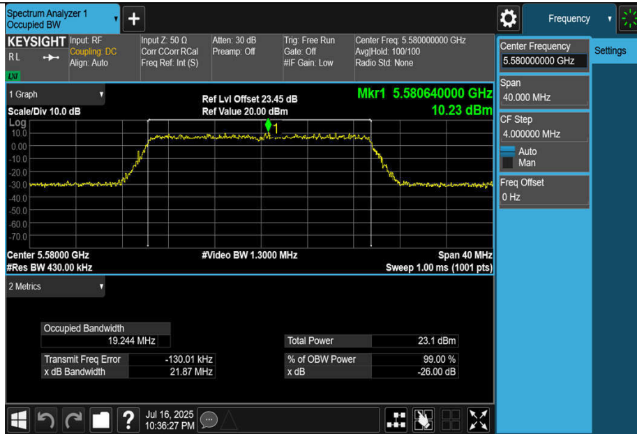
11BE20MIMO-Ant1-5580
