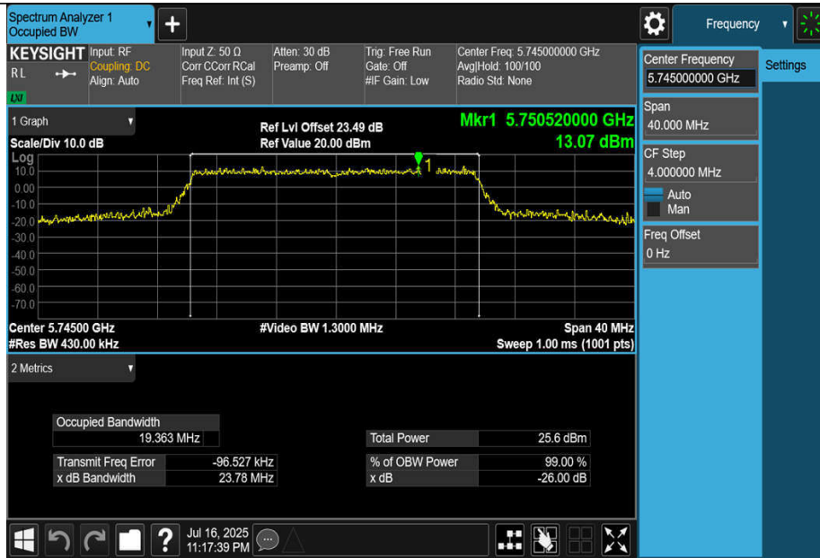
11BE20MIMO-Ant1-5745
