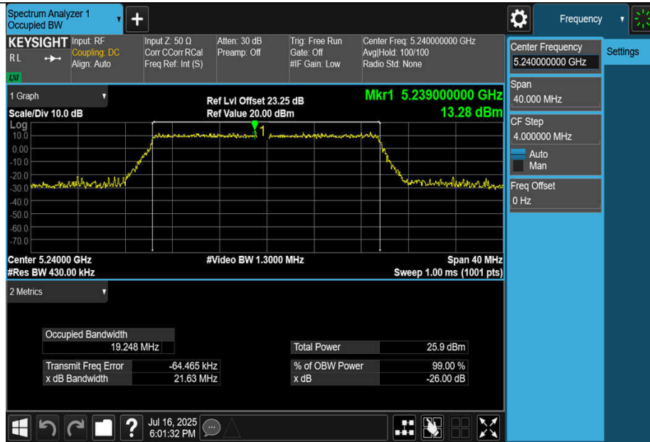
11BE20MIMO-Ant3-5240
