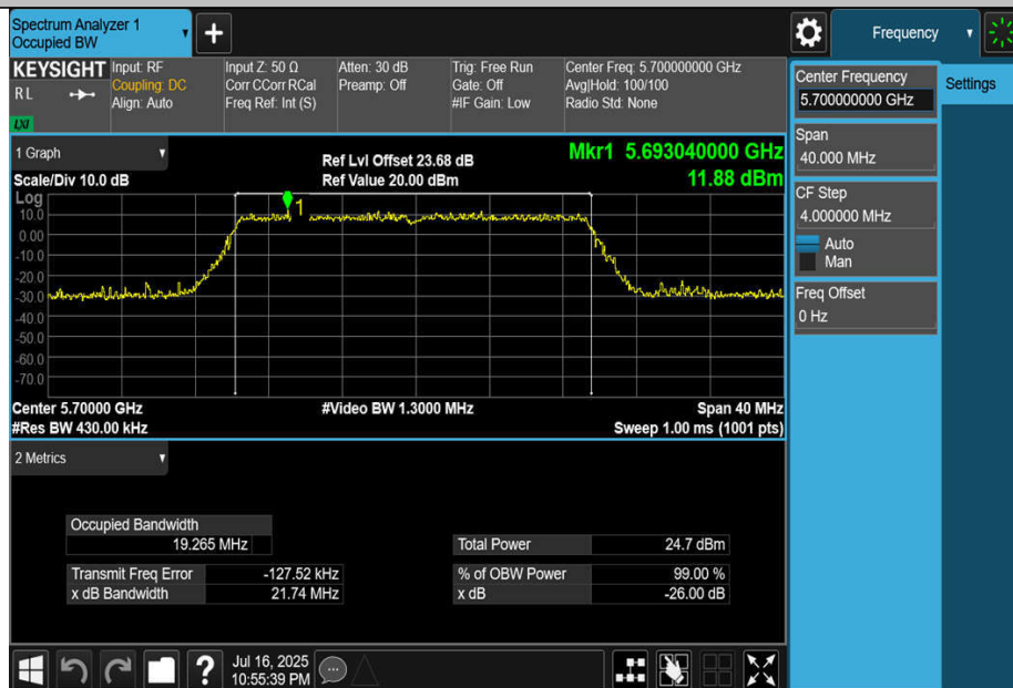
11BE20MIMO-Ant2-5700
