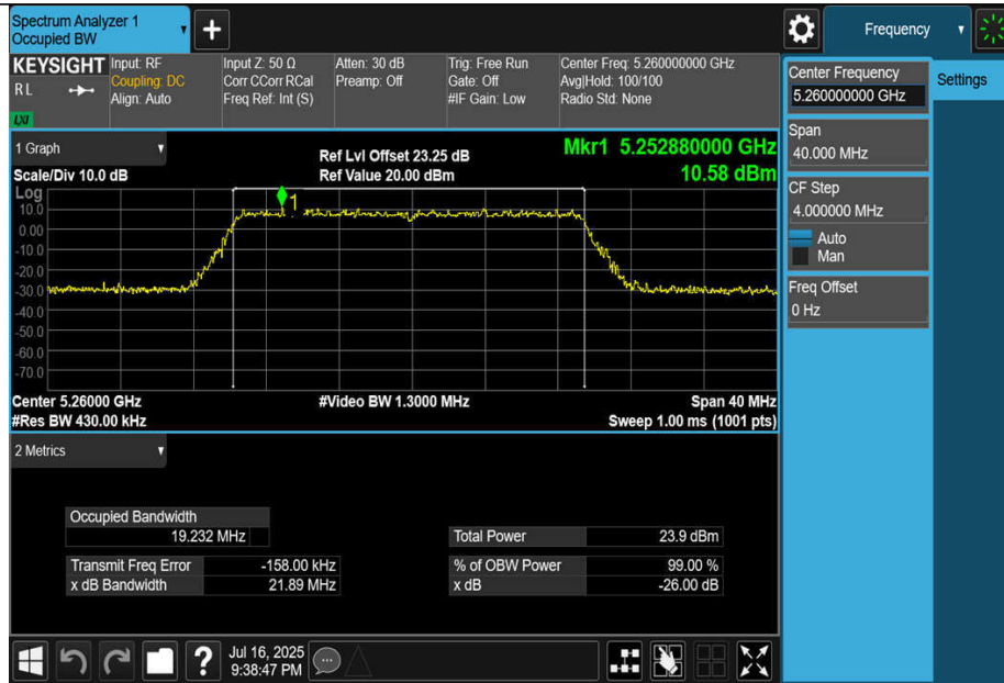
11BE20MIMO-Ant3-5260
