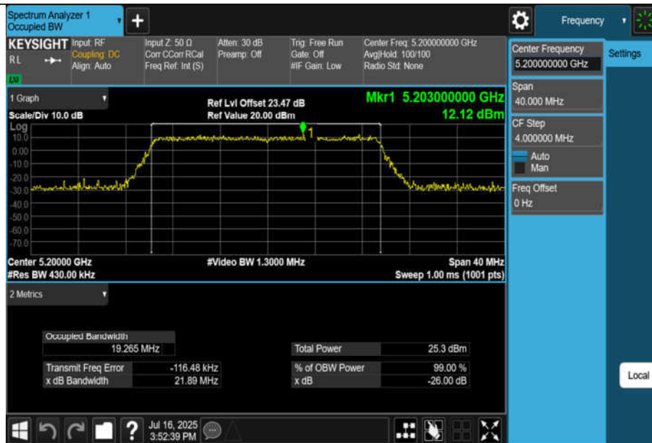
11BE20MIMO-Ant3-5200
