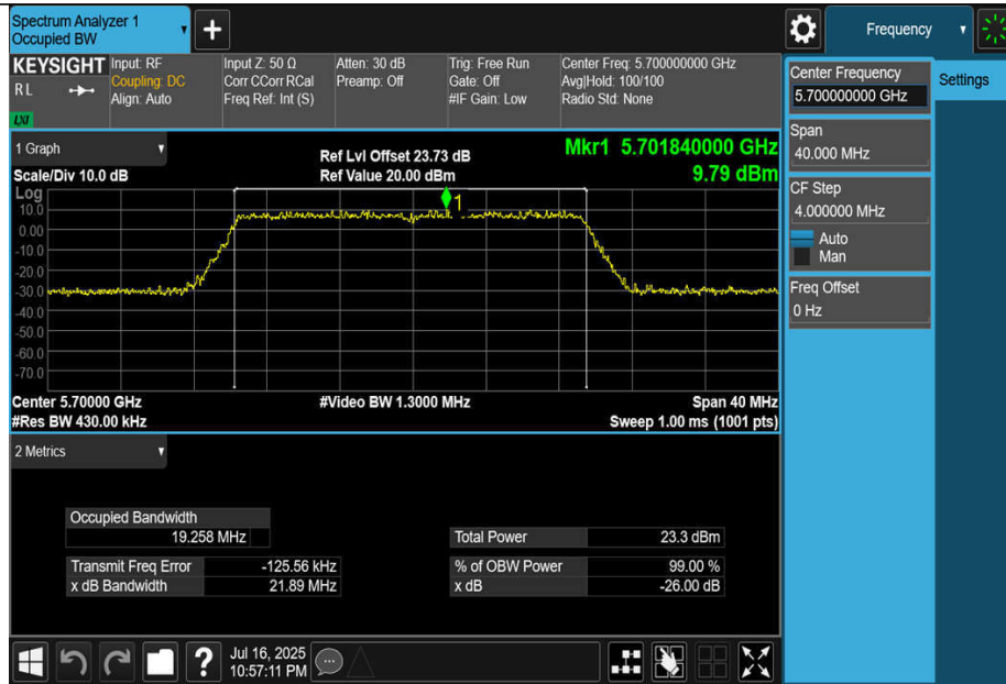
11BE20MIMO-Ant3-5700
