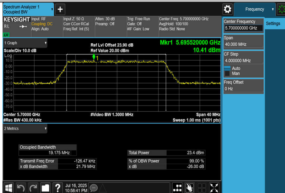
11BE20MIMO-Ant4-5700
