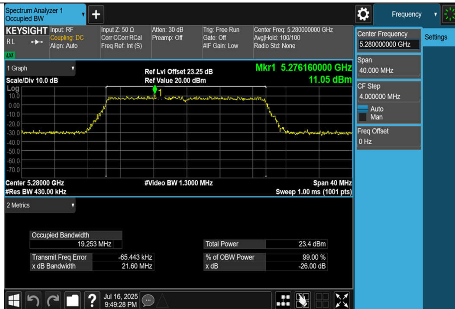
11BE20MIMO-Ant3-5280
