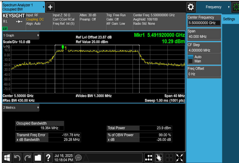
11BE20MIMO-Ant1-5500
