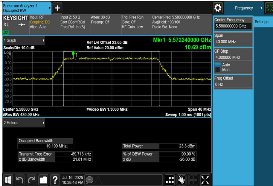
11BE20MIMO-Ant3-5580
