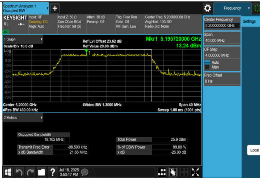
11BE20MIMO-Ant1-5200
