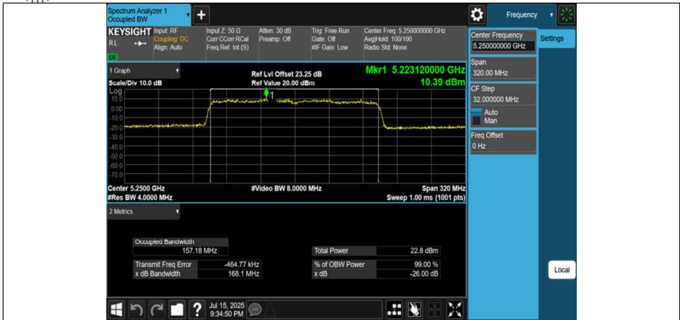
11AX160MIMO-Ant3-5250
