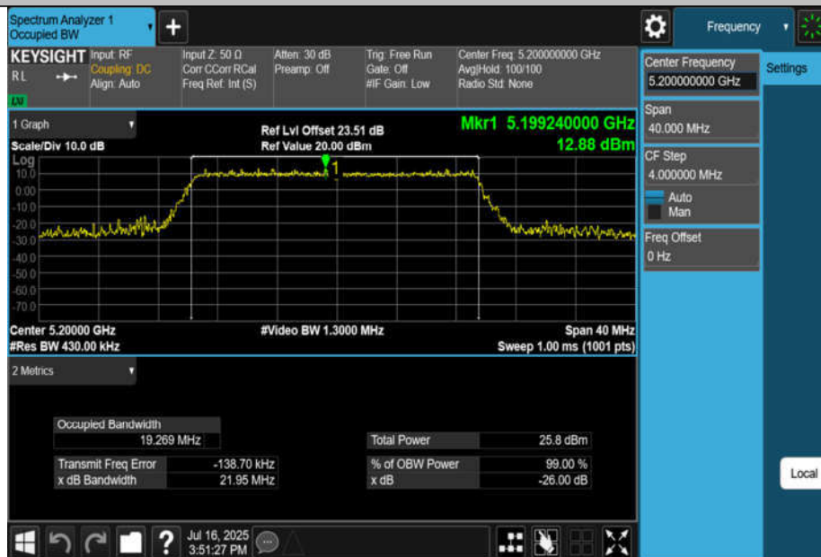
11BE20MIMO-Ant2-5200
