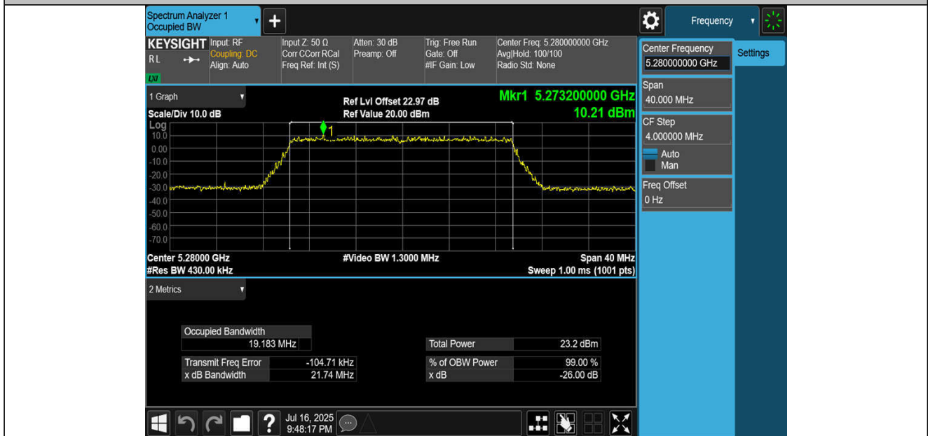
11BE20MIMO-Ant2-5280
