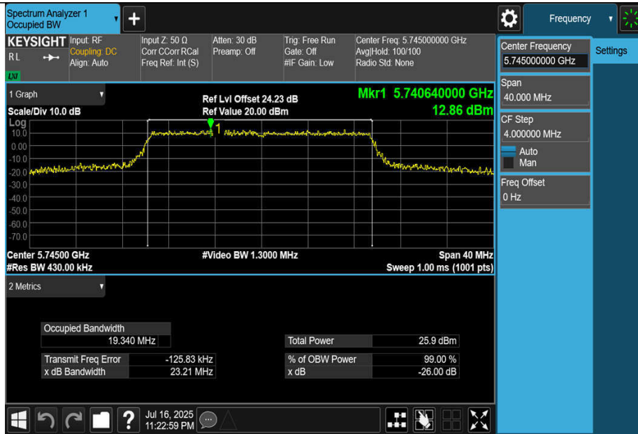
11BE20MIMO-Ant3-5745
