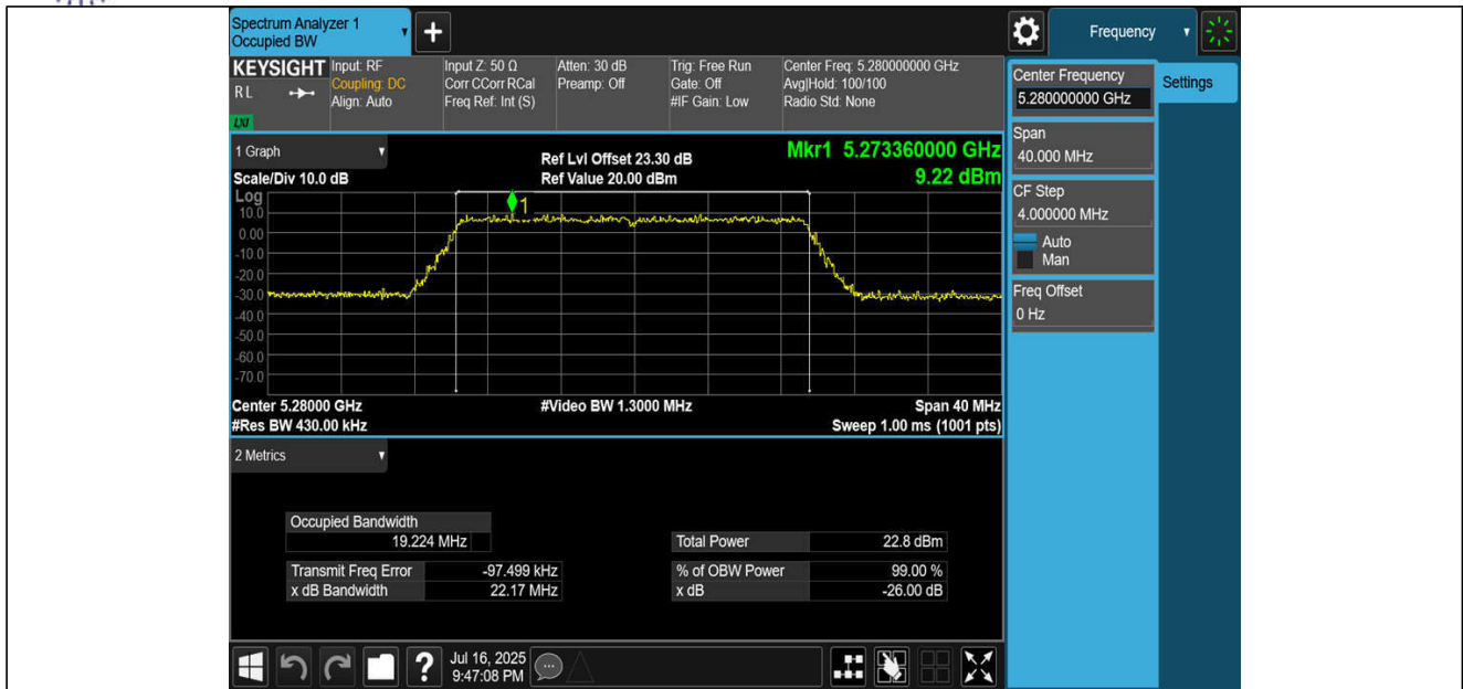
11BE20MIMO-Ant1-5280
