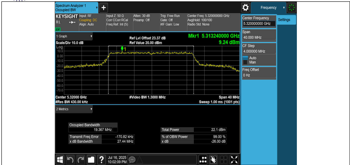
11BE20MIMO-Ant1-5320
