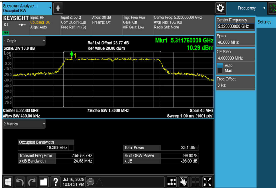
11BE20MIMO-Ant3-5320
