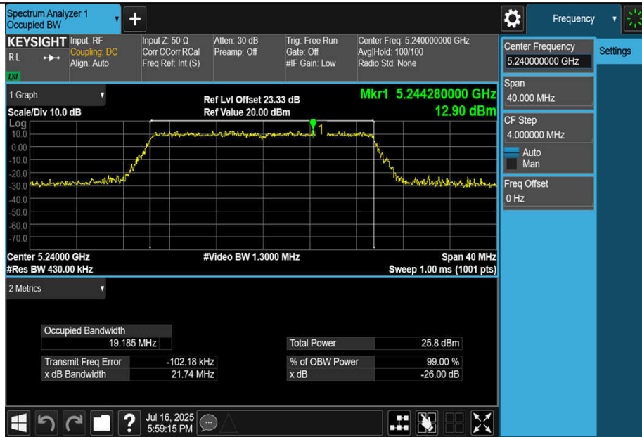
11BE20MIMO-Ant1-5240
