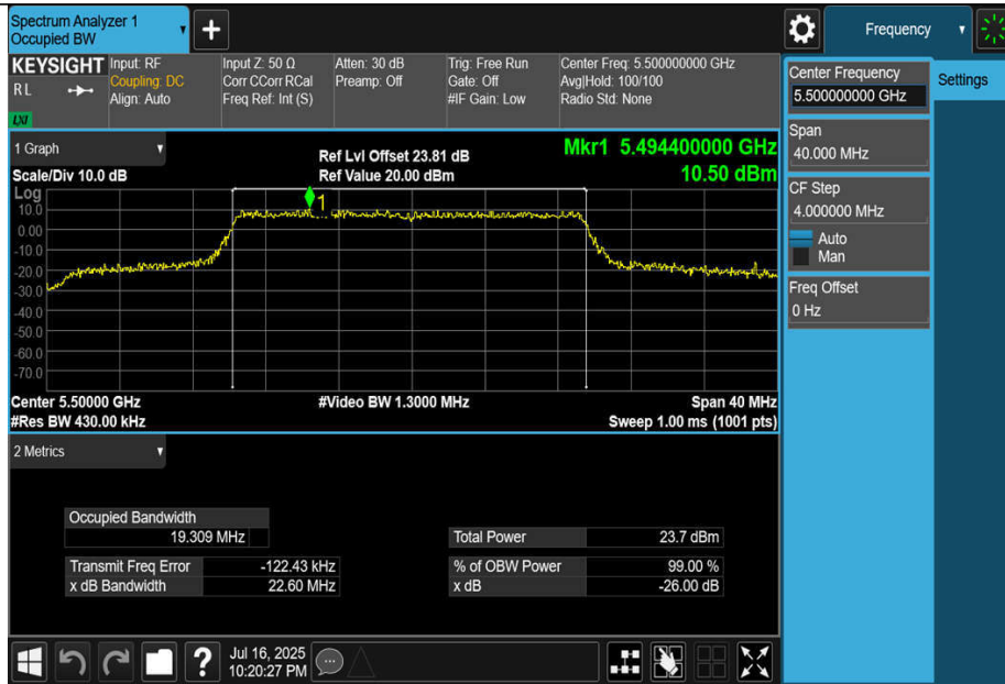
11BE20MIMO-Ant3-5500
