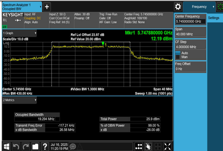
11BE20MIMO-Ant2-5745
