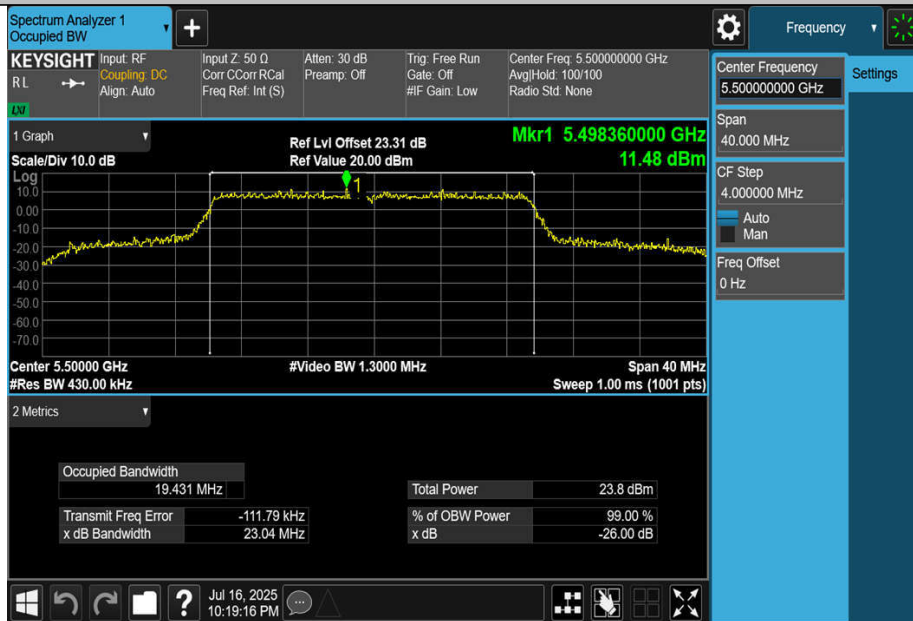
11BE20MIMO-Ant2-5500
