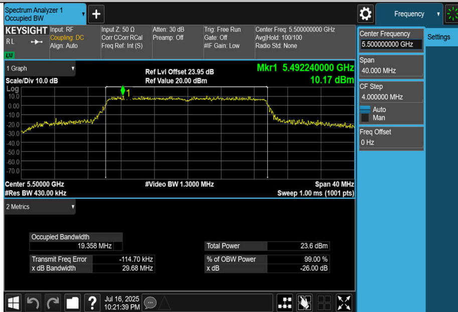
11BE20MIMO-Ant4-5500
