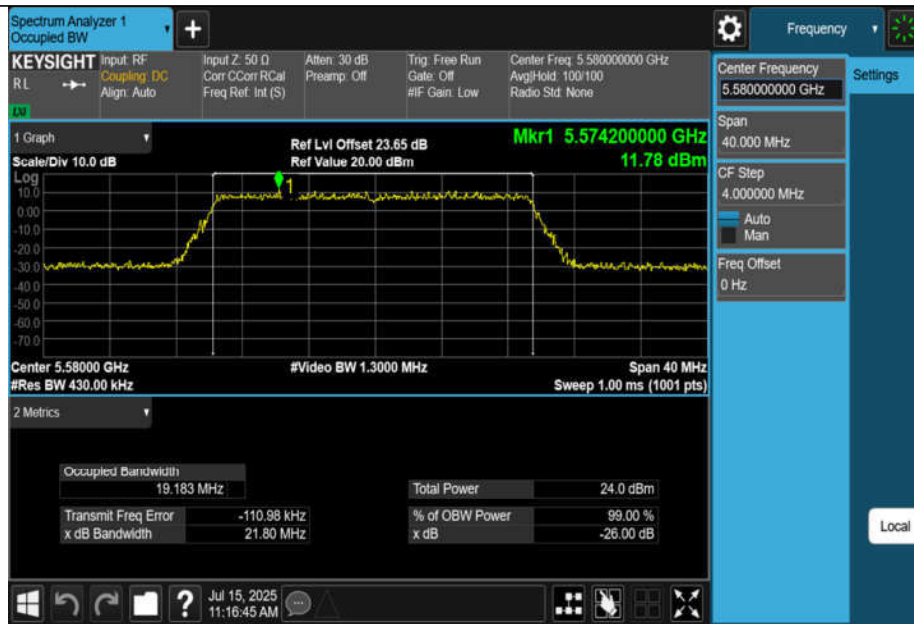
11AX20MIMO-Ant3-5580
