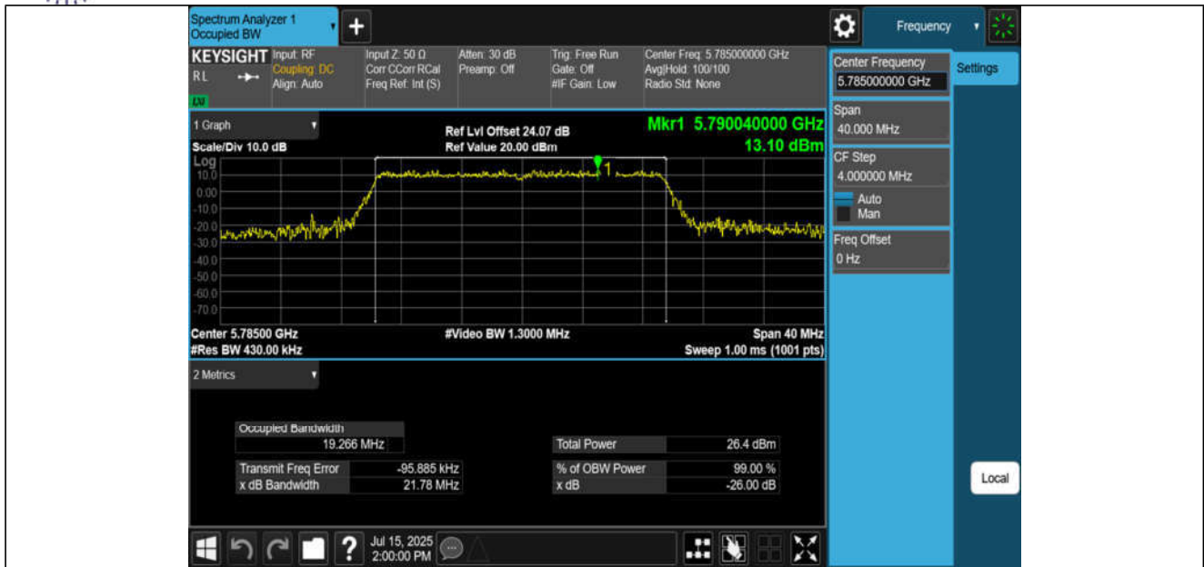
11AX20MIMO-Ant1-5785
