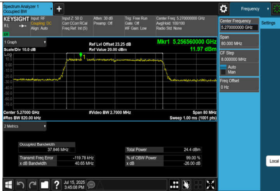
11AX40MIMO-Ant3-5270
