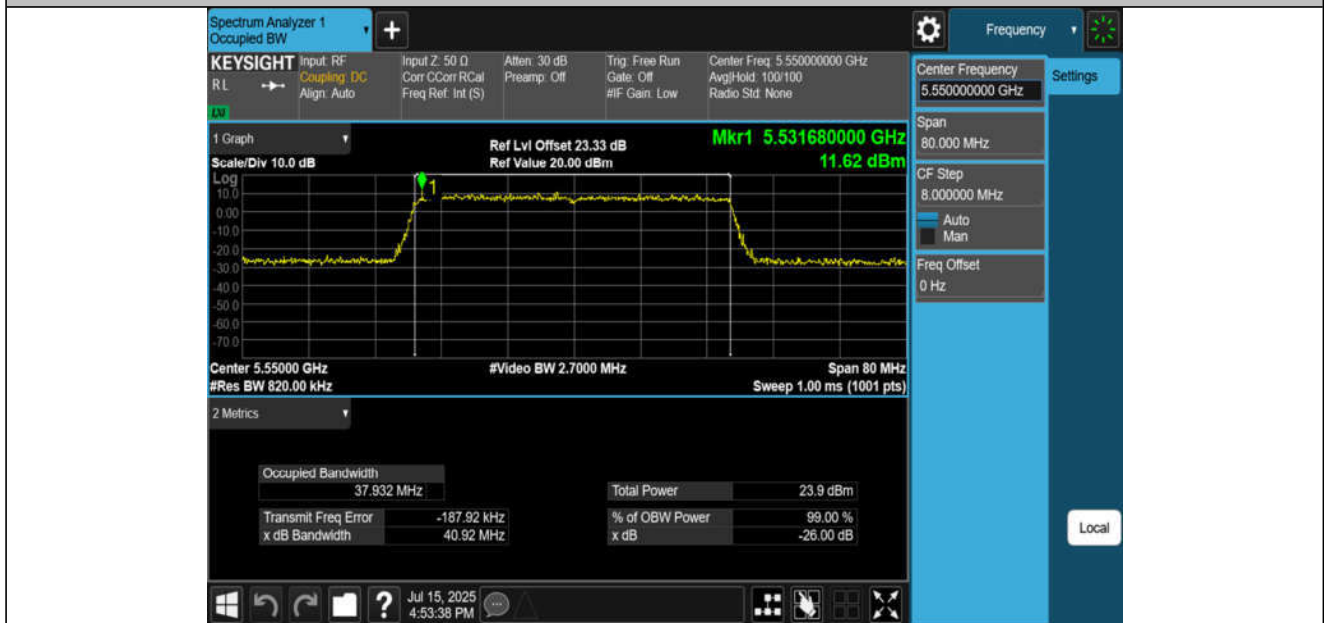
11AX40MIMO-Ant2-5550
