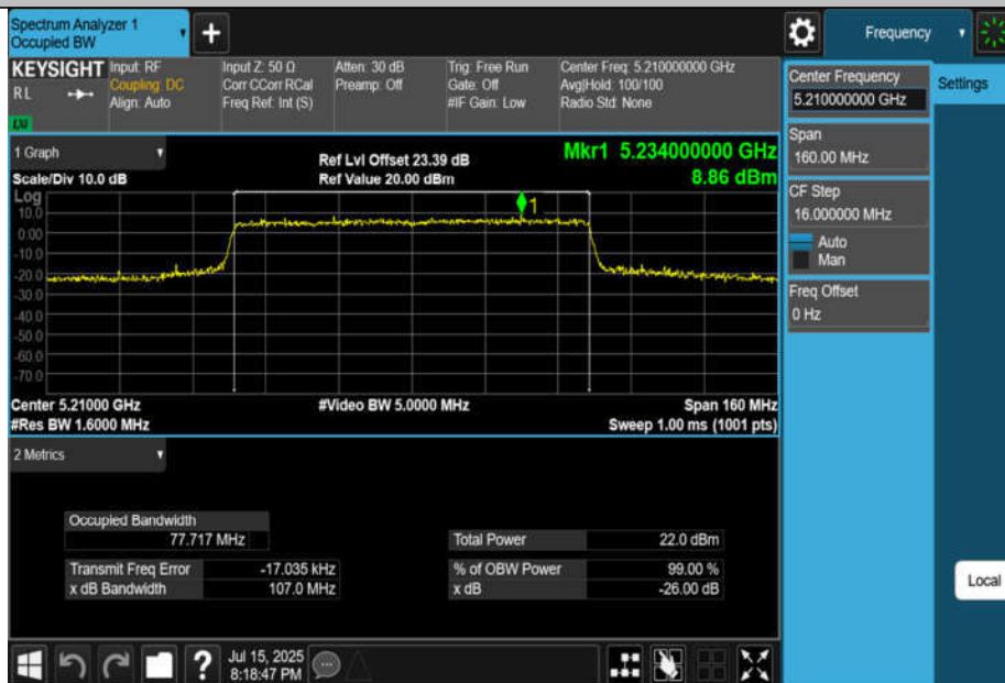
11AX80MIMO-Ant4-5210
