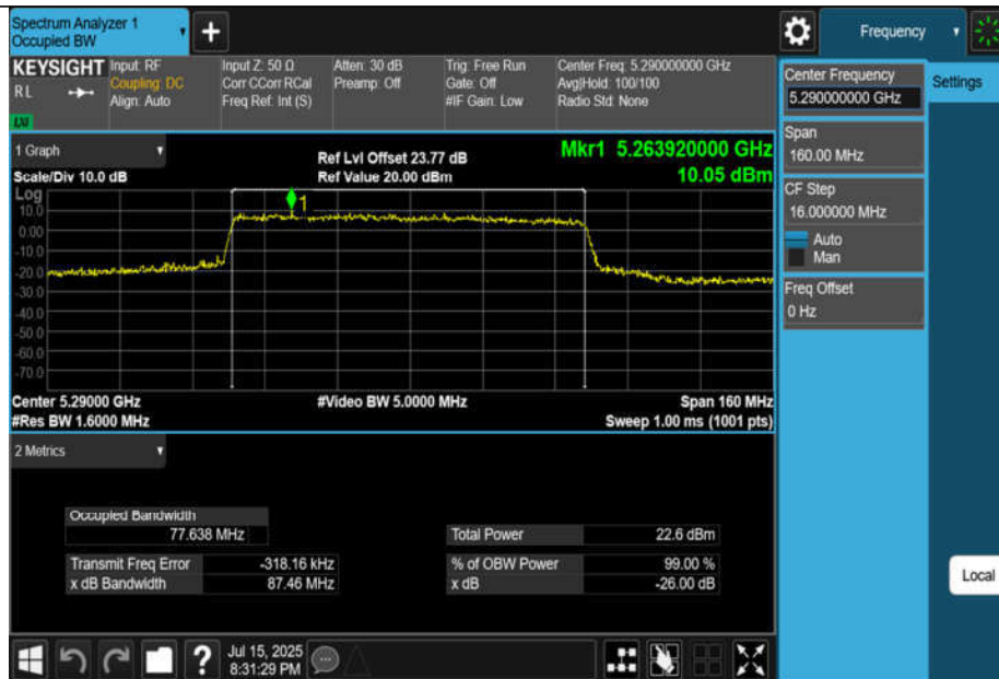
11AX80MIMO-Ant3-5290
