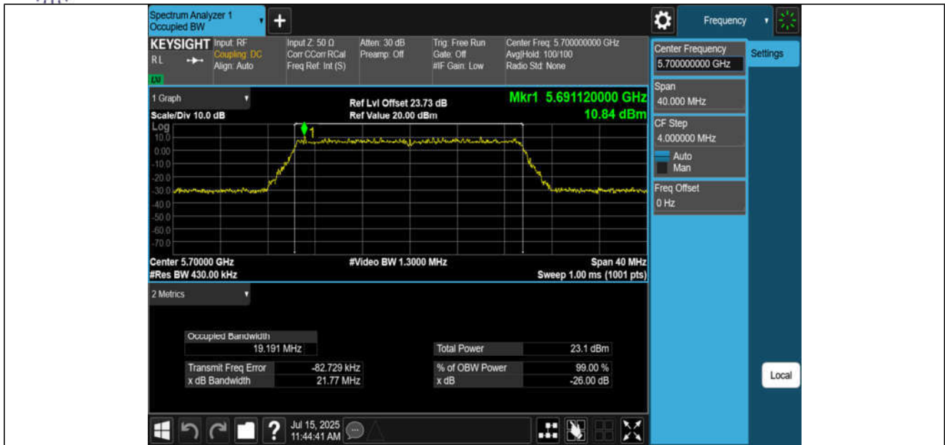
11AX20MIMO-Ant3-5700
