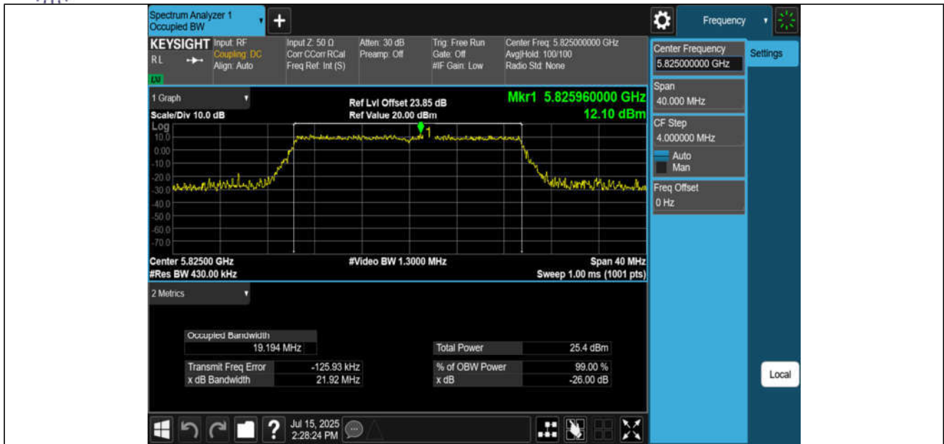
11AX20MIMO-Ant3-5825
