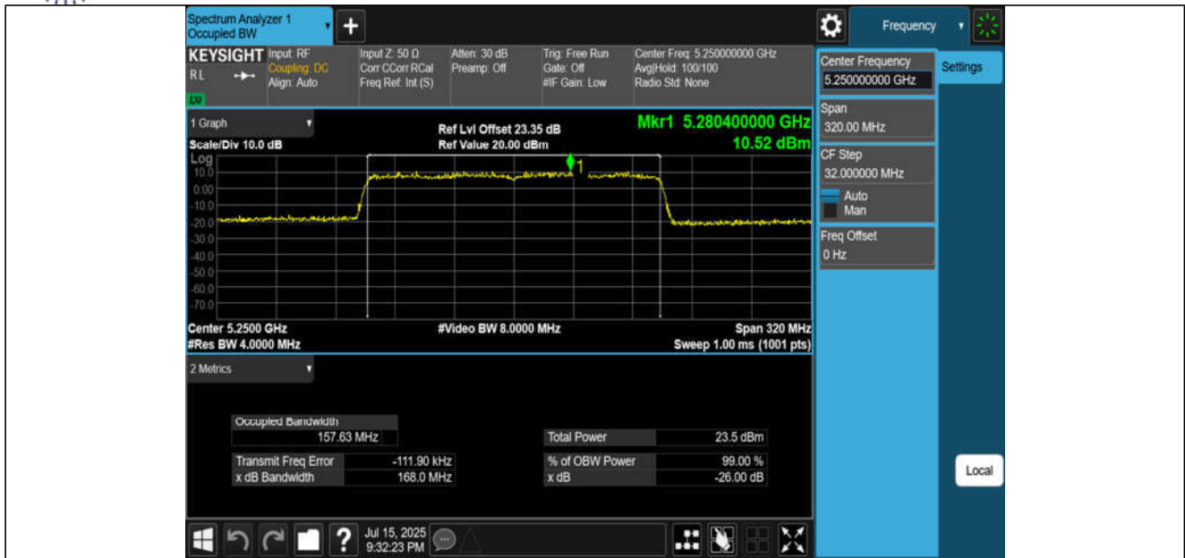
11AX160MIMO-Ant1-5250
