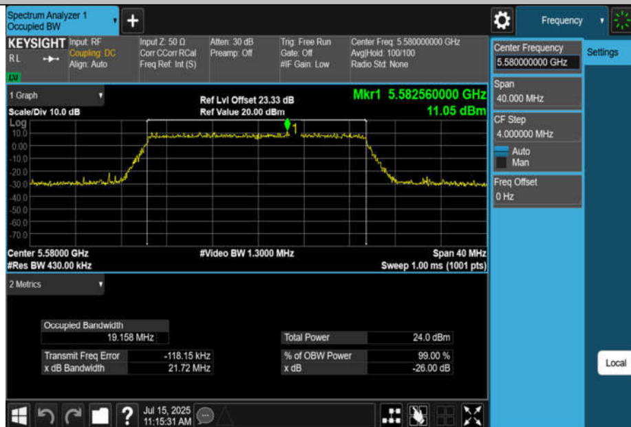
11AX20MIMO-Ant2-5580
