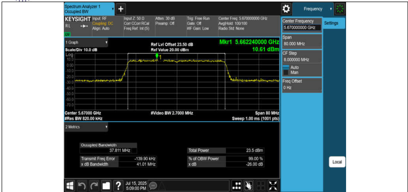
11AX40MIMO-Ant1-5670
