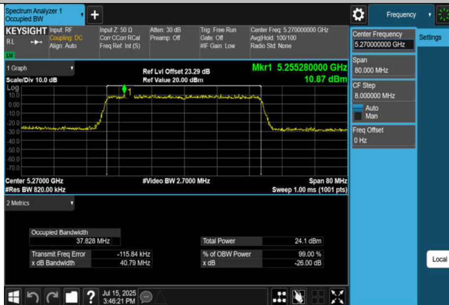
11AX40MIMO-Ant4-5270
