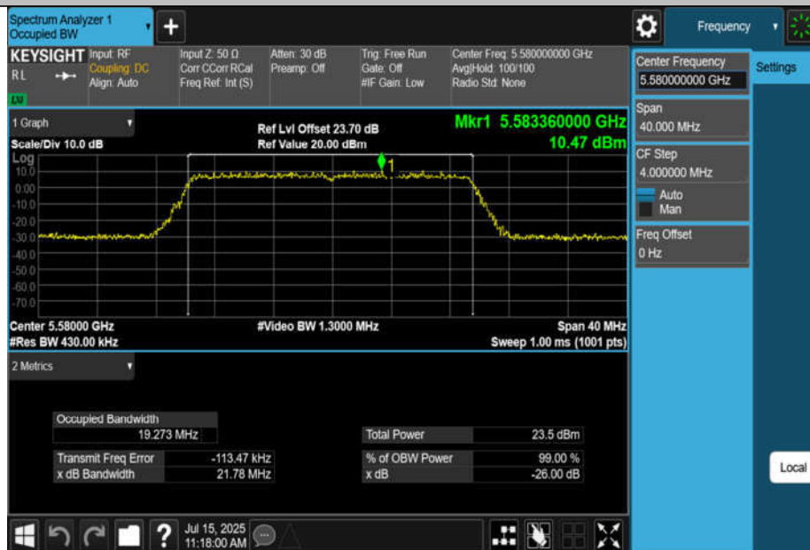
11AX20MIMO-Ant4-5580
