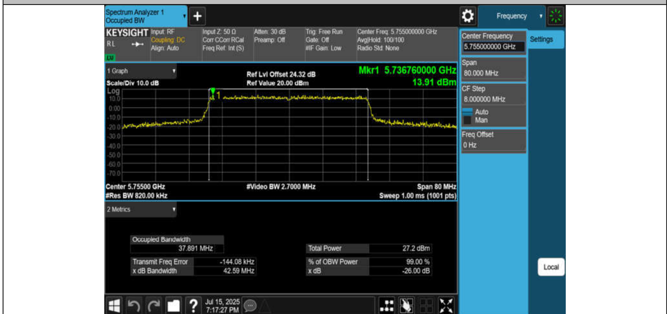
11AX40MIMO-Ant4-5755
