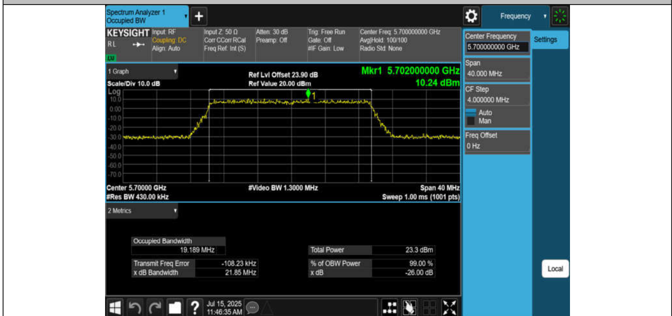
11AX20MIMO-Ant4-5700
