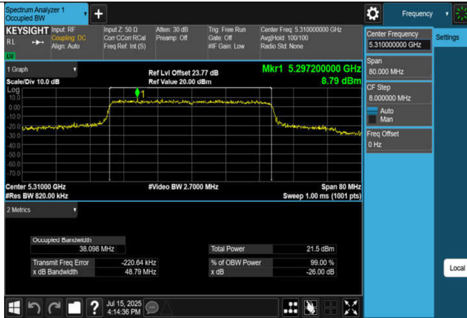
11AX40MIMO-Ant3-5310
