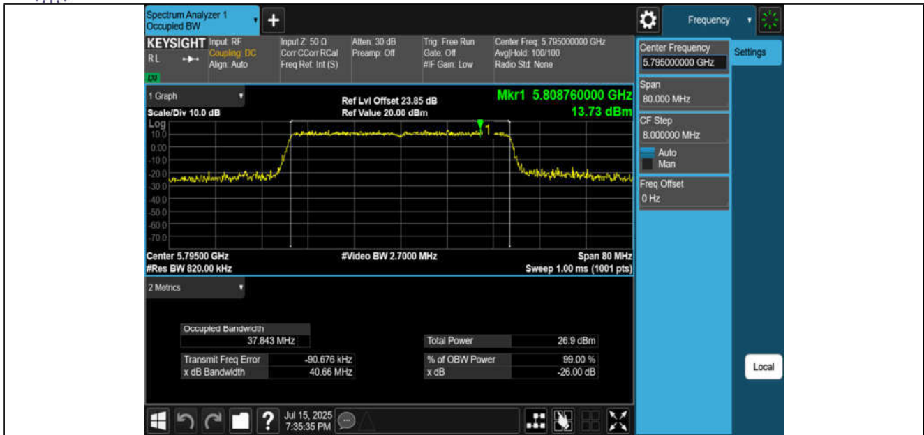
11AX40MIMO-Ant3-5795
