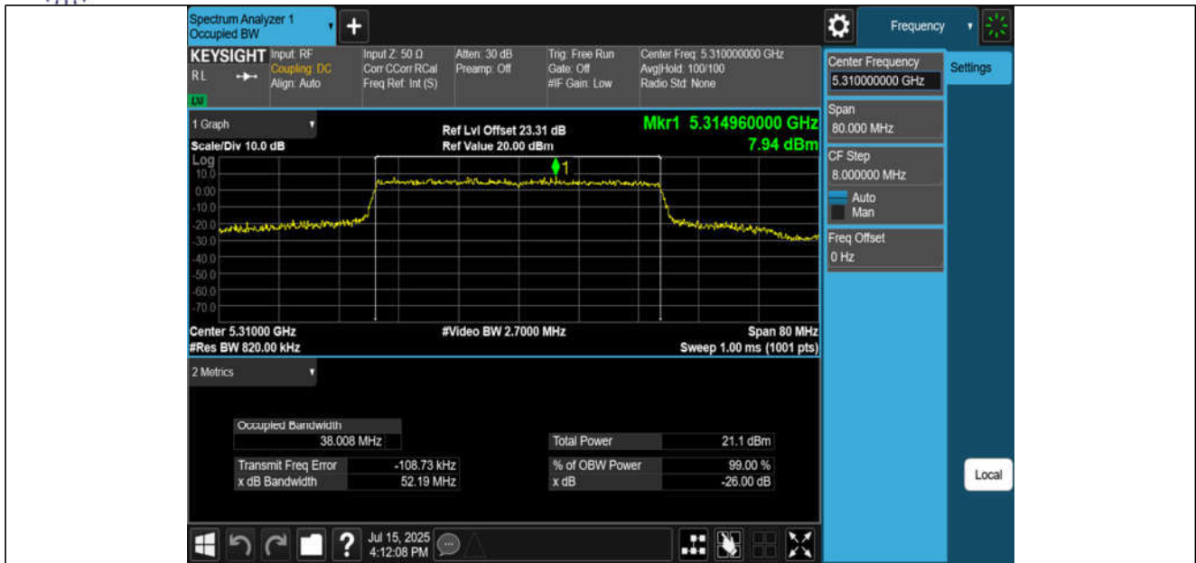
11AX40MIMO-Ant1-5310
