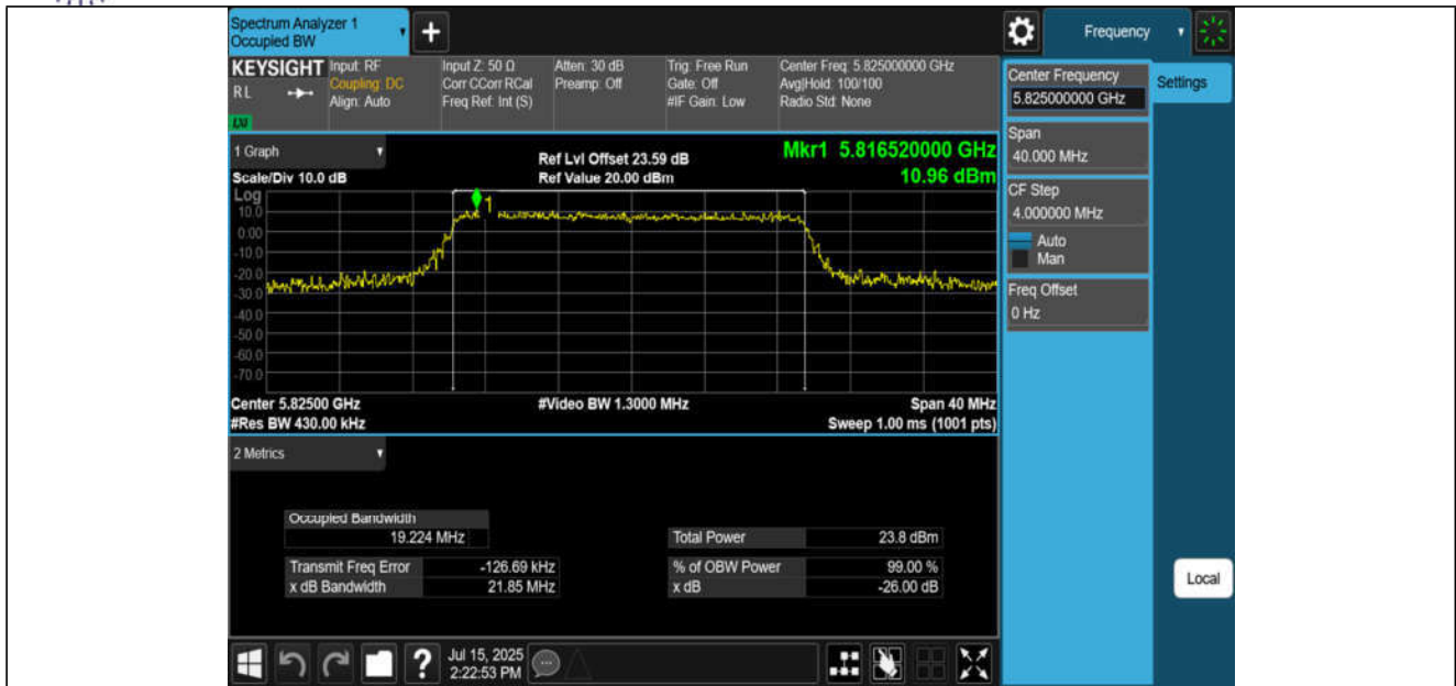
11AX20MIMO-Ant1-5825
