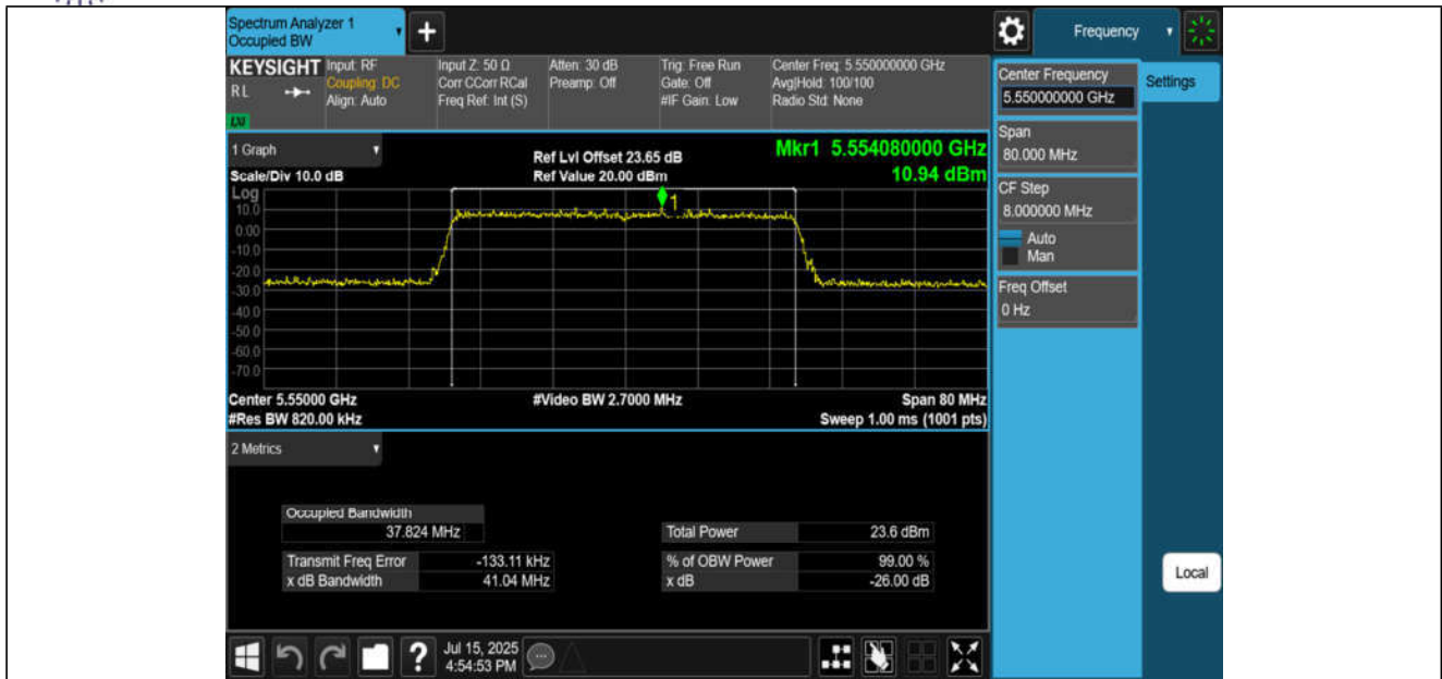
11AX40MIMO-Ant3-5550
