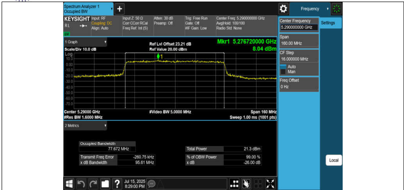
11AX80MIMO-Ant1-5290
