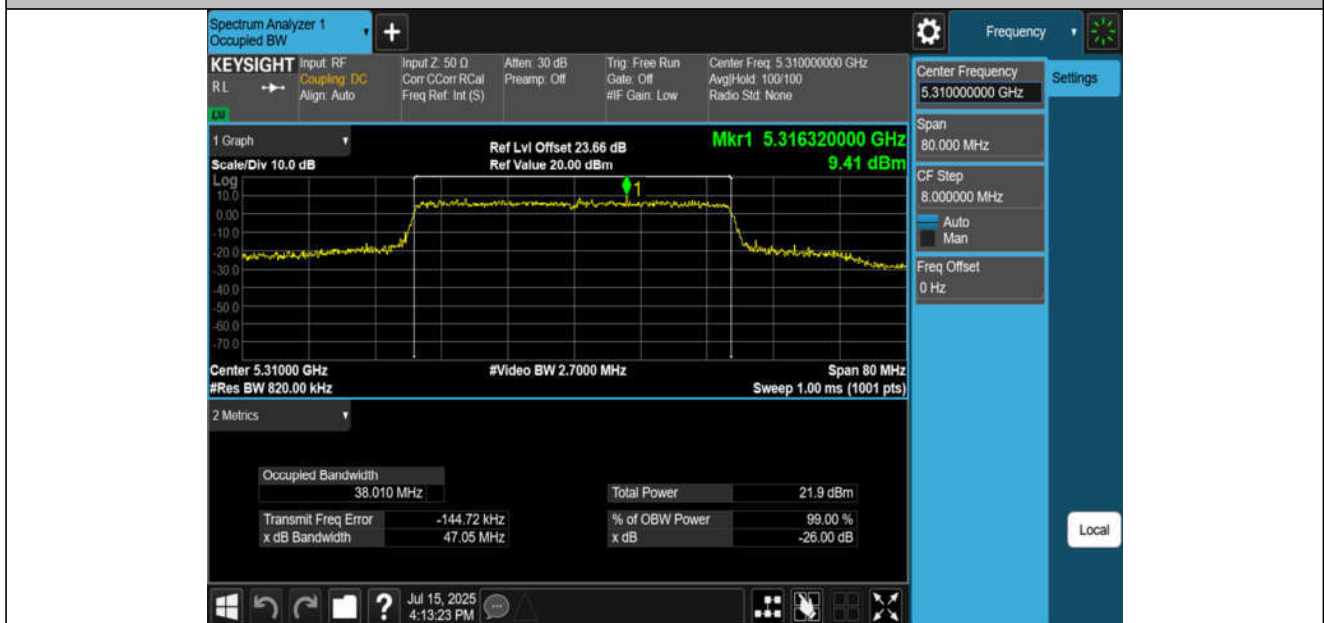
11AX40MIMO-Ant2-5310
