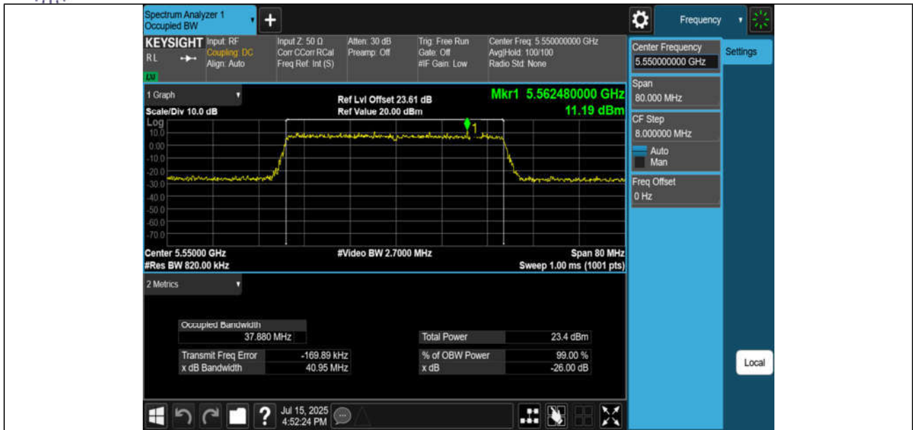
11AX40MIMO-Ant1-5550
