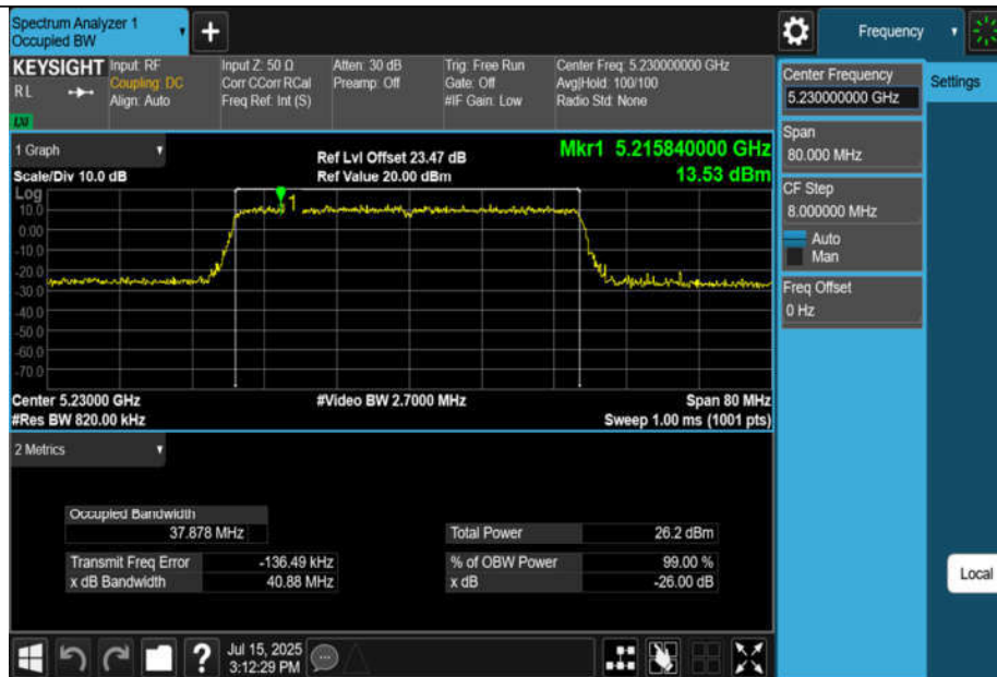
11AX40MIMO-Ant3-5230
