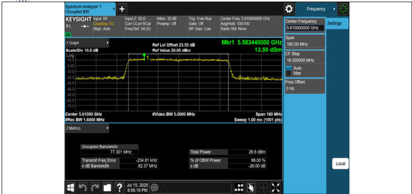
11AX80MIMO-Ant1-5610
