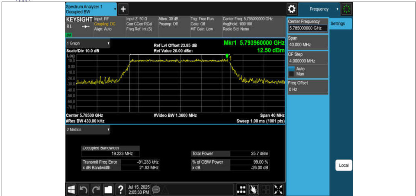
11AX20MIMO-Ant3-5785
