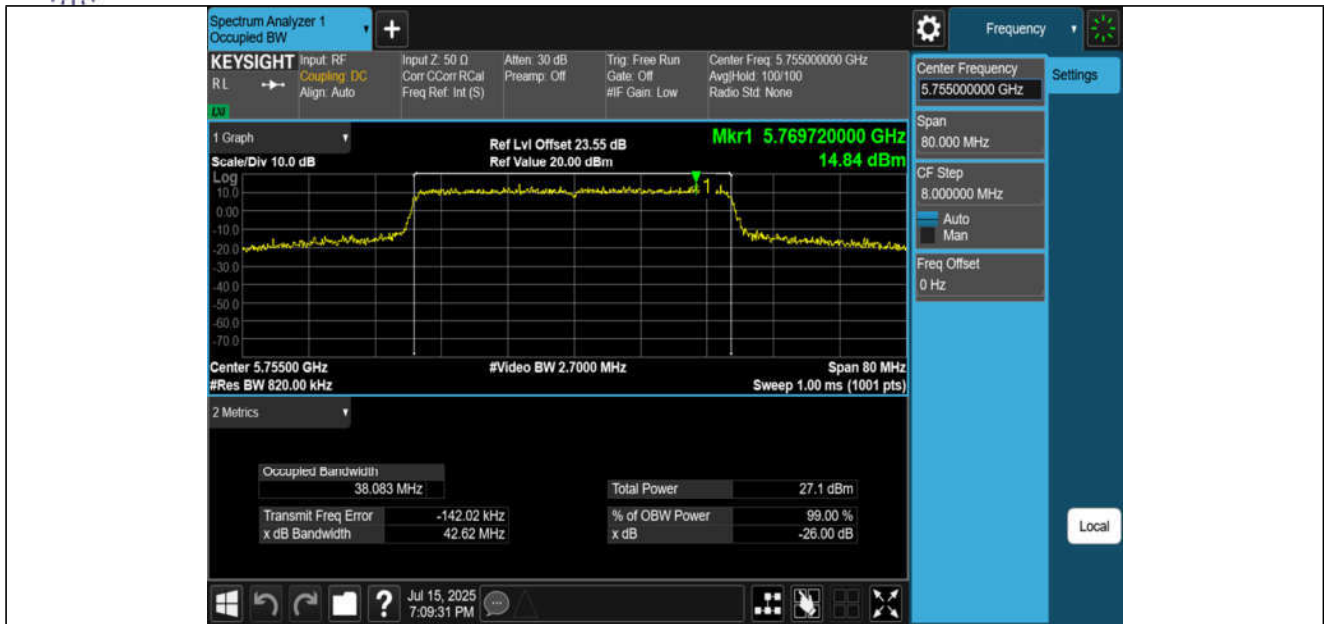
11AX40MIMO-Ant1-5755
