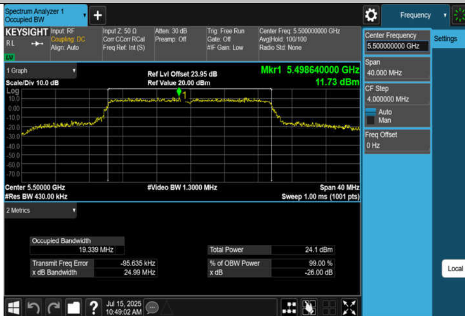
11AX20MIMO-Ant4-5500
