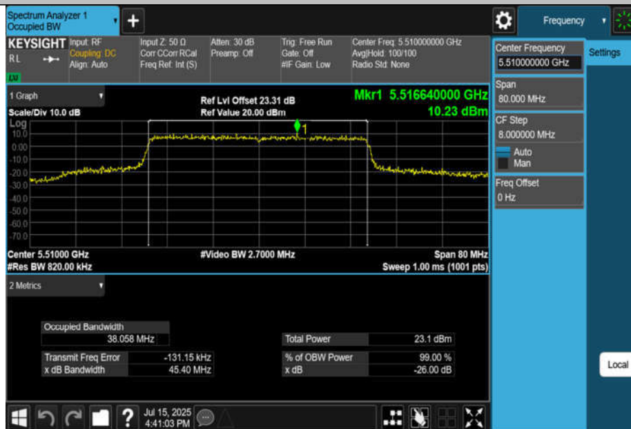
11AX40MIMO-Ant2-5510
