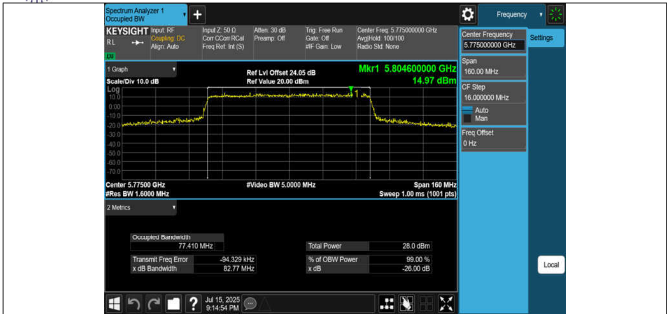
11AX80MIMO-Ant1-5775
