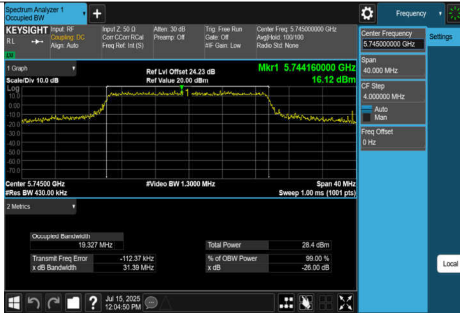
11AX20MIMO-Ant3-5745
