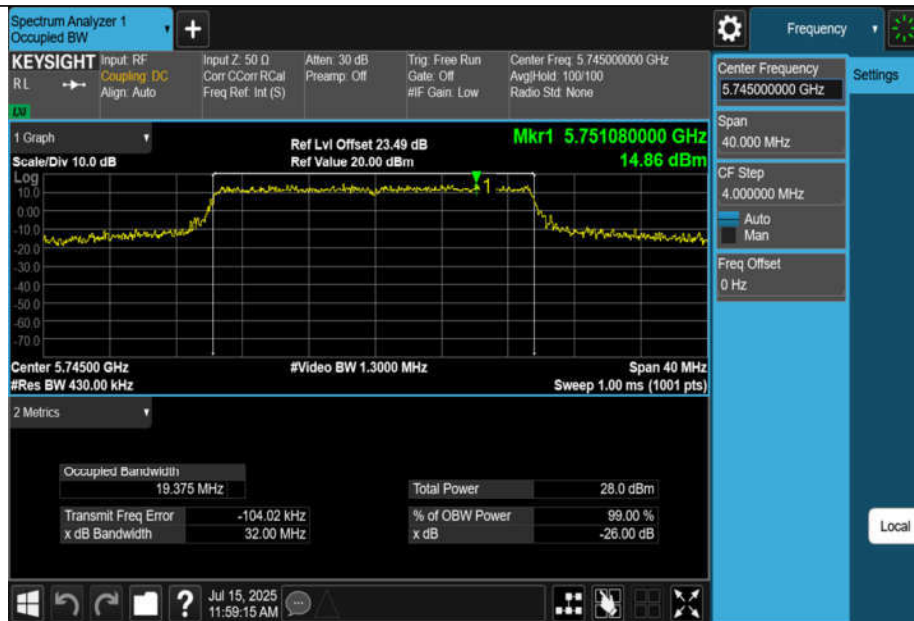
11AX20MIMO-Ant1-5745
