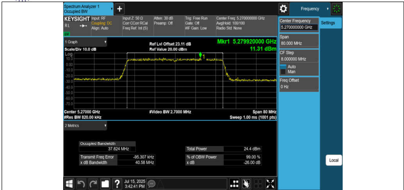
11AX40MIMO-Ant1-5270
