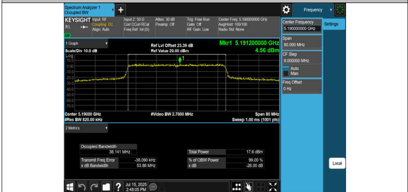
11AX40MIMO-Ant4-5190
