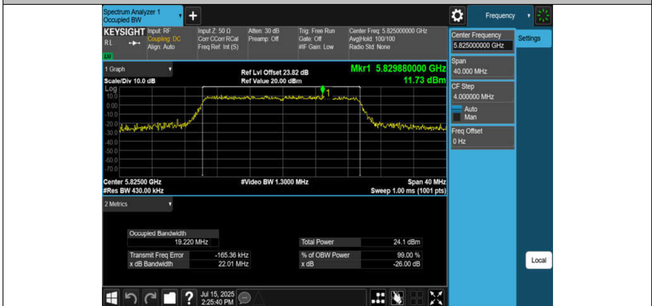
11AX20MIMO-Ant2-5825
