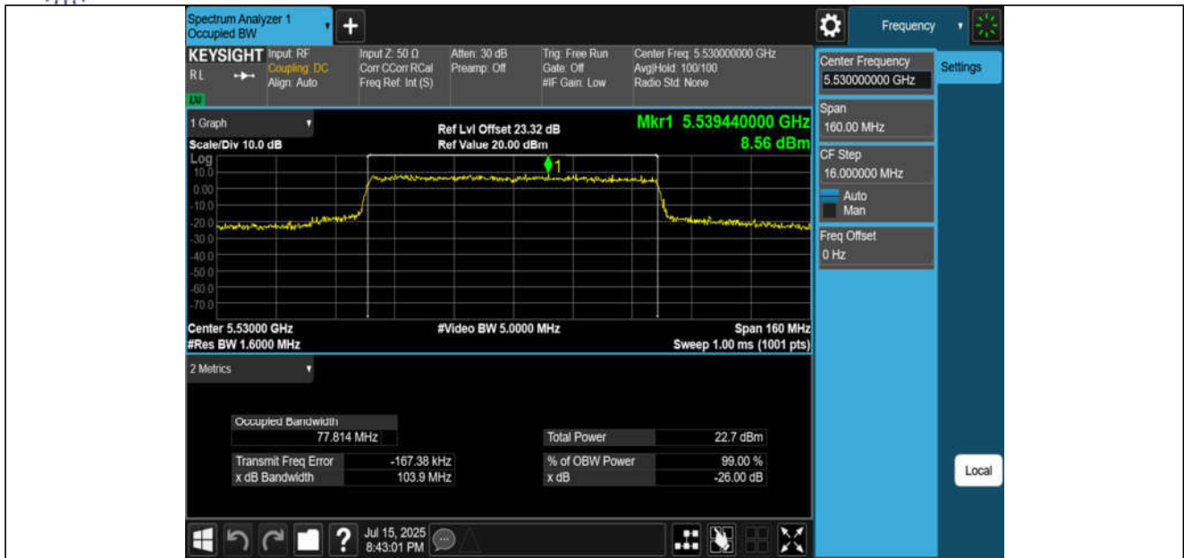
11AX80MIMO-Ant1-5530
