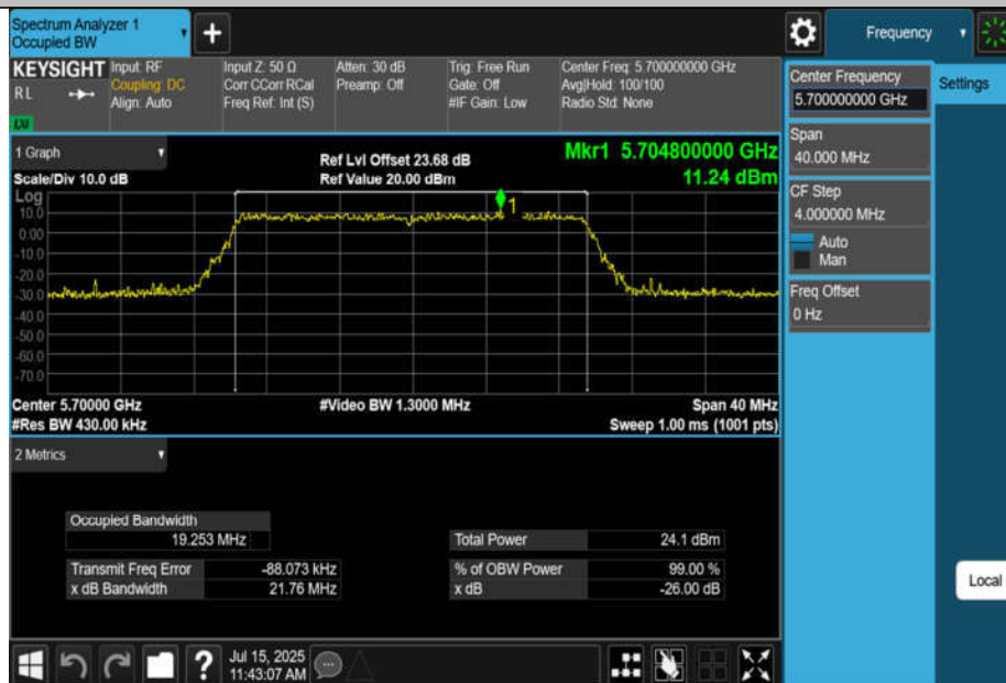
11AX20MIMO-Ant2-5700
