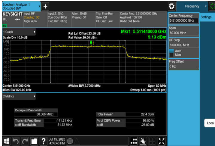
11AX40MIMO-Ant1-5510
