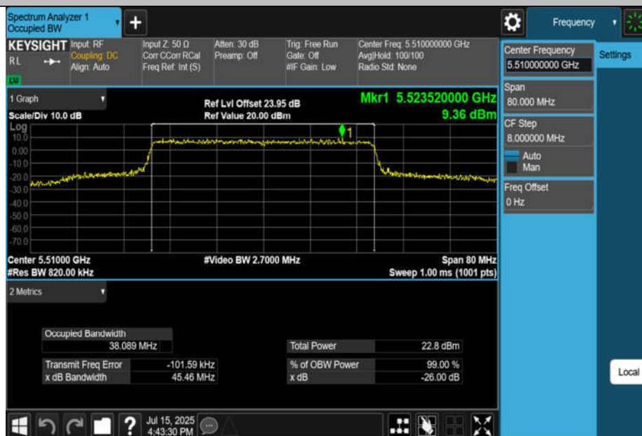
11AX40MIMO-Ant4-5510
