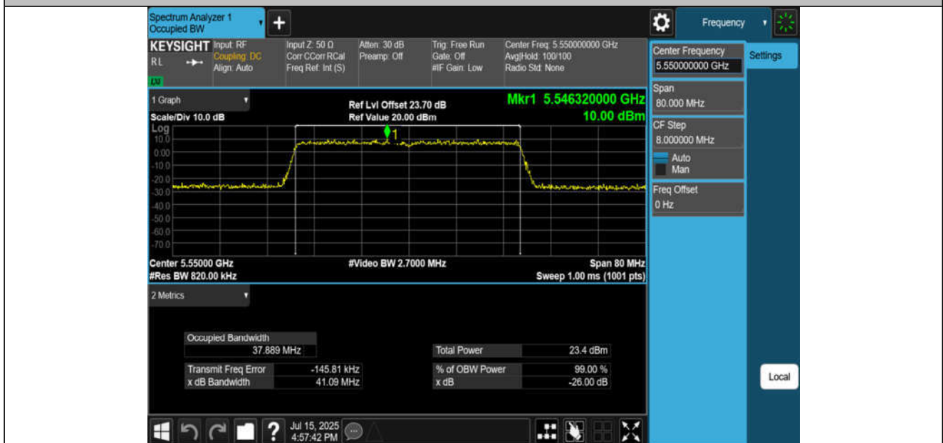
11AX40MIMO-Ant4-5550
