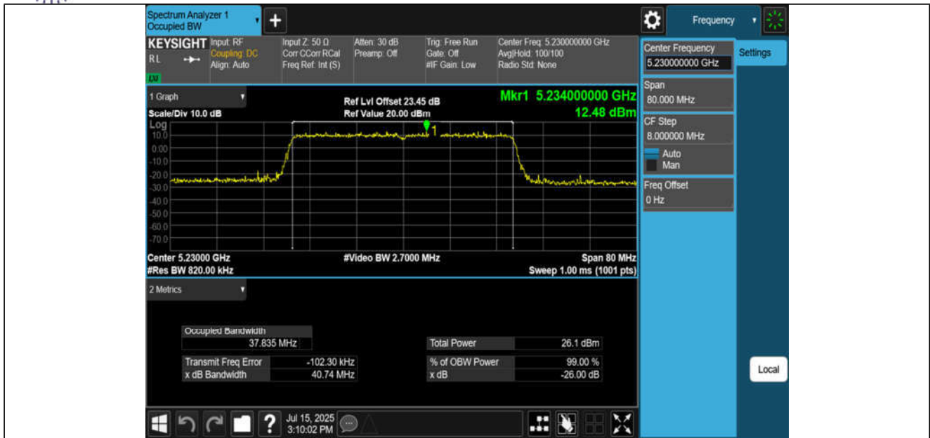
11AX40MIMO-Ant1-5230
