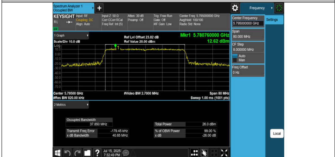
11AX40MIMO-Ant2-5795
