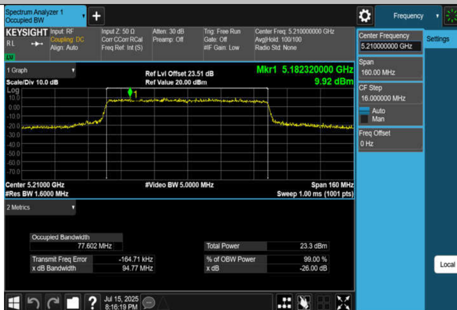
11AX80MIMO-Ant2-5210
