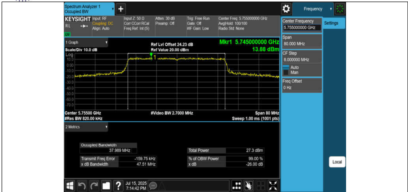
11AX40MIMO-Ant3-5755
