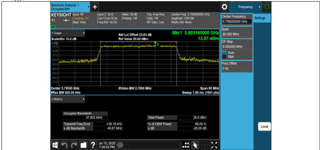
11AX40MIMO-Ant1-5795
