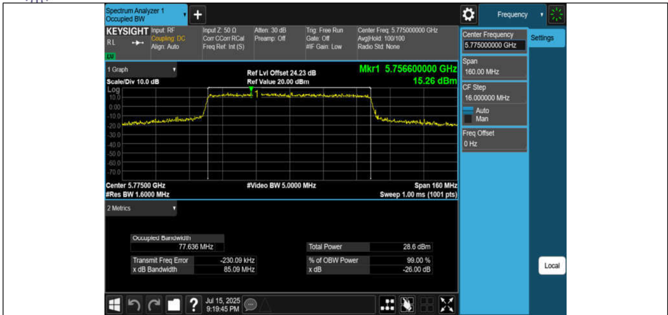
11AX80MIMO-Ant3-5775
