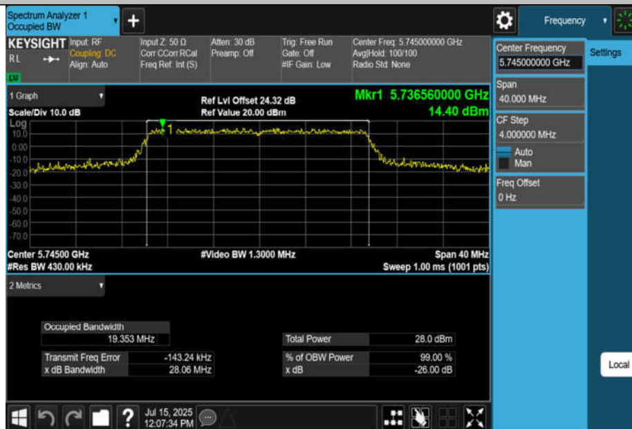
11AX20MIMO-Ant4-5745
