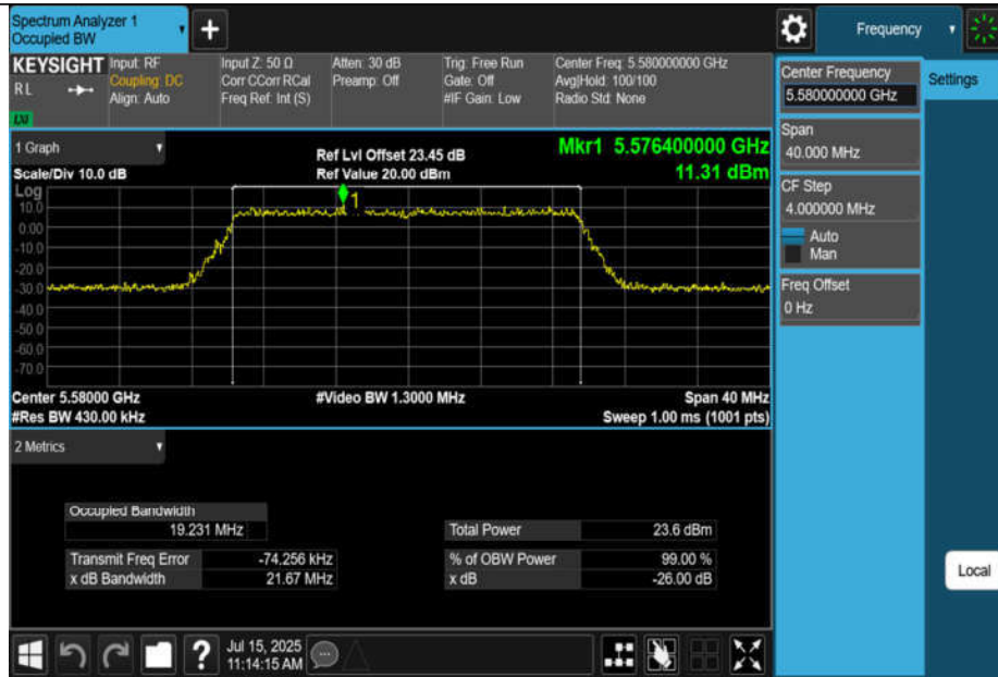
11AX20MIMO-Ant1-5580
