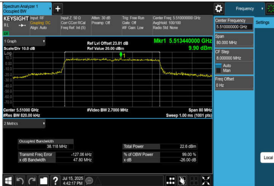
11AX40MIMO-Ant3-5510
