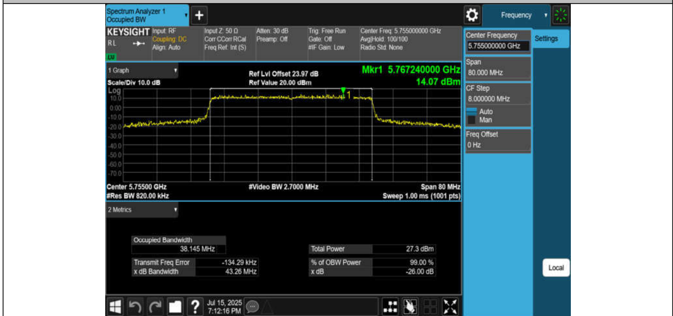
11AX40MIMO-Ant2-5755
