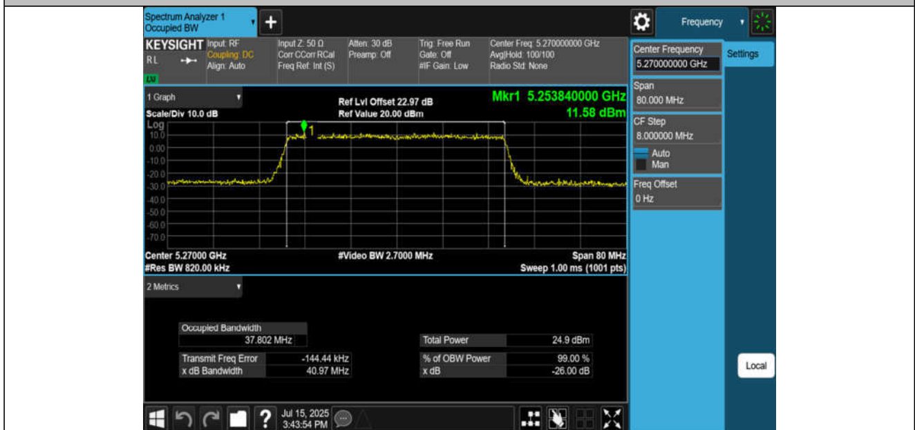
11AX40MIMO-Ant2-5270
