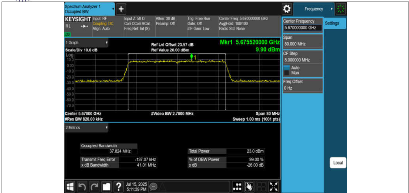
11AX40MIMO-Ant3-5670
