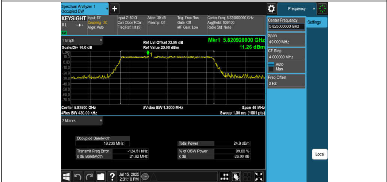
11AX20MIMO-Ant4-5825
