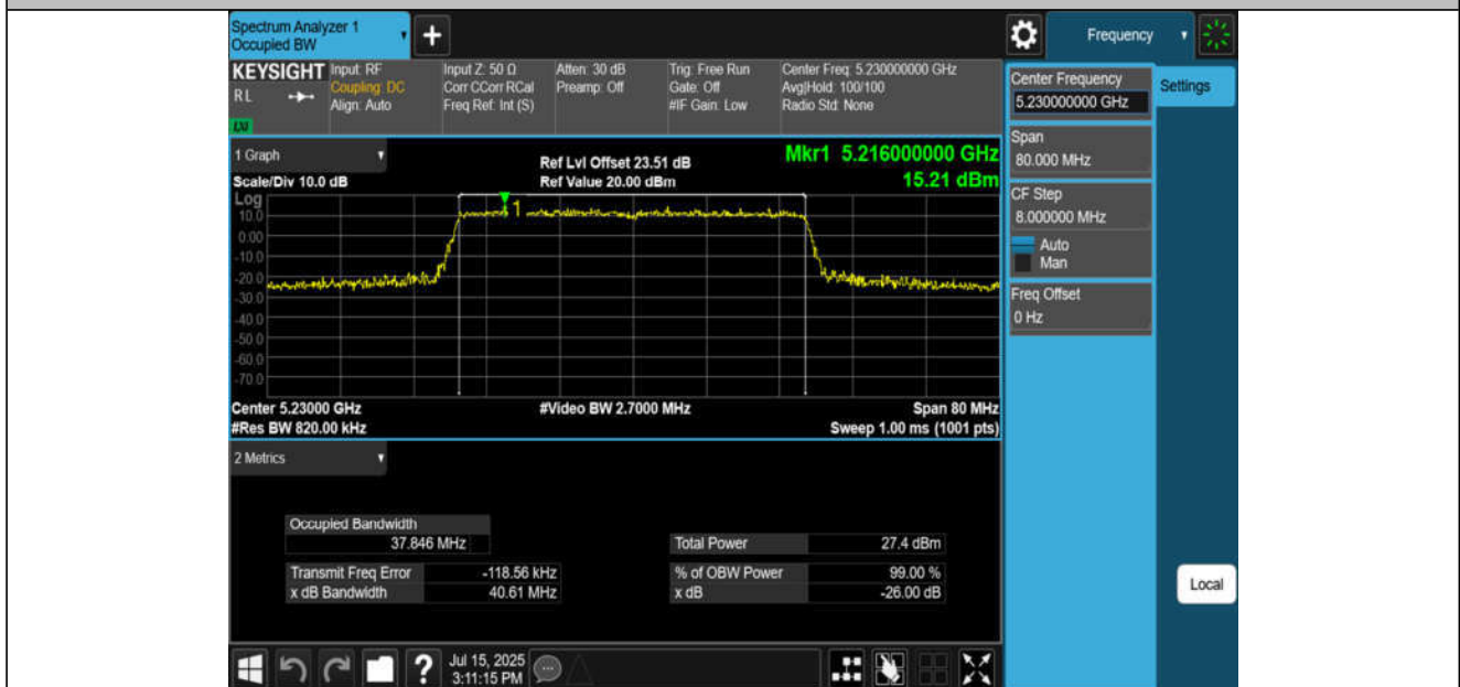
11AX40MIMO-Ant2-5230
