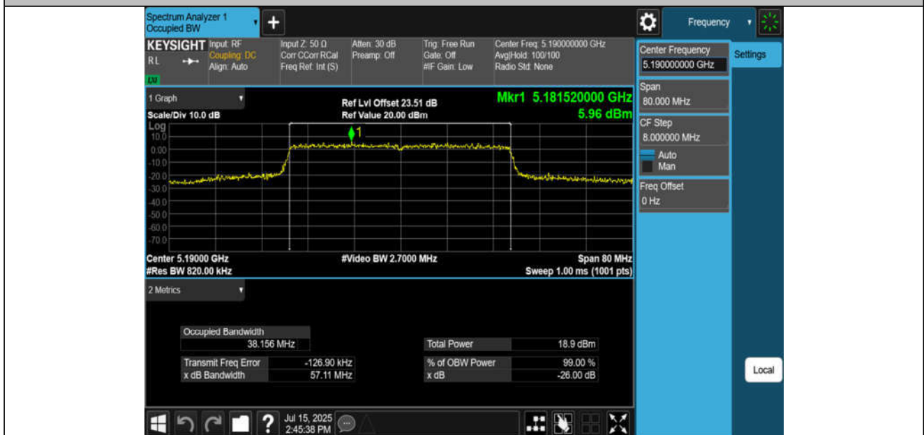
11AX40MIMO-Ant2-5190
