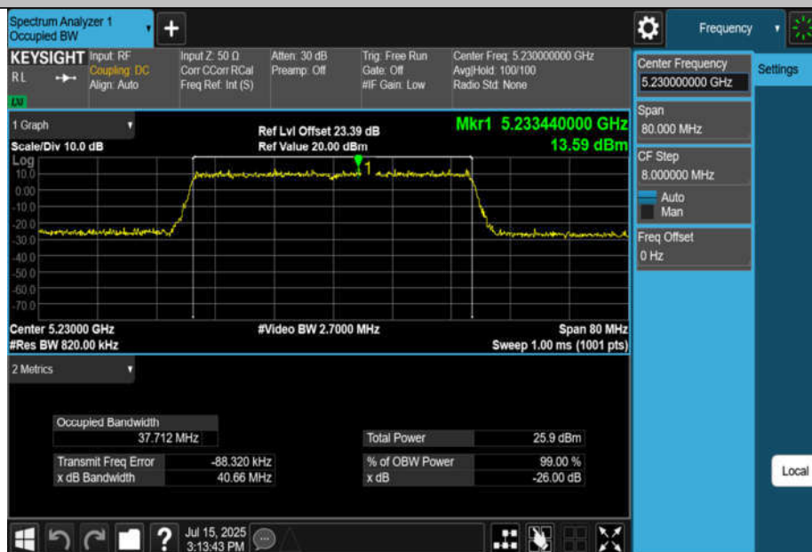
11AX40MIMO-Ant4-5230
