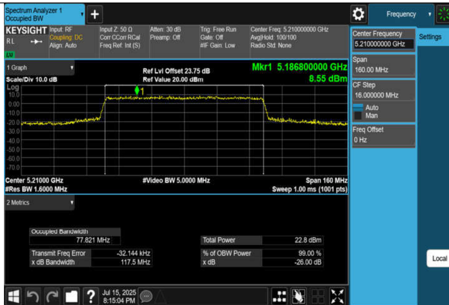
11AX80MIMO-Ant1-5210
