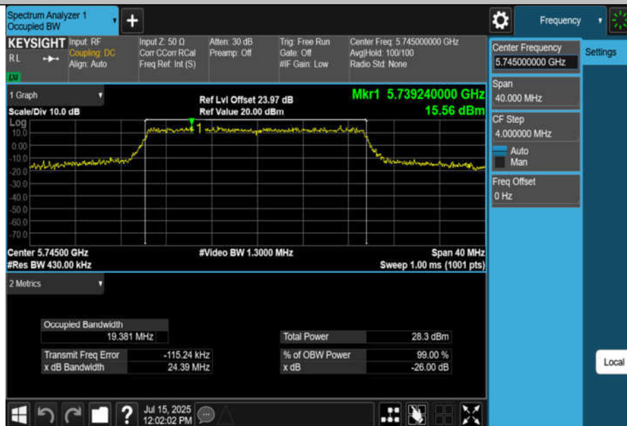
11AX20MIMO-Ant2-5745
