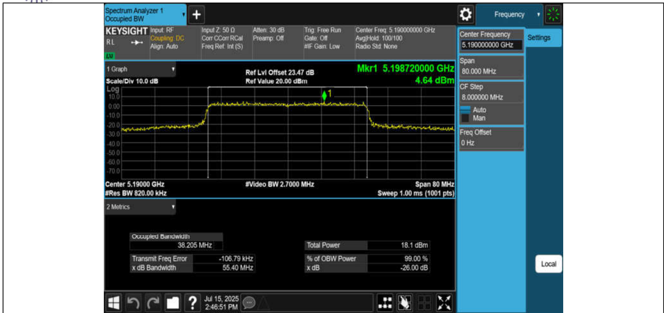
11AX40MIMO-Ant3-5190
