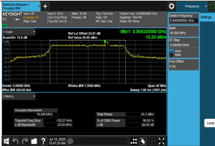
11AX20MIMO-Ant3-5500
