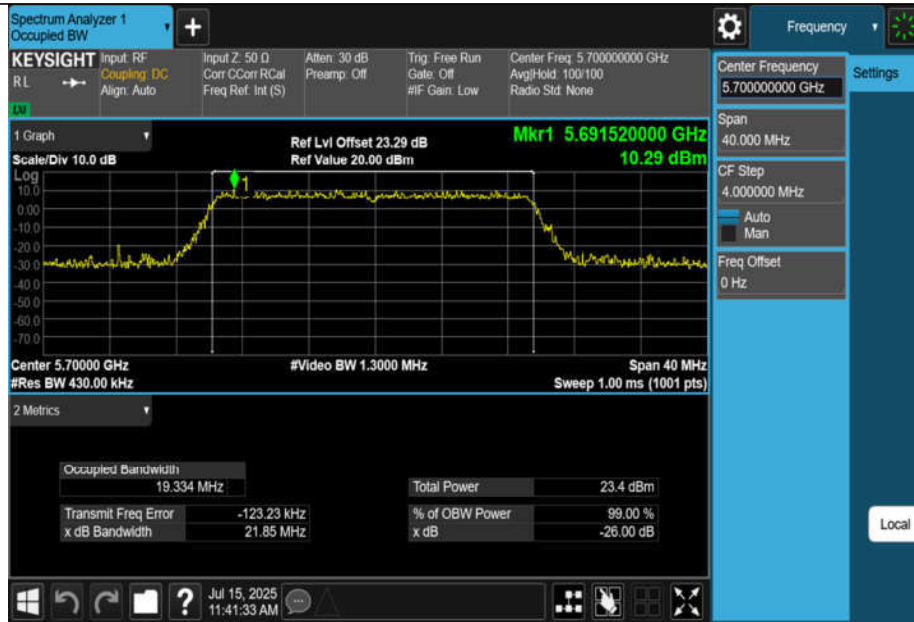
11AX20MIMO-Ant1-5700
