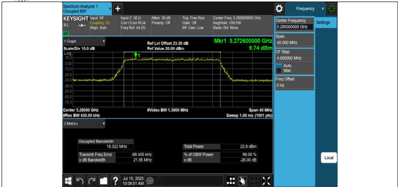
11AX20MIMO-Ant1-5280
