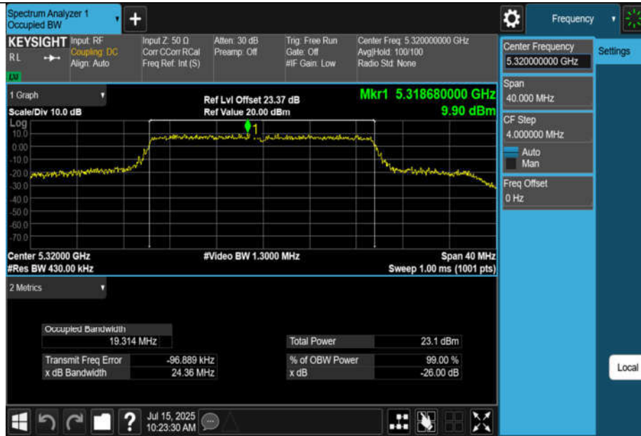
11AX20MIMO-Ant1-5320
