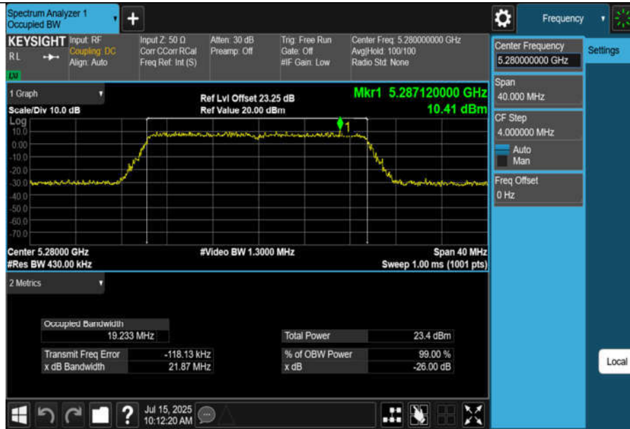
11AX20MIMO-Ant3-5280
