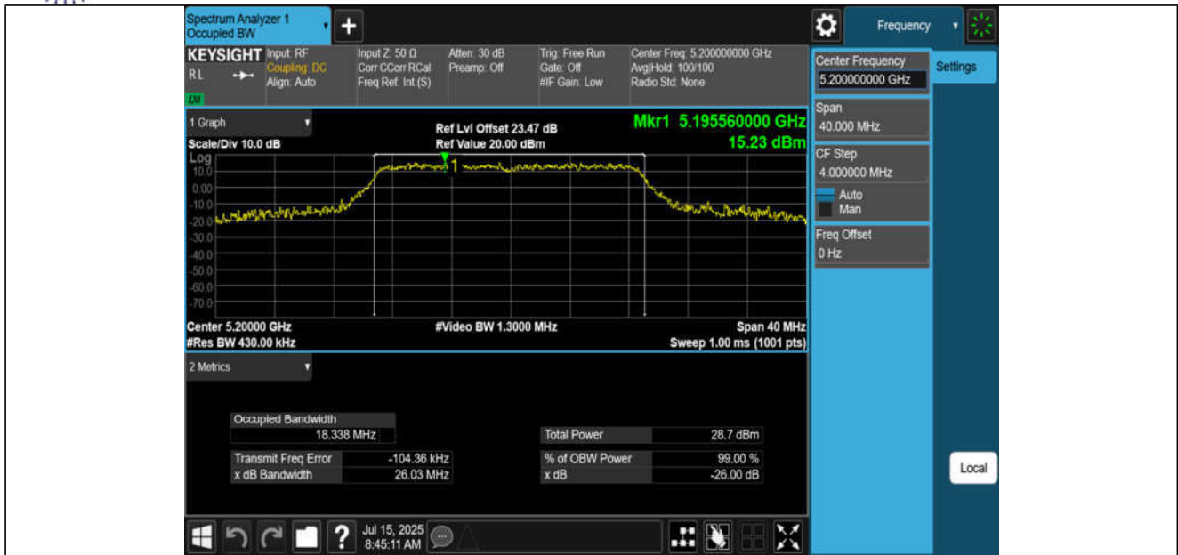
11AX20MIMO-Ant3-5200
