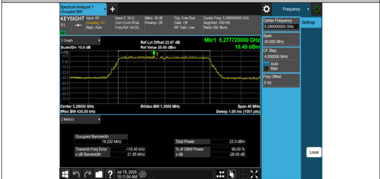
11AX20MIMO-Ant2-5280
