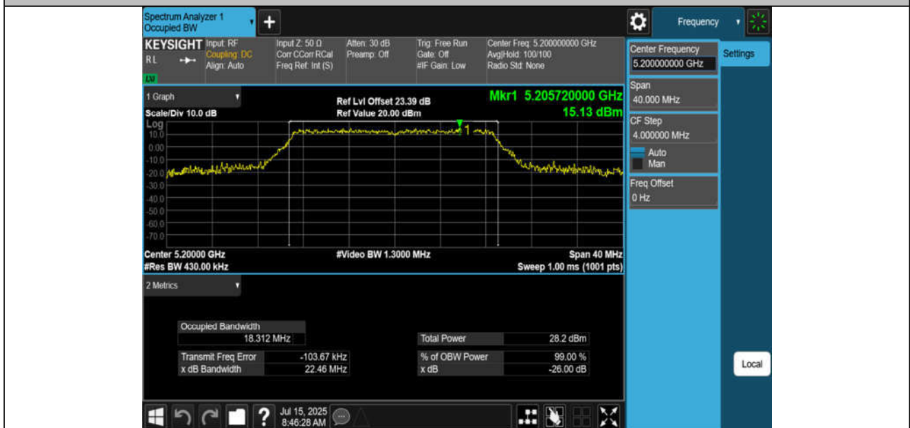
11AX20MIMO-Ant4-5200
