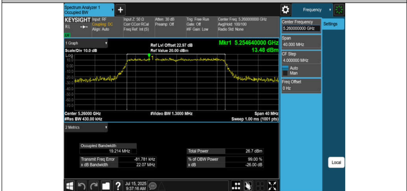
11AX20MIMO-Ant2-5260
