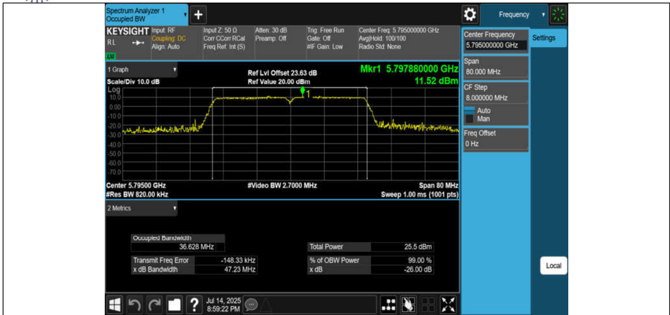
11AC40MIMO-Ant1-5795
