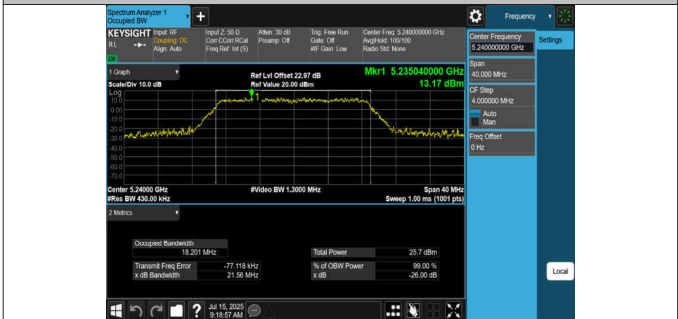
11AX20MIMO-Ant2-5240
