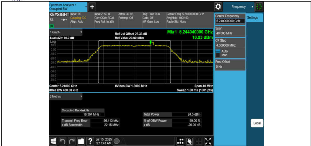
11AX20MIMO-Ant1-5240
