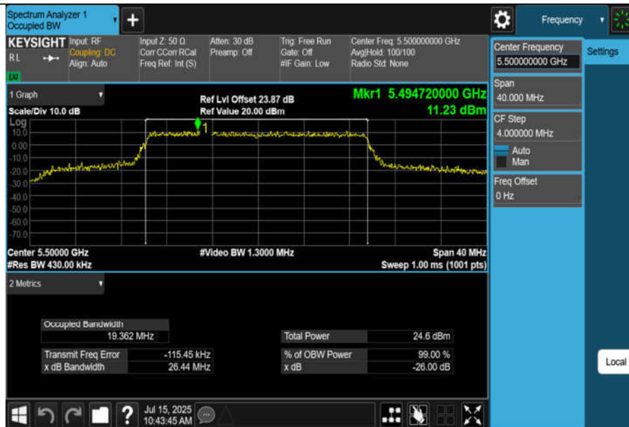
11AX20MIMO-Ant1-5500
