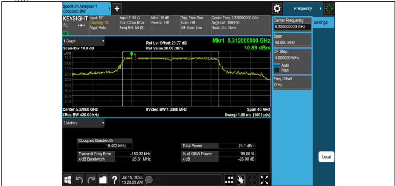
11AX20MIMO-Ant3-5320
