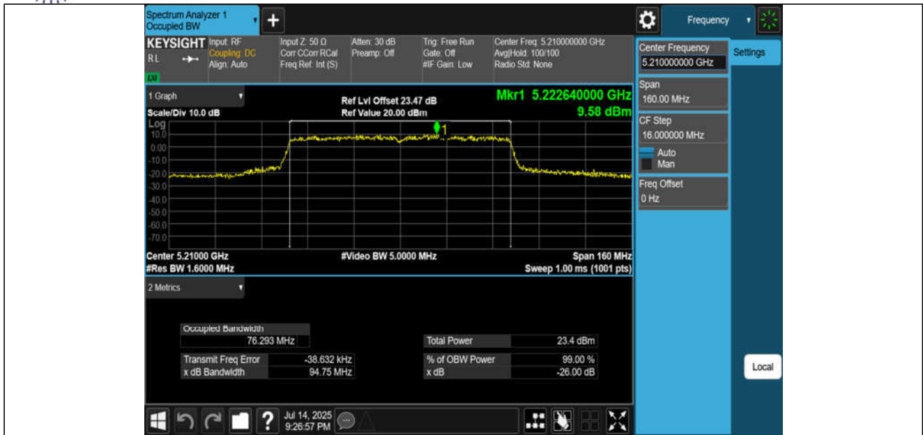
11AC80MIMO-Ant3-5210
