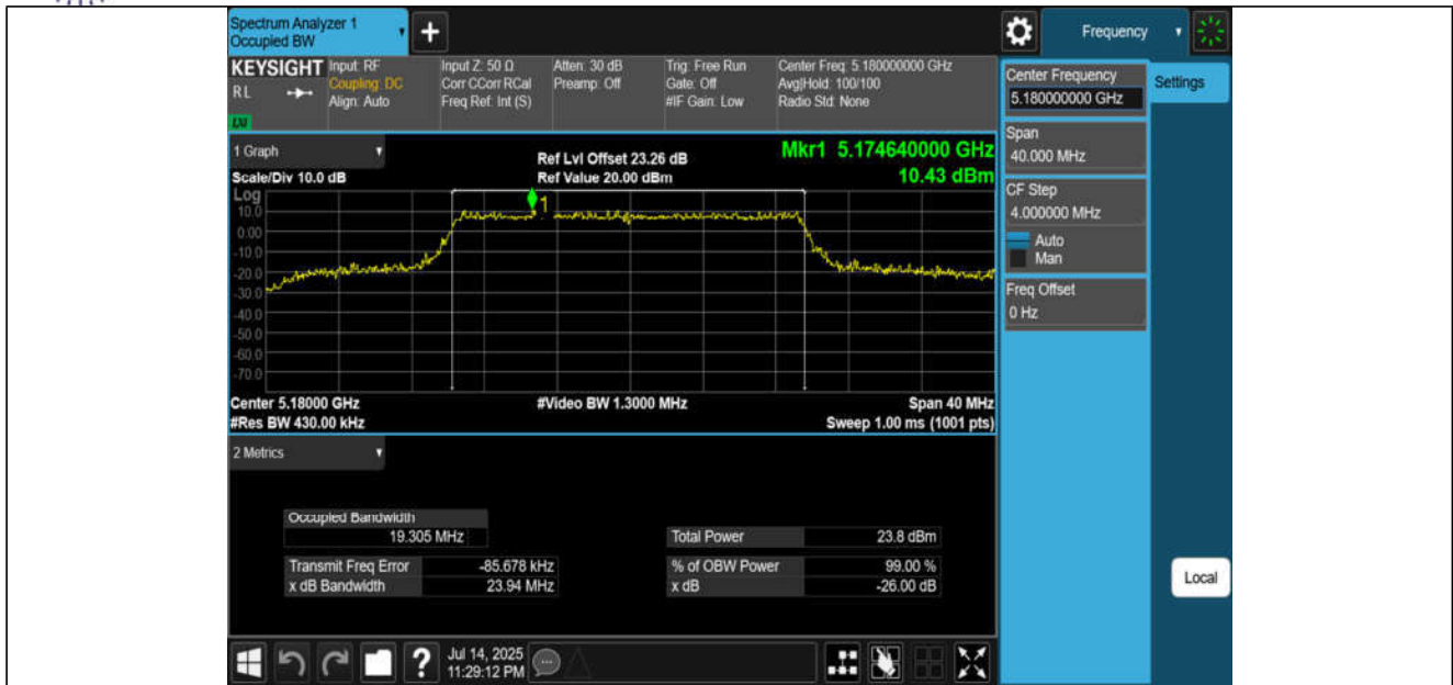
11AX20MIMO-Ant1-5180
