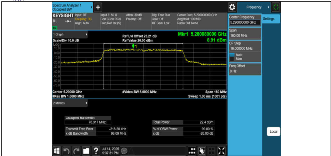
11AC80MIMO-Ant1-5290
