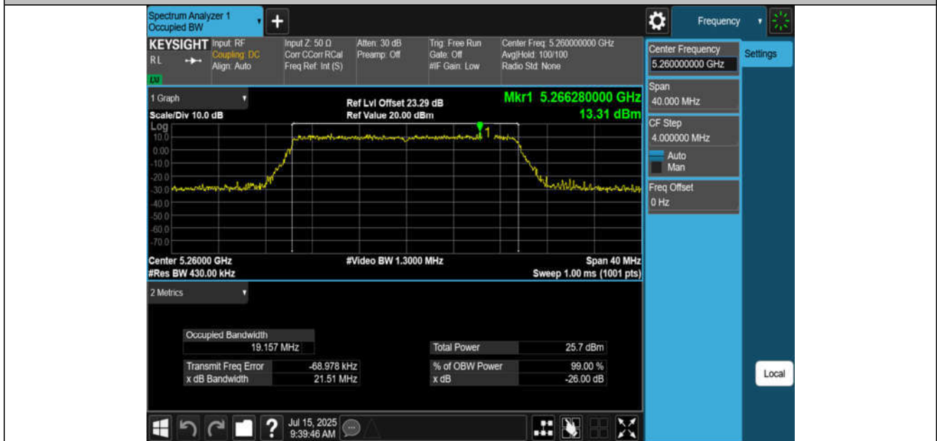
11AX20MIMO-Ant4-5260
