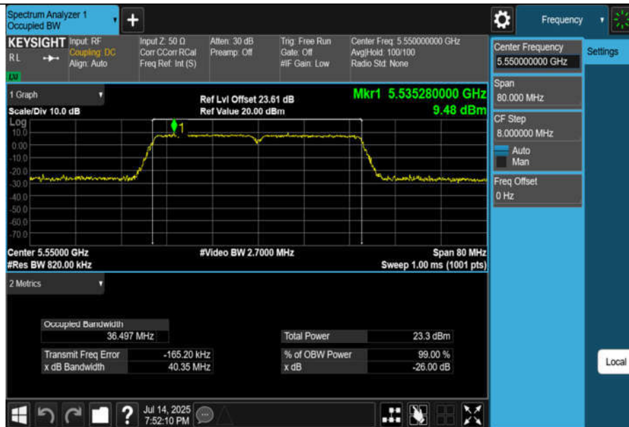
11AC40MIMO-Ant1-5550
