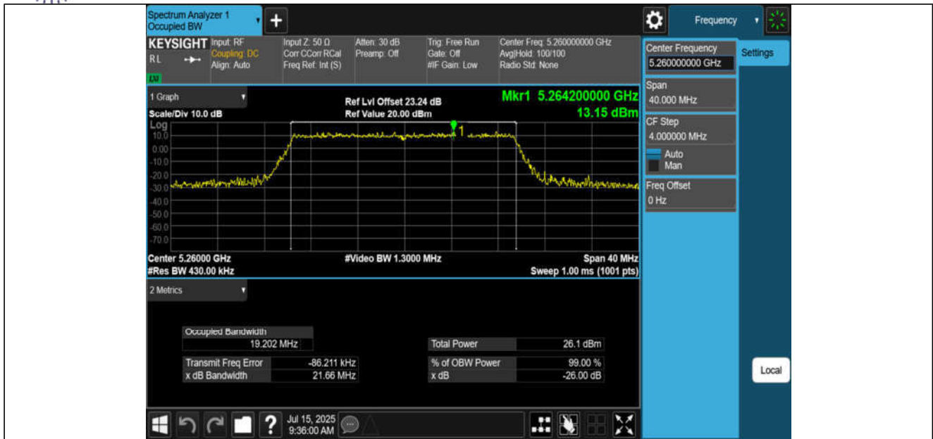
11AX20MIMO-Ant1-5260
