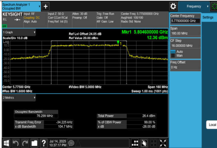
11AC80MIMO-Ant1-5775
