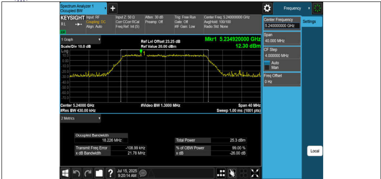
11AX20MIMO-Ant3-5240
