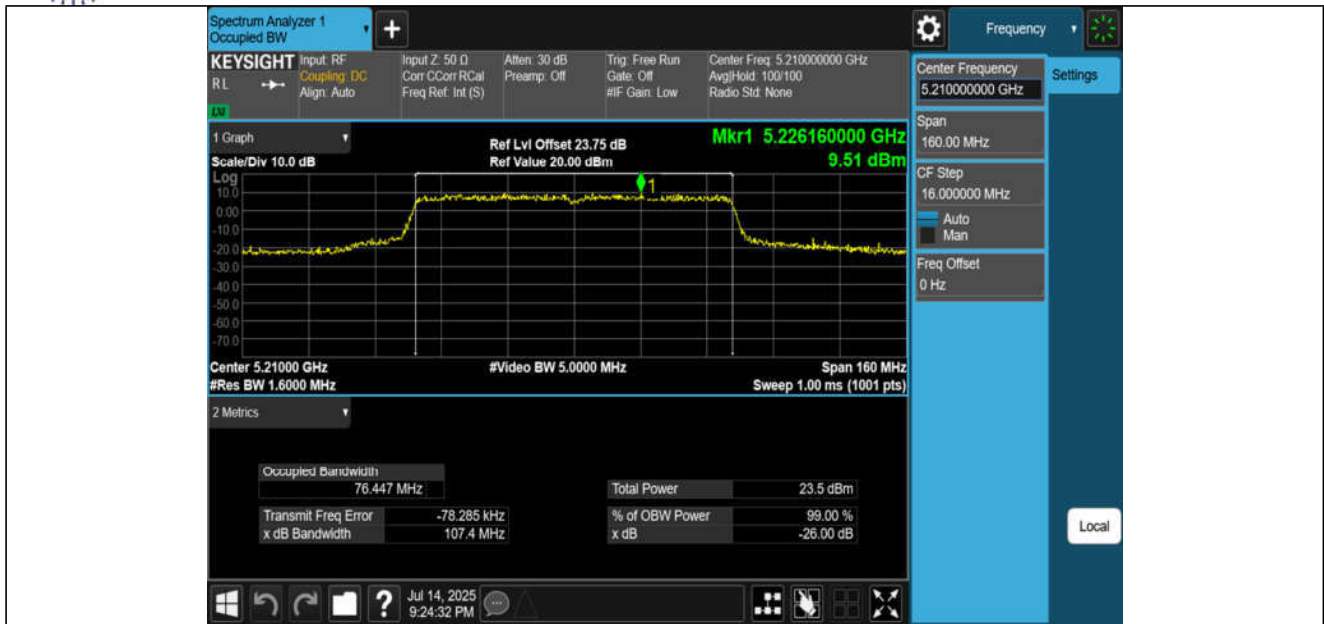
11AC80MIMO-Ant1-5210
