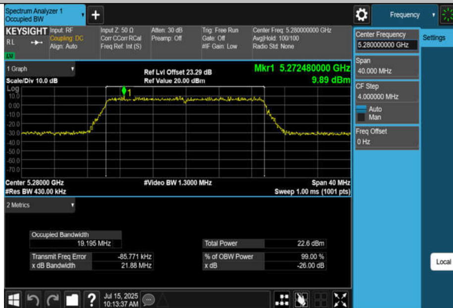
11AX20MIMO-Ant4-5280
