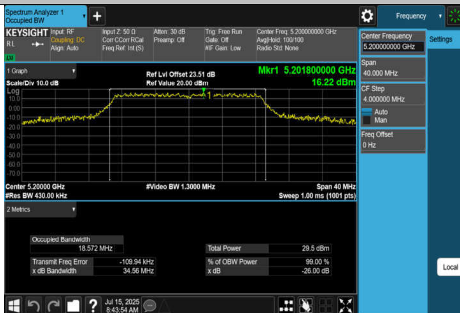
11AX20MIMO-Ant2-5200
