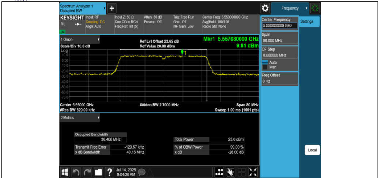
11N40MIMO-Ant3-5550
