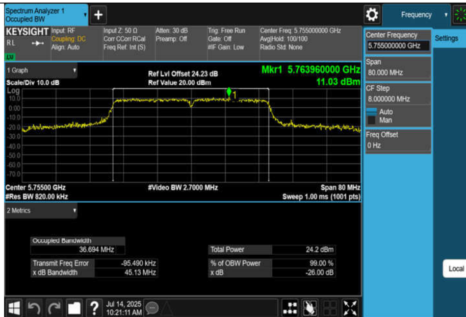
11N40MIMO-Ant3-5755
