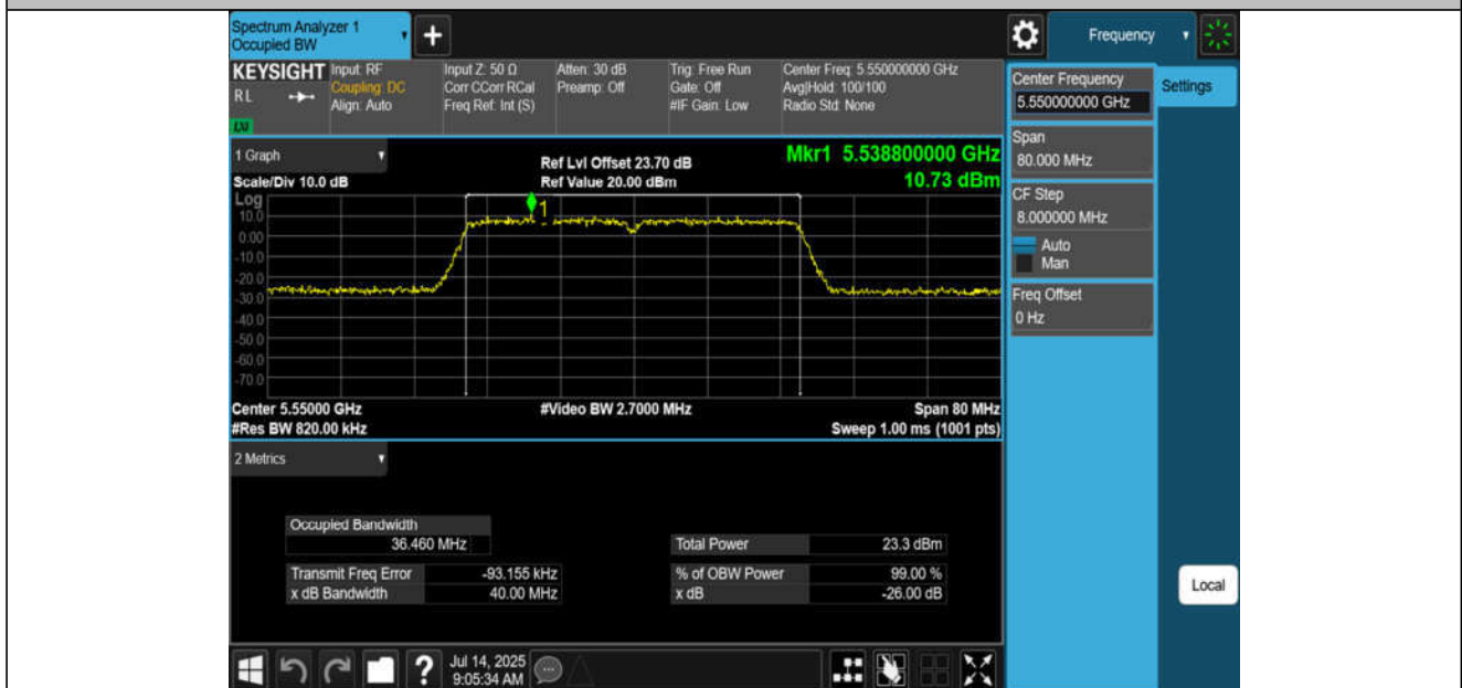
11N40MIMO-Ant4-5550
