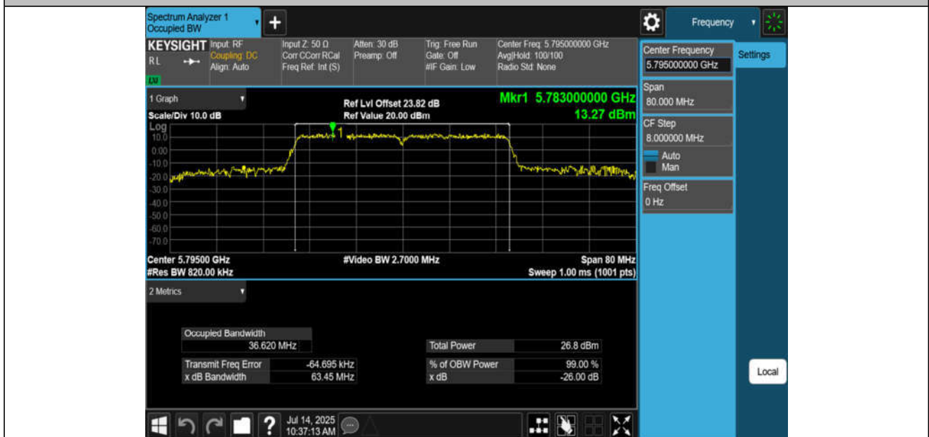
11N40MIMO-Ant2-5795
