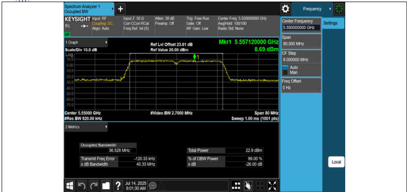
11N40MIMO-Ant1-5550
