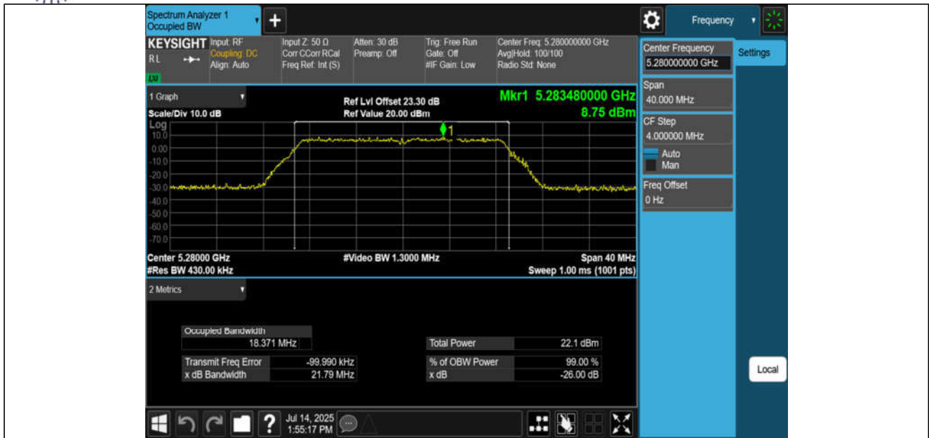
11AC20MIMO-Ant1-5280
