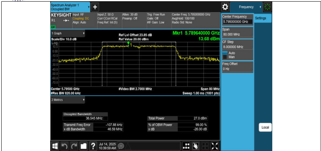
11N40MIMO-Ant3-5795
