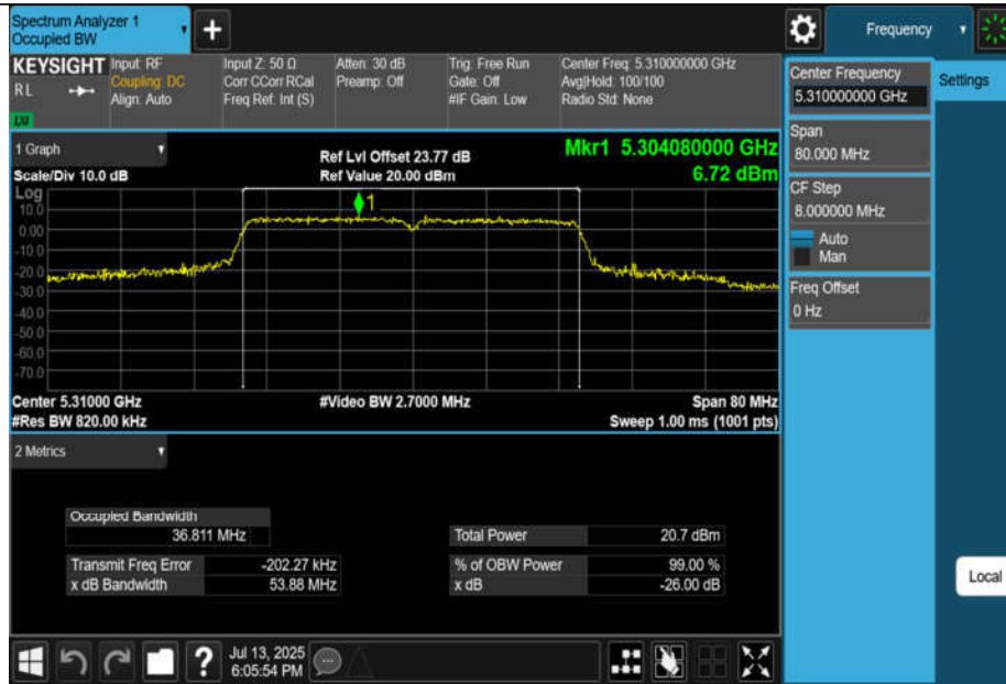
11N40MIMO-Ant3-5310
