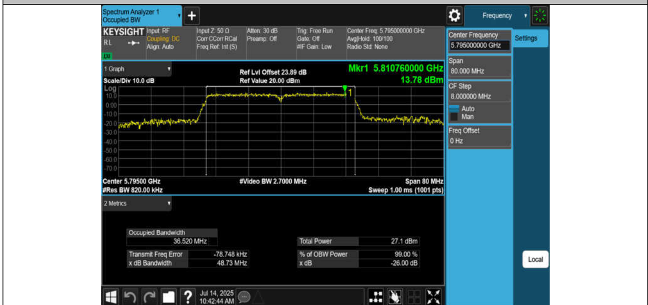
11N40MIMO-Ant4-5795
