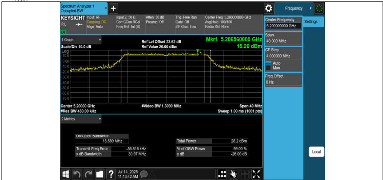
11AC20MIMO-Ant1-5200
