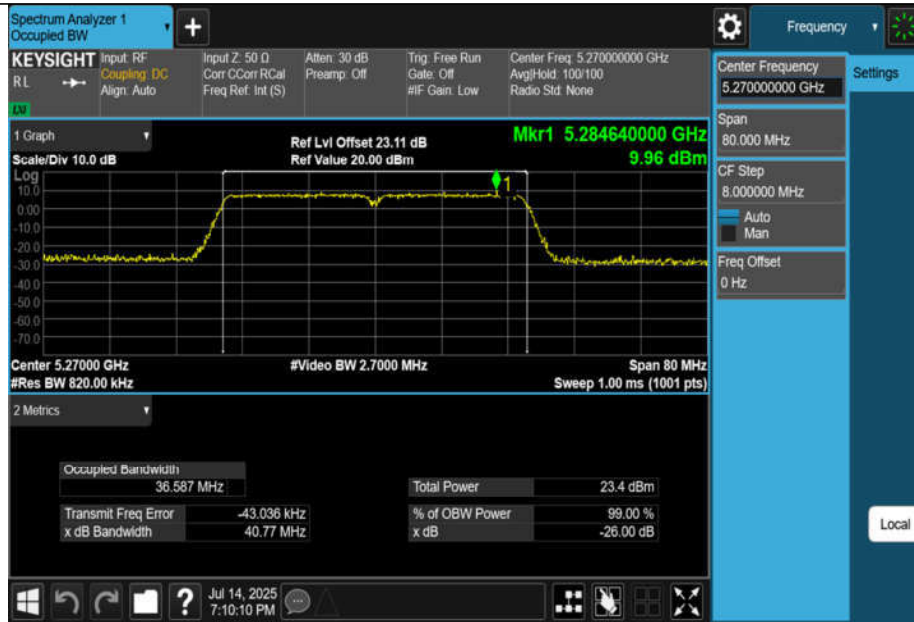
11AC40MIMO-Ant1-5270
