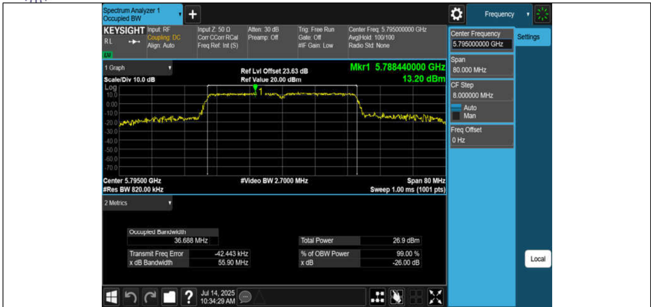
11N40MIMO-Ant1-5795
