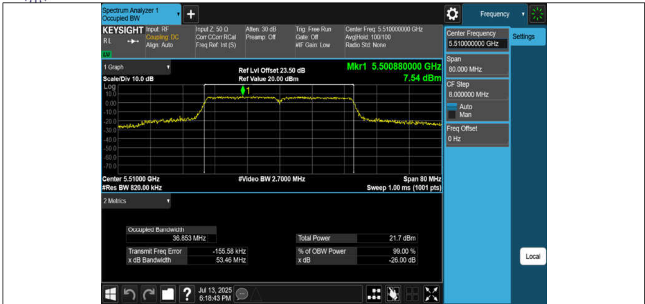
11N40MIMO-Ant1-5510
