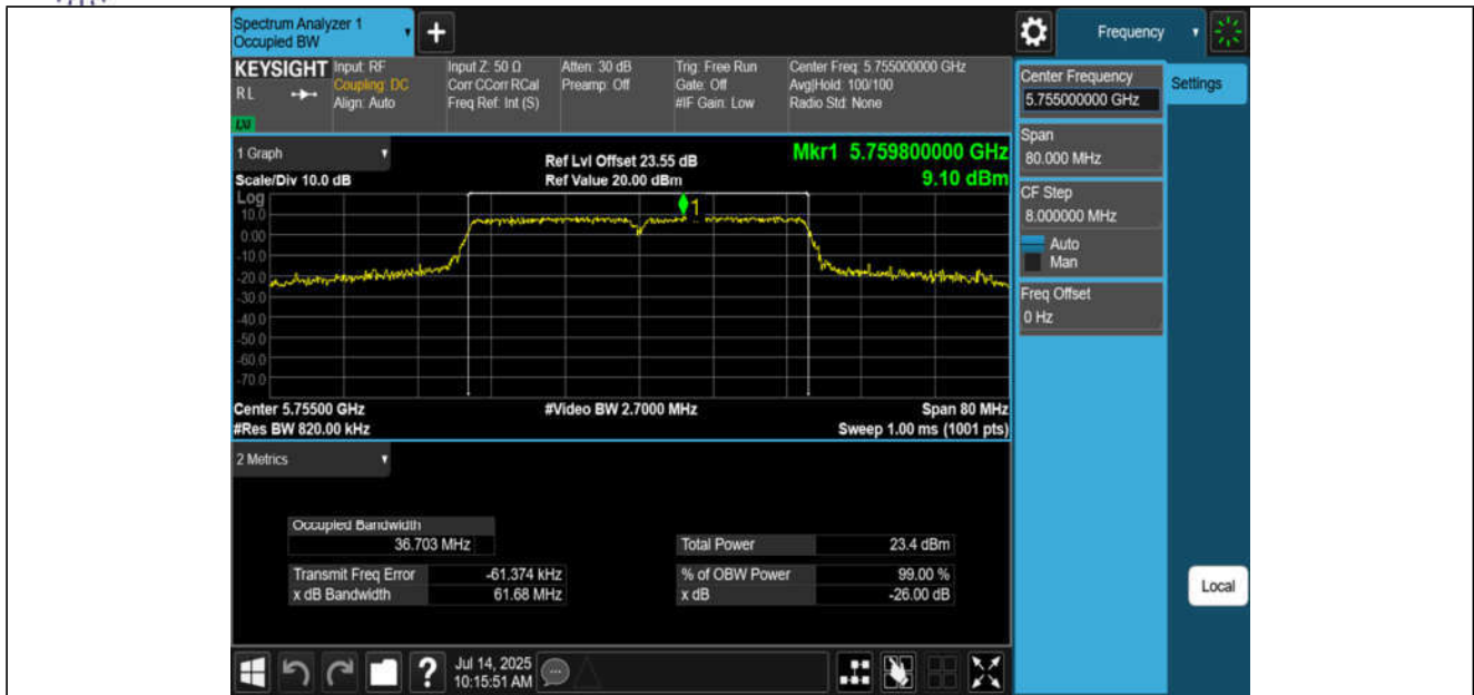
11N40MIMO-Ant1-5755
