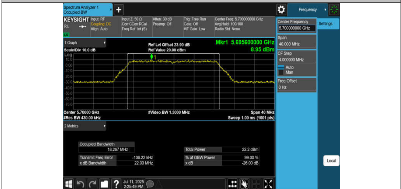
11N20MIMO-Ant4-5700
