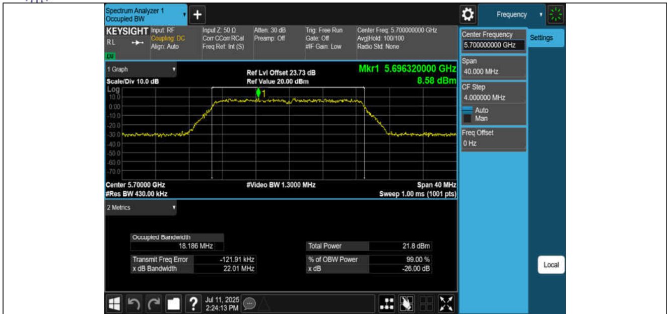
11N20MIMO-Ant3-5700
