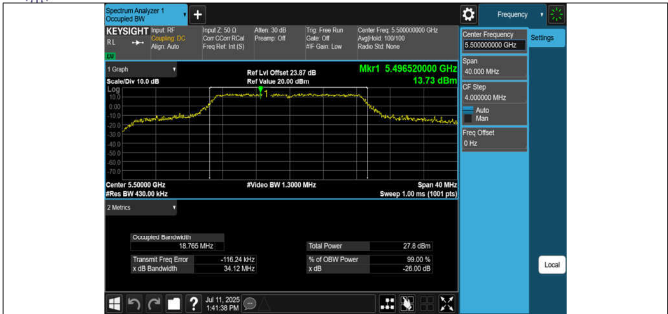
11N20MIMO-Ant1-5500
