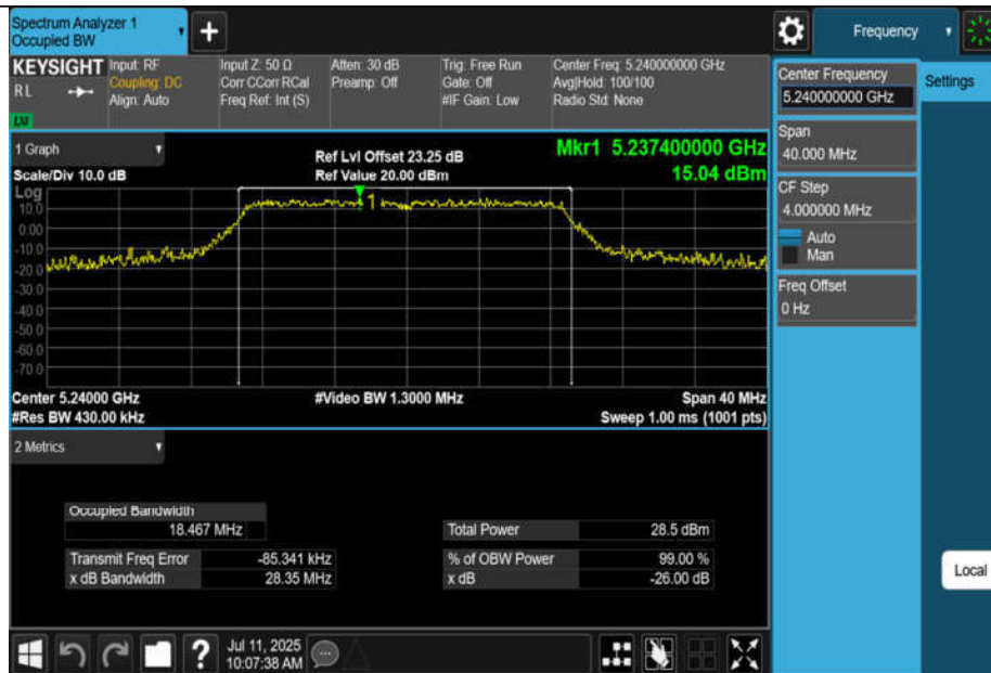
11N20MIMO-Ant3-5240
