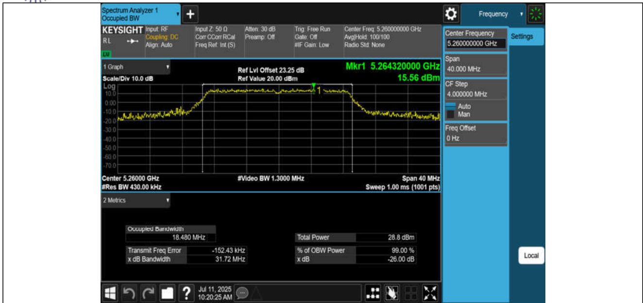
11N20MIMO-Ant3-5260
