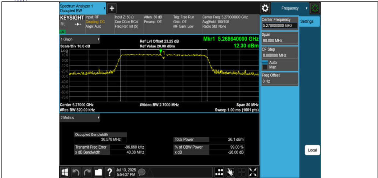
11N40MIMO-Ant3-5270
