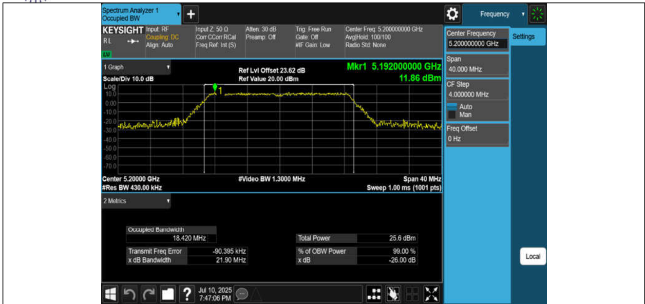
11N20MIMO-Ant1-5200
