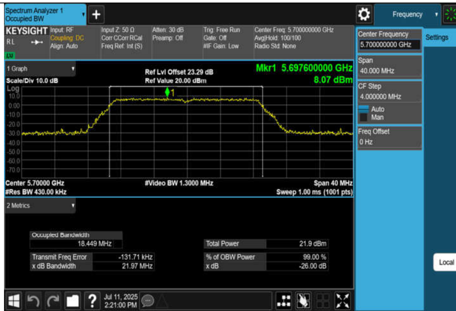
11N20MIMO-Ant1-5700
