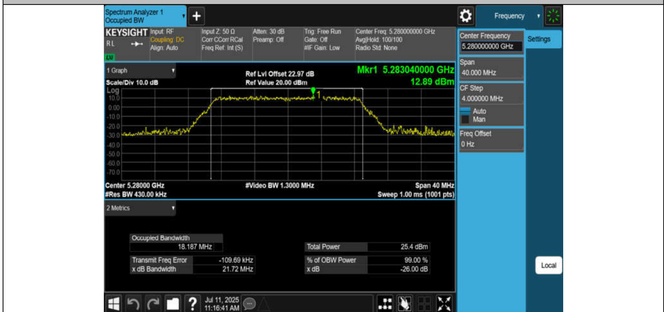
11N20MIMO-Ant2-5280
