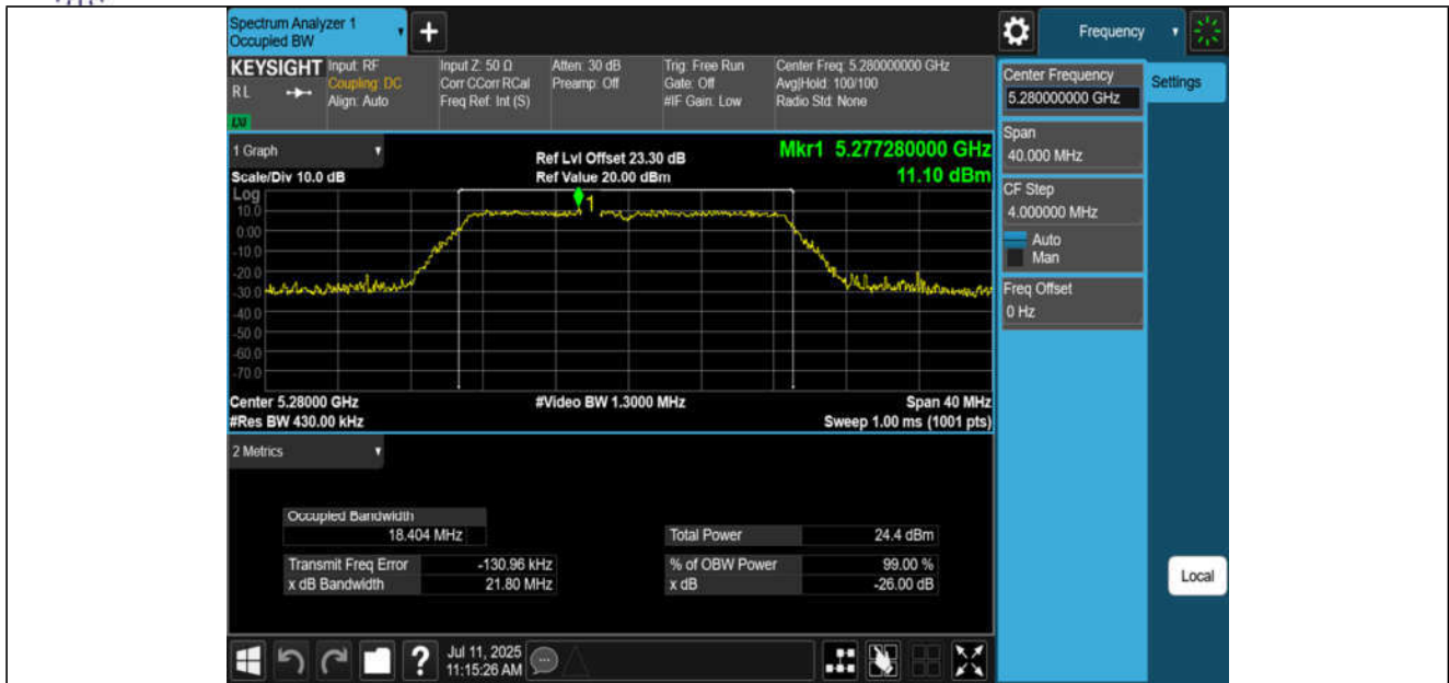
11N20MIMO-Ant1-5280
