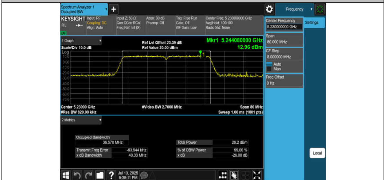
11N40MIMO-Ant4-5230
