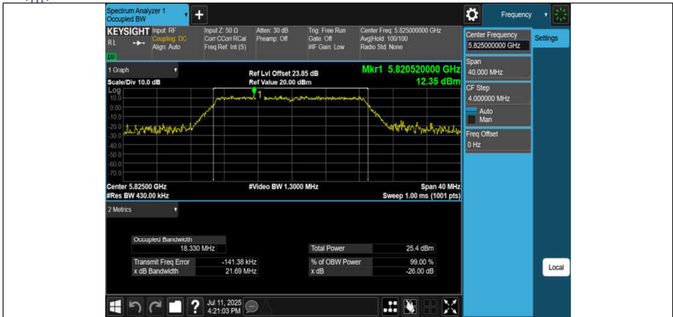
11N20MIMO-Ant3-5825
