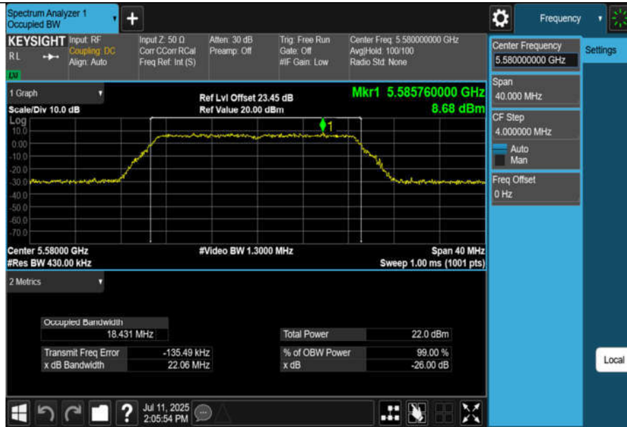
11N20MIMO-Ant1-5580
