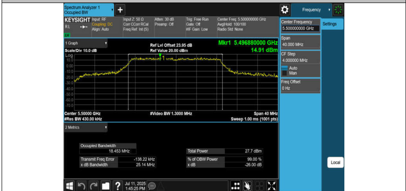
11N20MIMO-Ant4-5500
