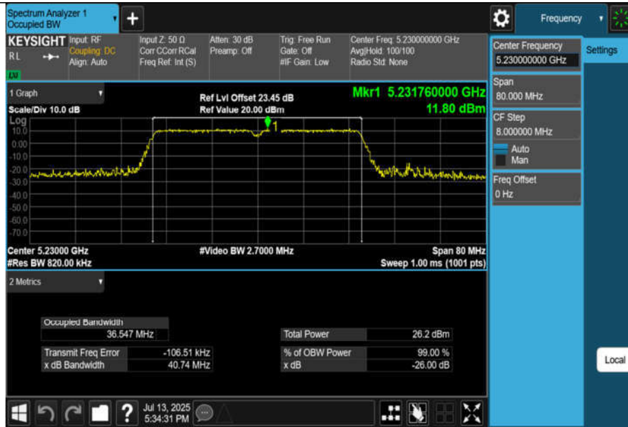
11N40MIMO-Ant1-5230
