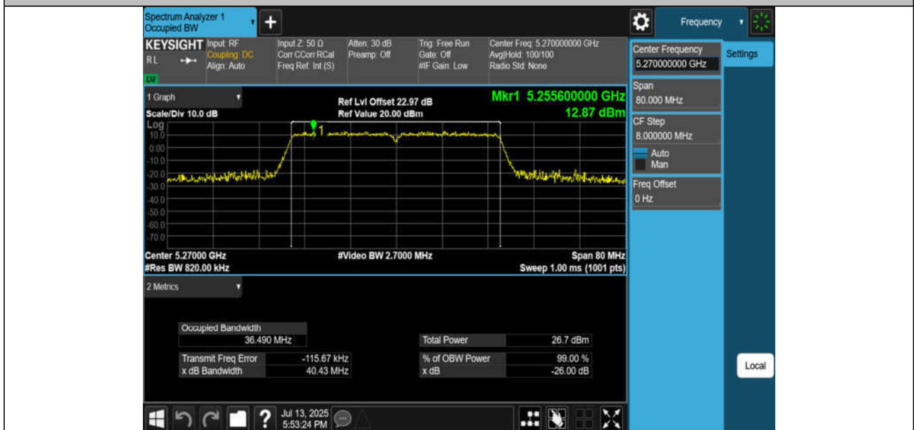
11N40MIMO-Ant2-5270
