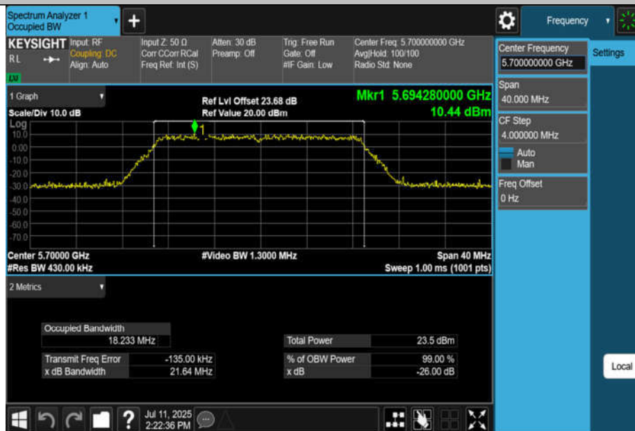
11N20MIMO-Ant2-5700
