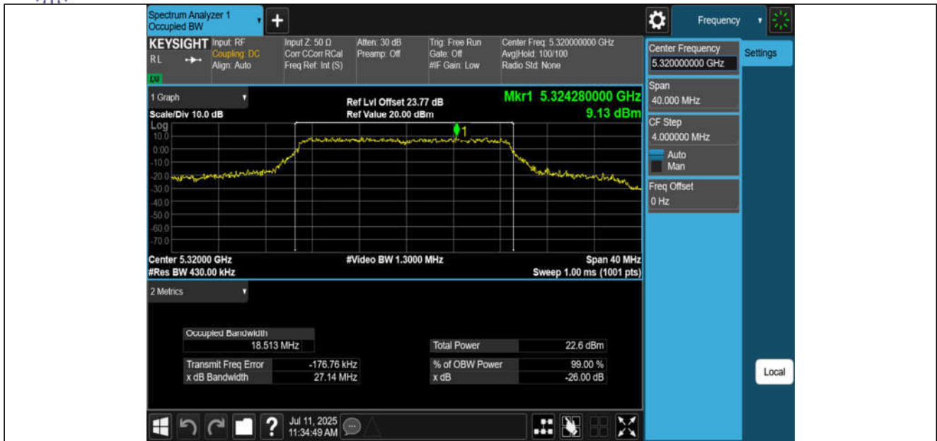
11N20MIMO-Ant3-5320
