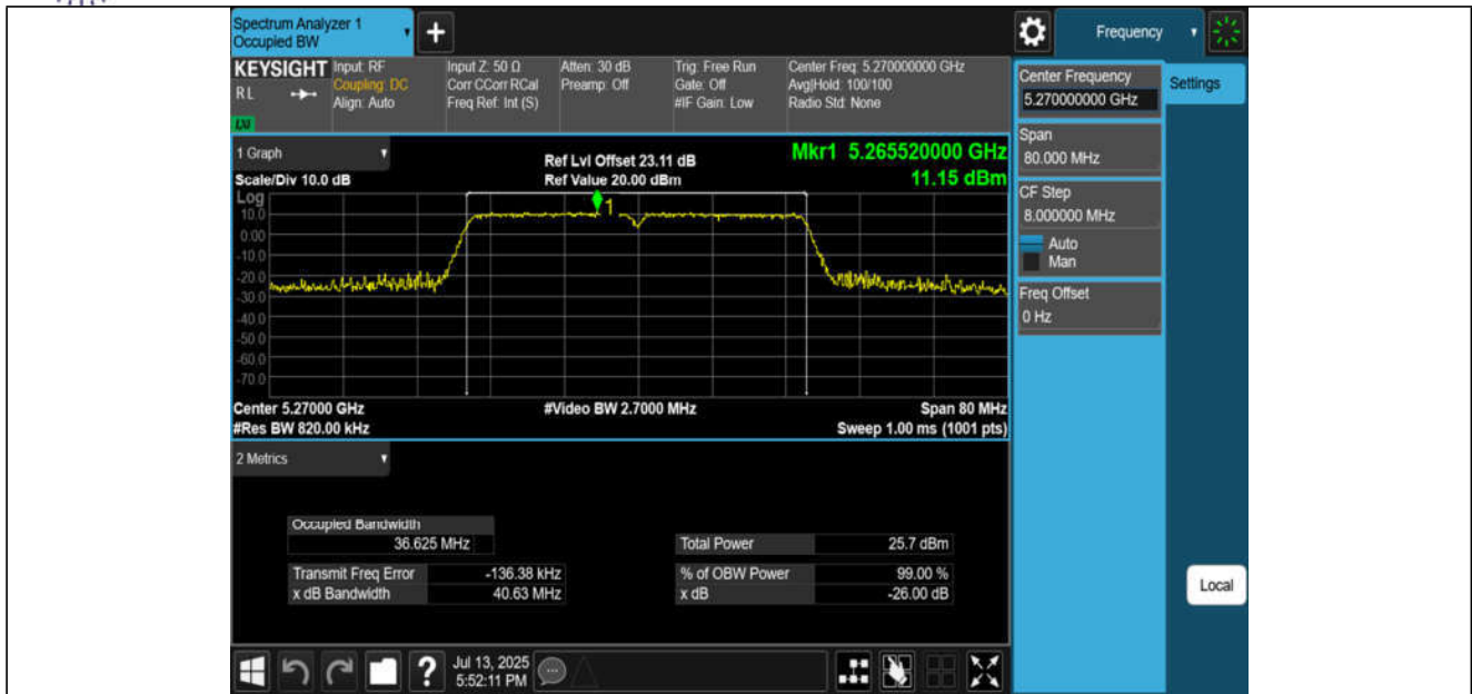
11N40MIMO-Ant1-5270
