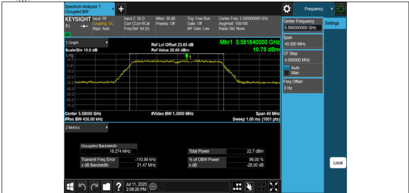
11N20MIMO-Ant3-5580
