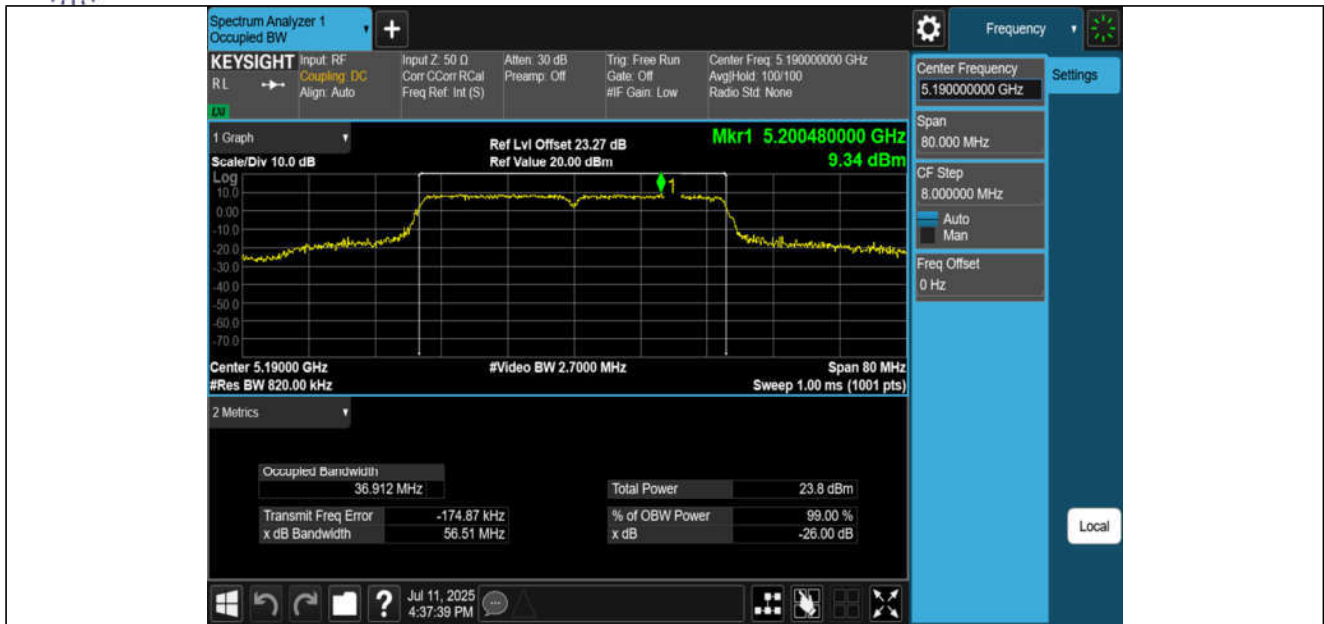
11N40MIMO-Ant1-5190
