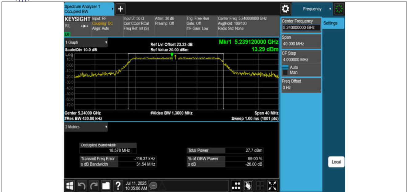
11N20MIMO-Ant1-5240
