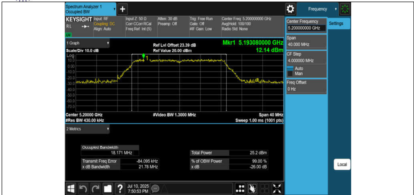
11N20MIMO-Ant4-5200
