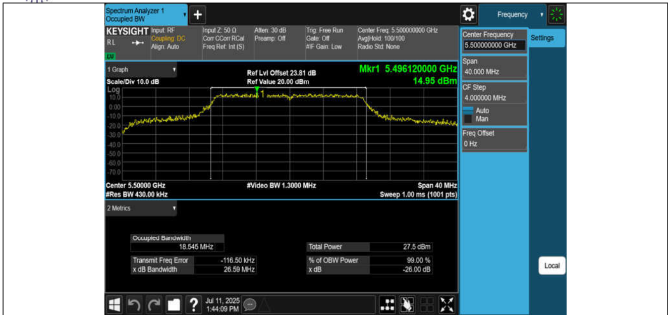
11N20MIMO-Ant3-5500
