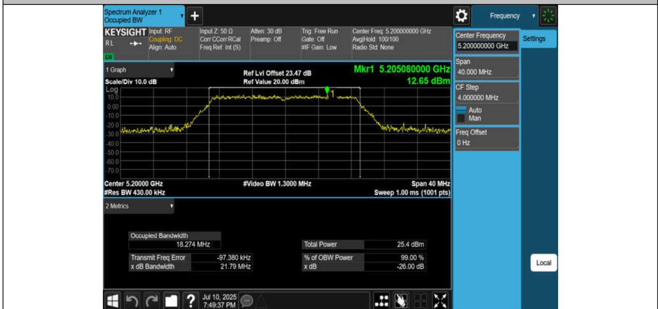
11N20MIMO-Ant3-5200
