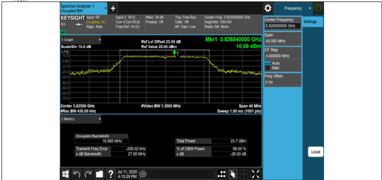
11N20MIMO-Ant1-5825
