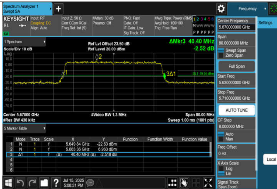
11AX40MIMO-Ant1-5670
