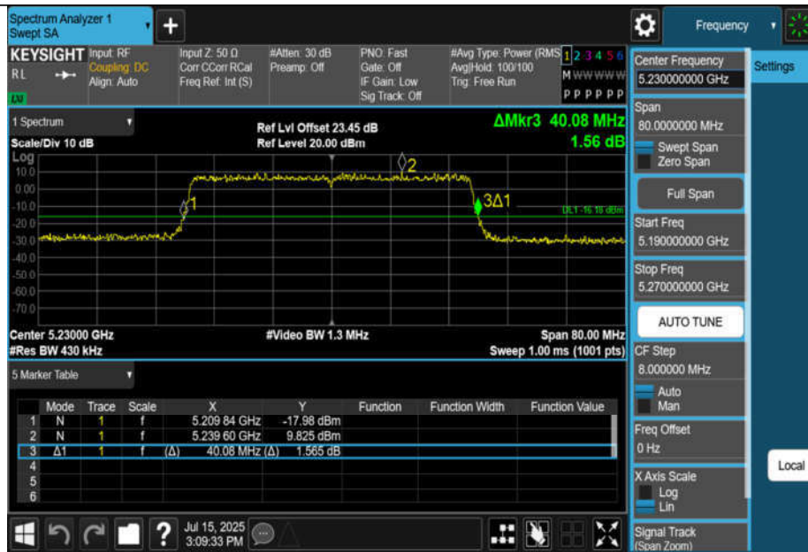
11AX40MIMO-Ant1-5230
