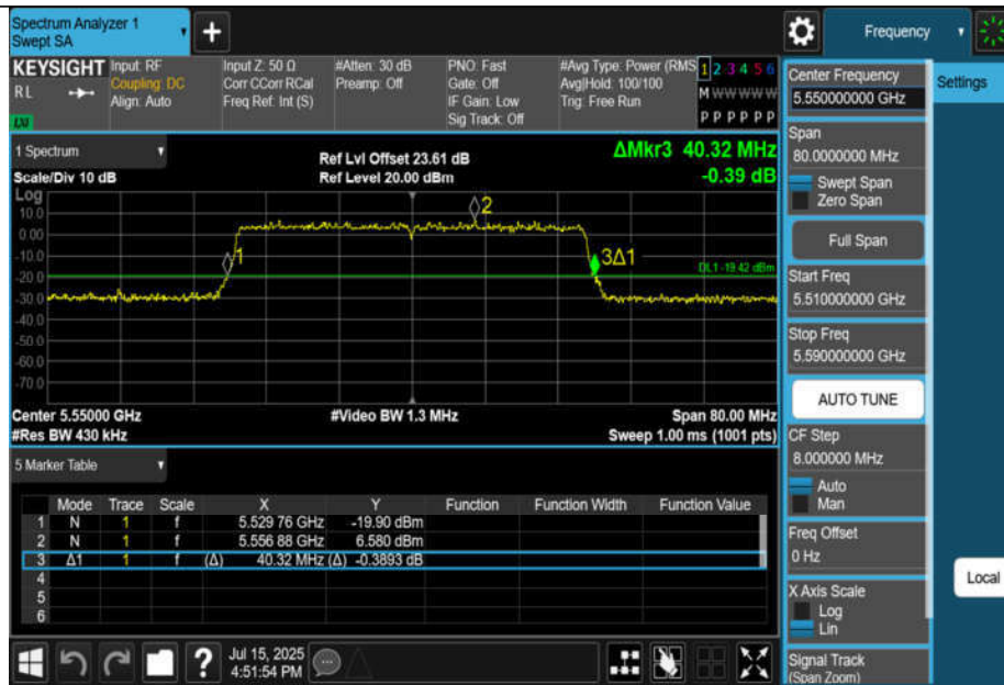
11AX40MIMO-Ant1-5550
