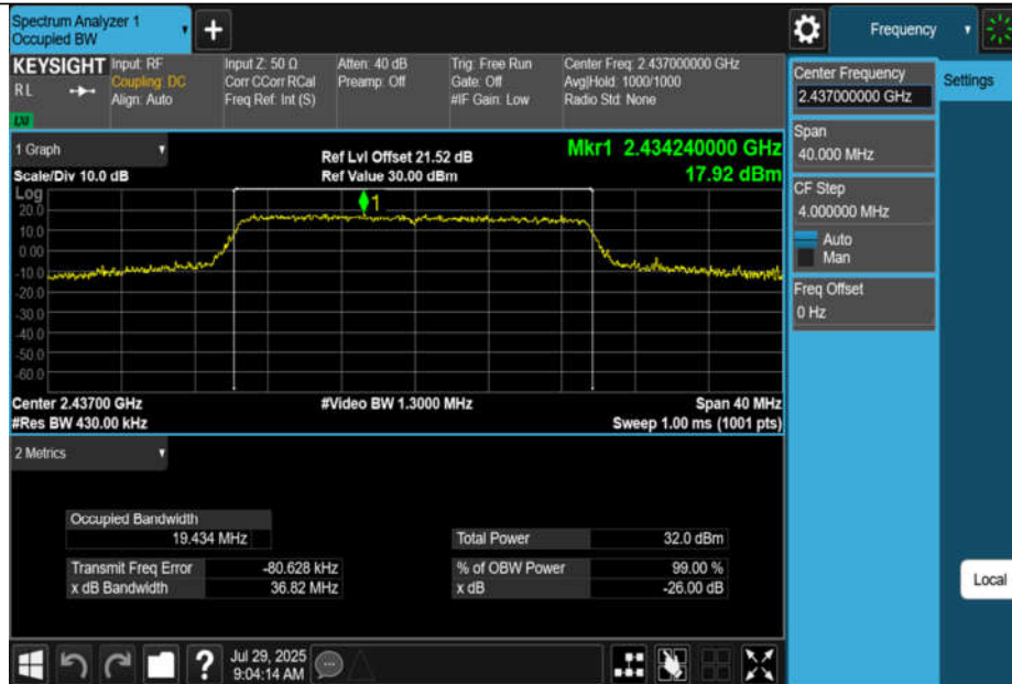
11BE20MIMO-Ant1-2437
