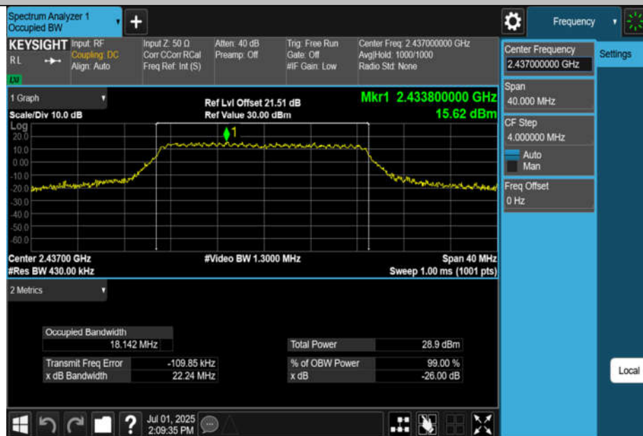
11N20MIMO-Ant2-2437
