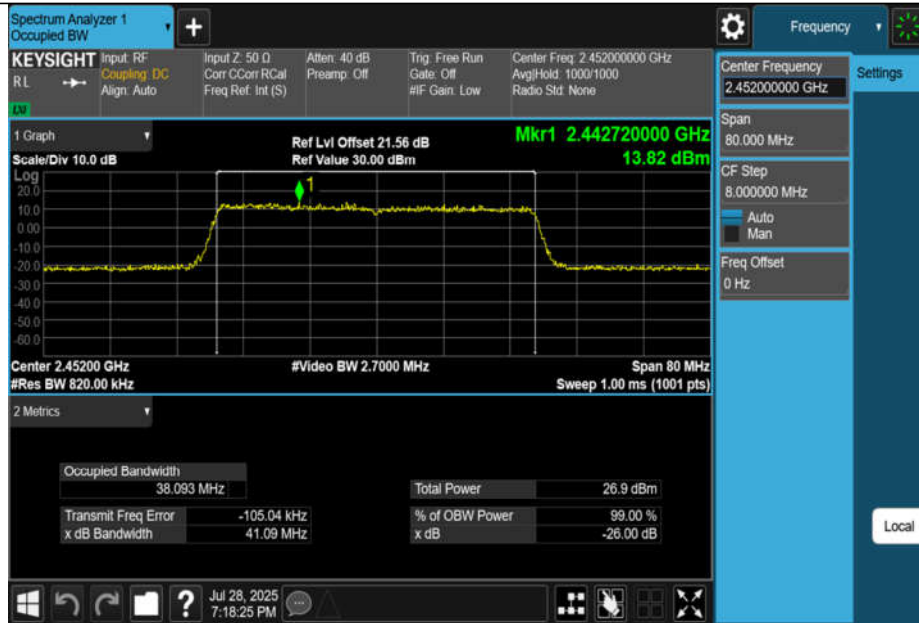
11AX40MIMO-Ant1-2452
