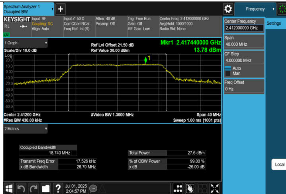
11N20MIMO-Ant1-2412
