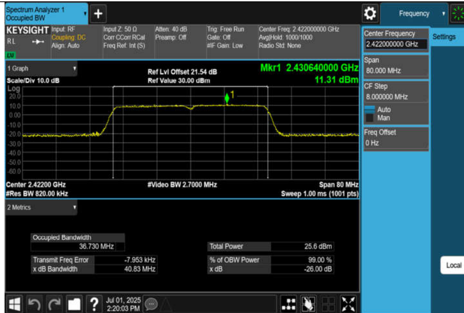
11N40MIMO-Ant1-2422
