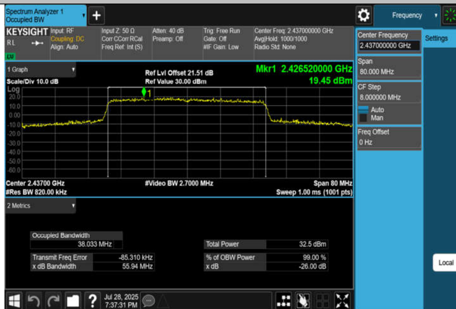
11AX40MIMO-Ant2-2437
