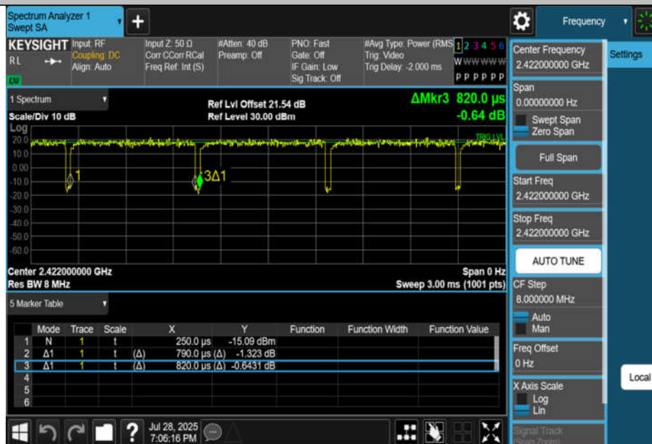
NTNV-11AX40MIMO-Ant1-2422
