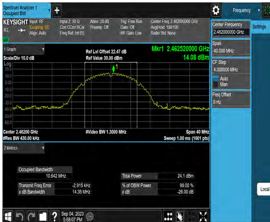
11B_Ant2_2462
