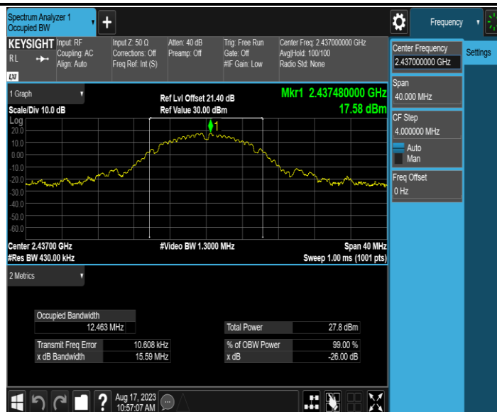
11B-MIMO_Ant2_2437
