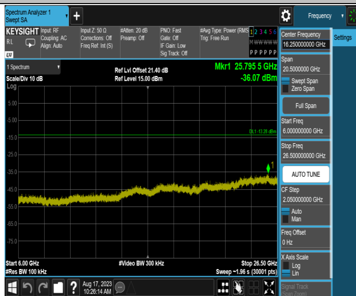
11AX40MIMO_Ant2_2452_0~Reference
