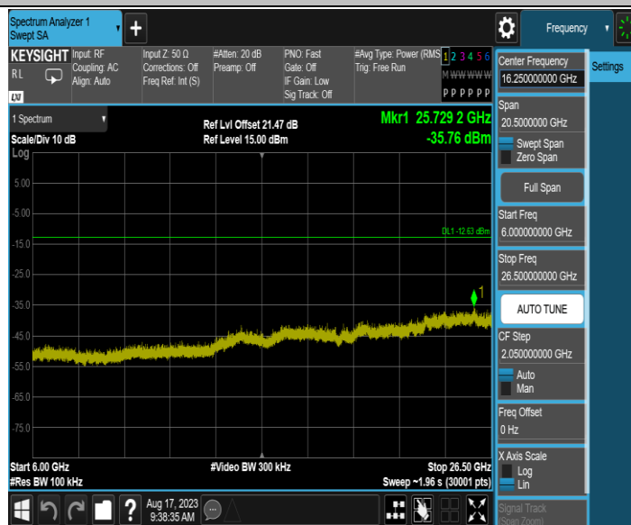
11N40MIMO_Ant2_2422_0~Reference
