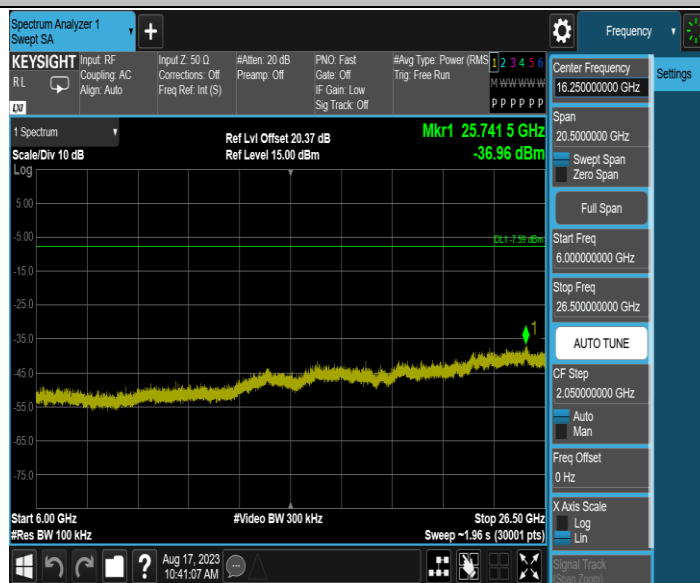
11AX20MIMO_Ant1_2462_0~Reference
