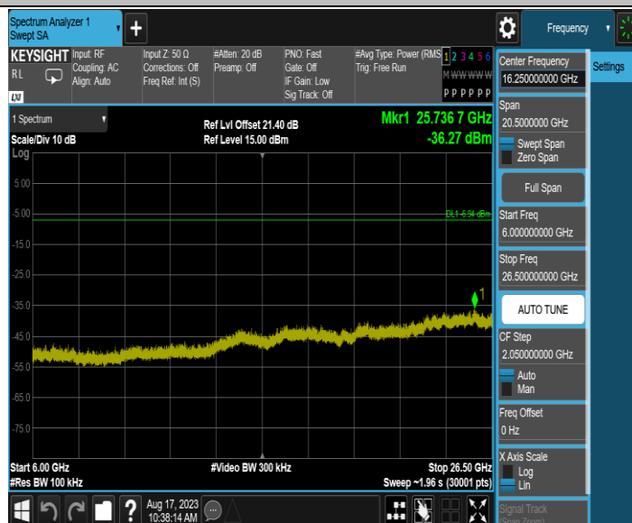
11AX20MIMO_Ant2_2437_0~Reference
