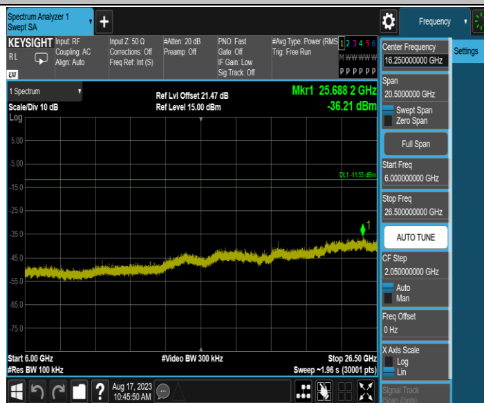
11AX20MIMO_Ant2_2412_0~Reference
