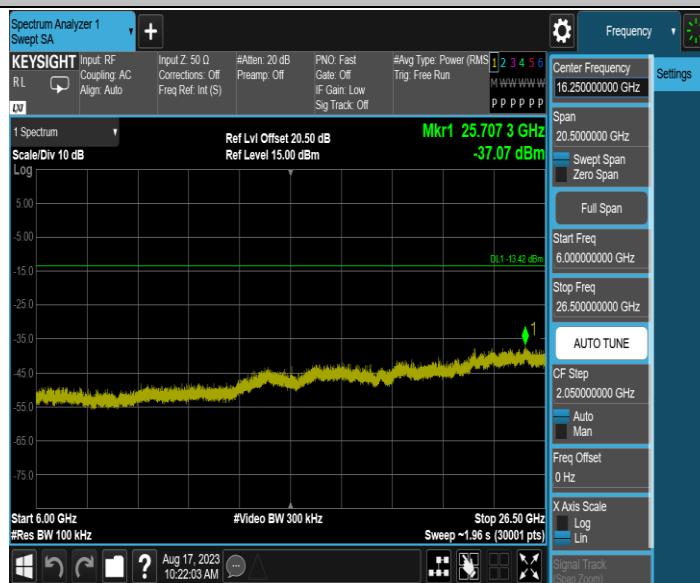
11AX40MIMO_Ant1_2437_0~Reference
