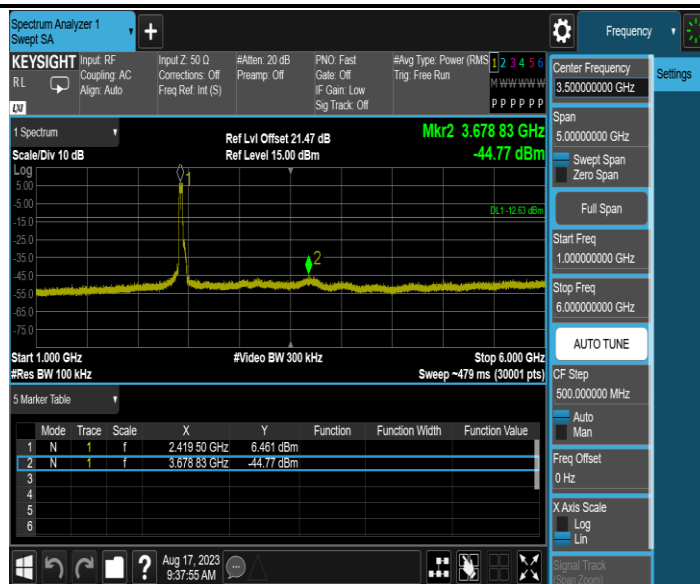
11N40MIMO_Ant1_2422_6000~26500
