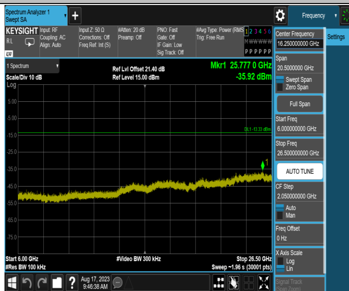
11N40MIMO_Ant2_2452_0~Reference
