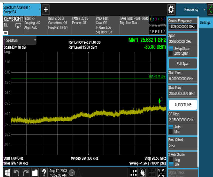
11AX20MIMO_Ant2_2462_0~Reference
