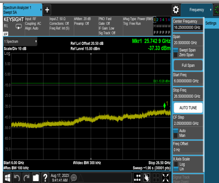
11N40MIMO_Ant1_2437_0~Reference
