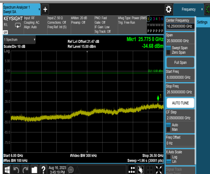
11B-MIMO_Ant2_2412_0~Reference
