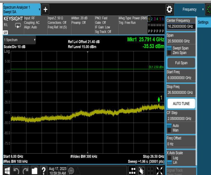
11B-MIMO_Ant2_2437_0~Reference
