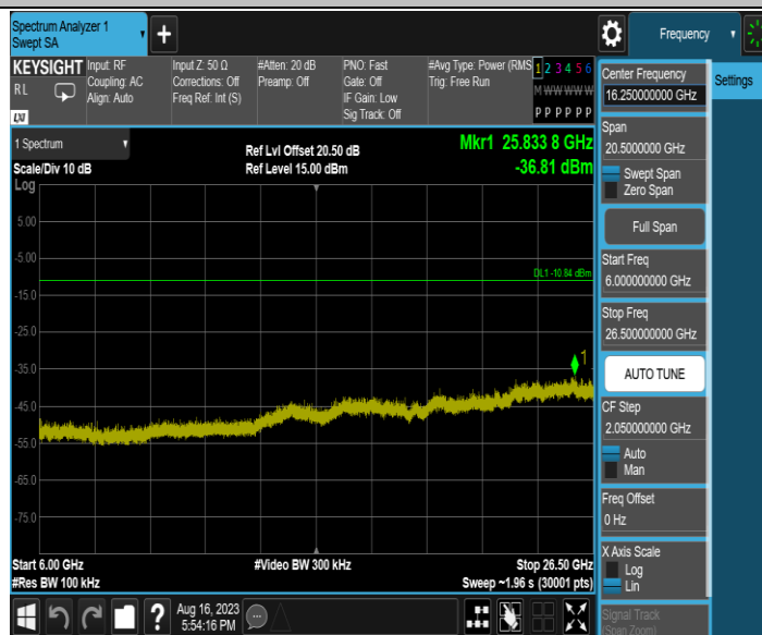
11N20MIMO_Ant1_2437_0~Reference
