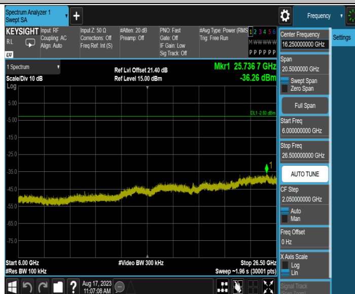
11B-MIMO_Ant2_2462_0~Reference
