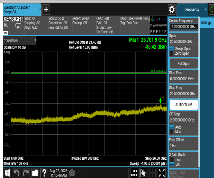
11N20MIMO_Ant2_2437_0~Reference
