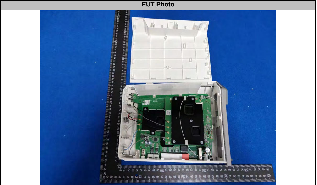
EUT Photo
