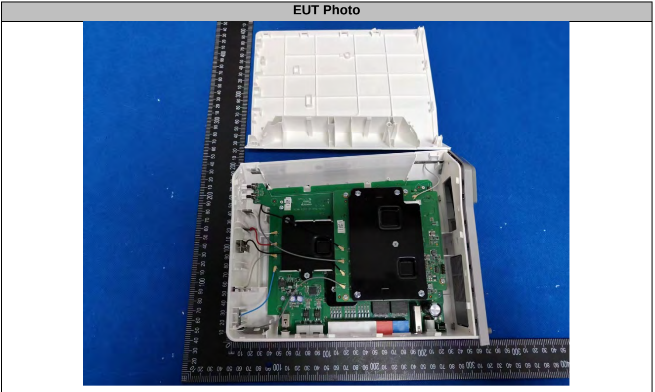
EUT Photo
