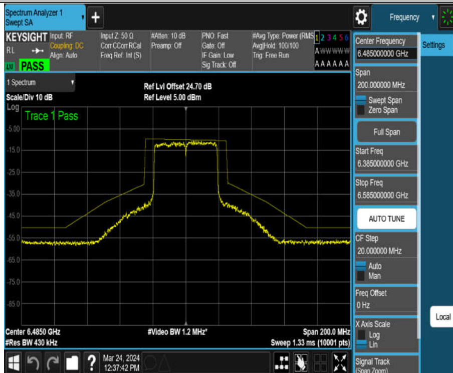
11AX40MIMO_Ant4_6485
