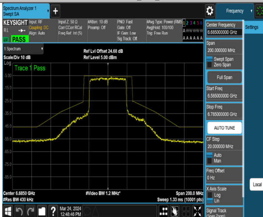
11AX40MIMO_Ant2_6685
