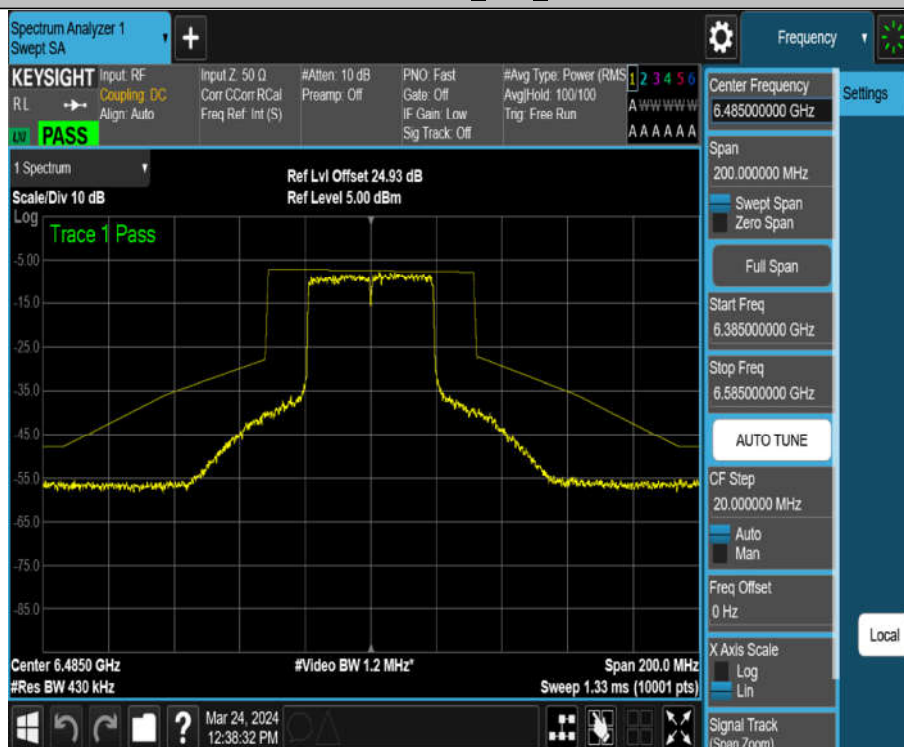
11AX40MIMO_Ant4_6485
