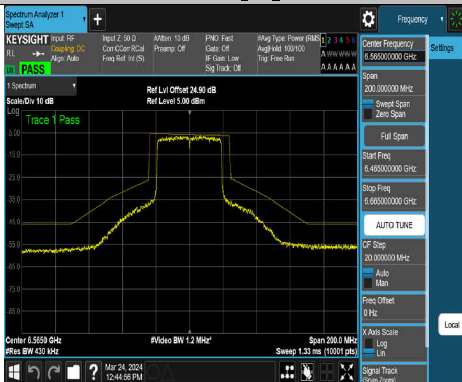
11AX40MIMO_Ant2_6565
