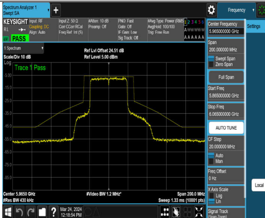
11AX40MIMO_Ant2_5965
