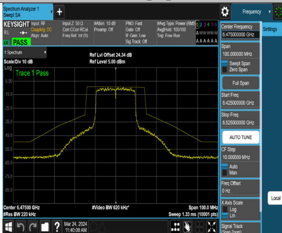
11AX20MIMO_Ant2_6475
