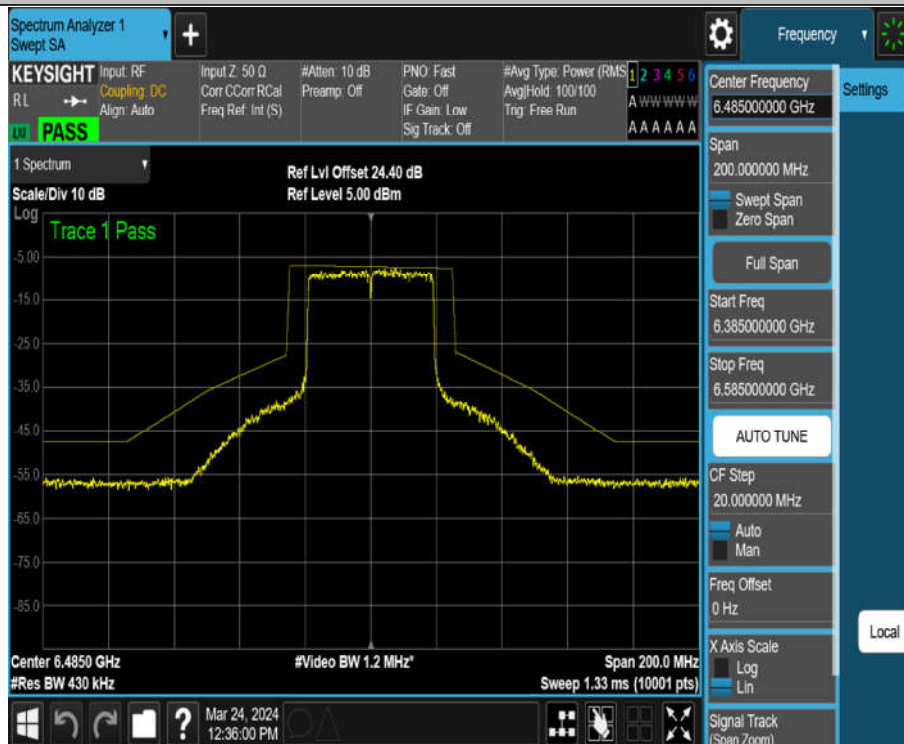
11AX40MIMO_Ant2_6485
