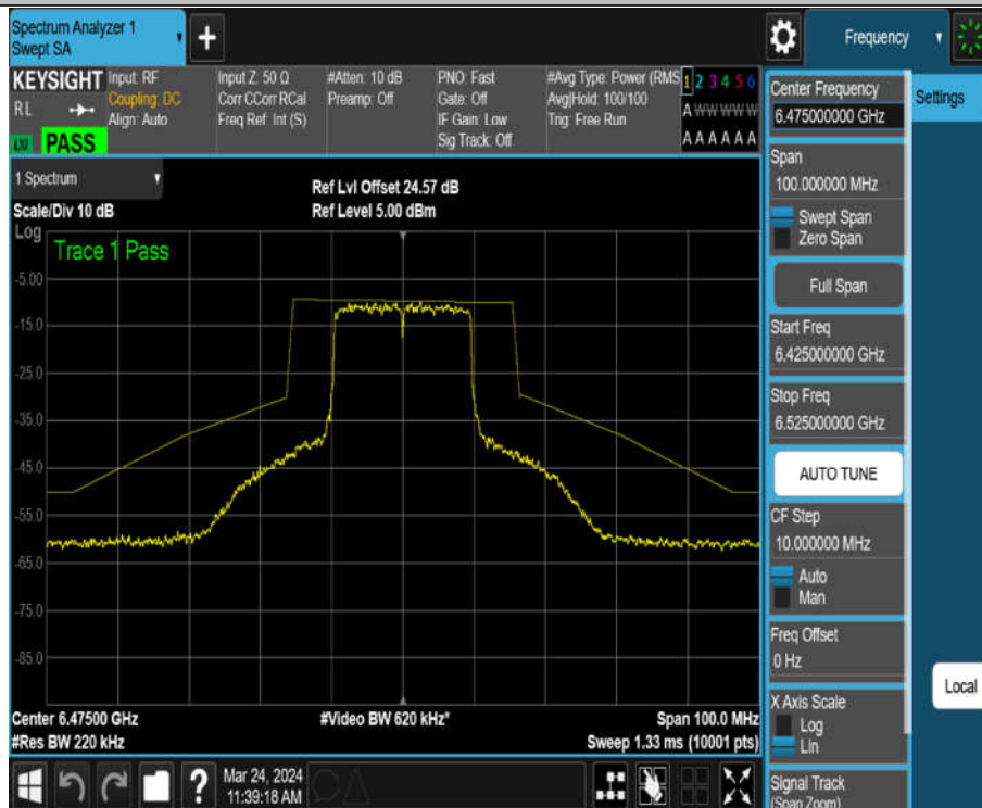
11AX20MIMO_Ant2_6475
