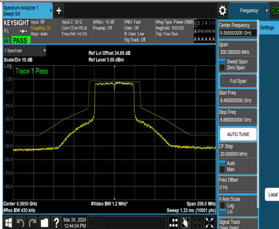
11AX40MIMO_Ant2_6565
