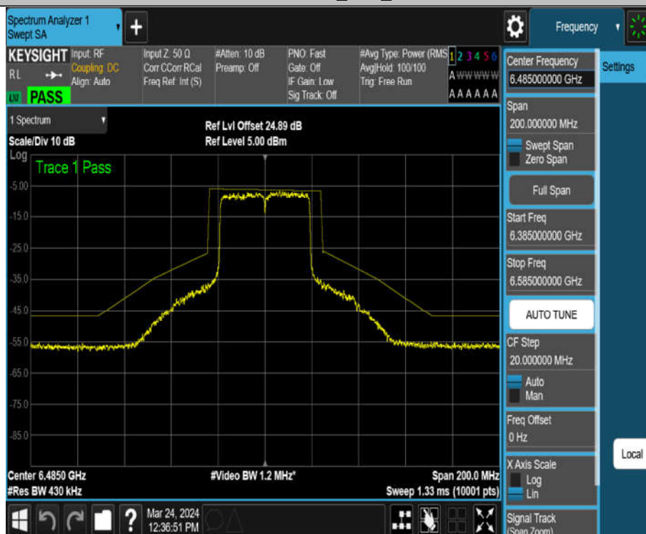
11AX40MIMO_Ant2_6485
