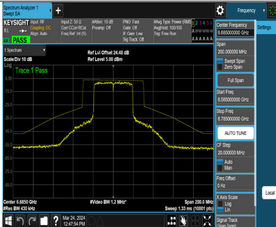
11AX40MIMO_Ant2_6685
