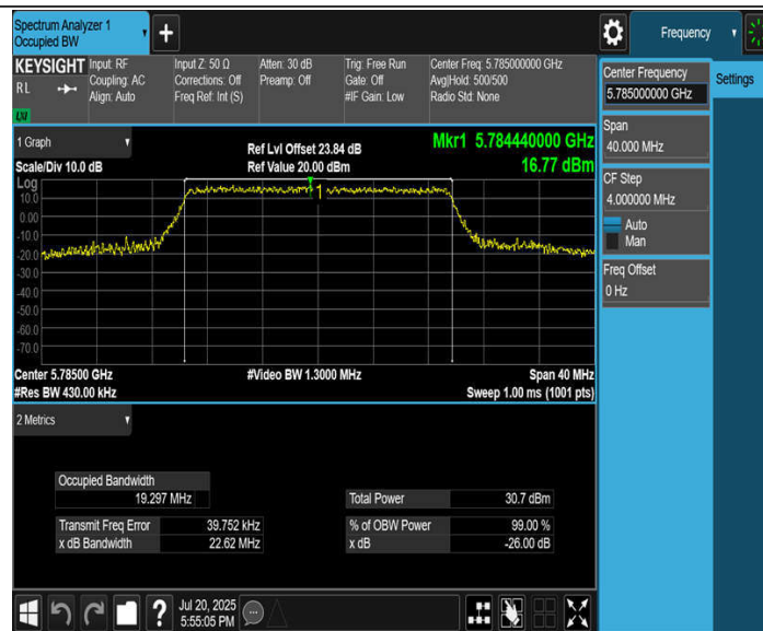
11BE20MIMO_Ant4_5785
