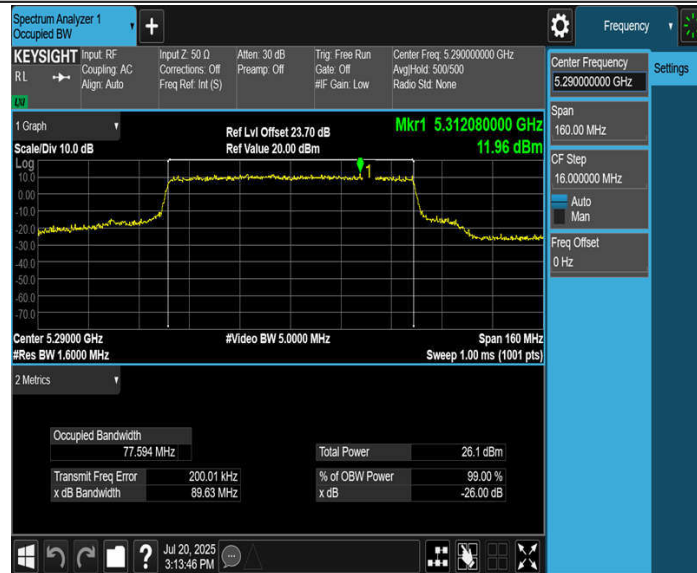
11BE80MIMO_Ant3_5290
