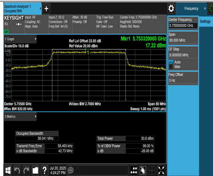
11BE40MIMO_Ant4_5755
