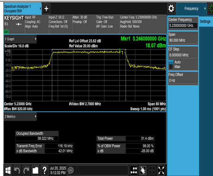
11BE40MIMO_Ant2_5230
