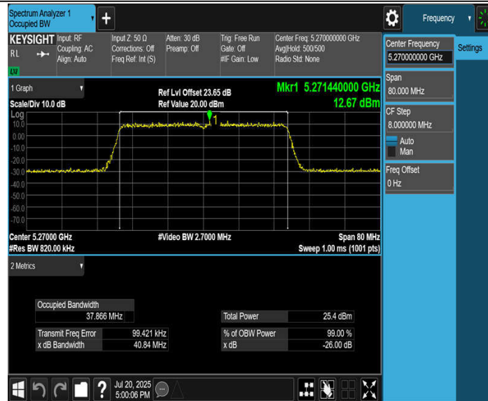
11BE40MIMO_Ant3_5270
