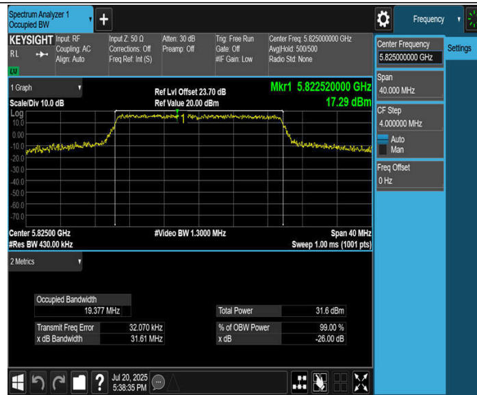
11BE20MIMO_Ant2_5825
