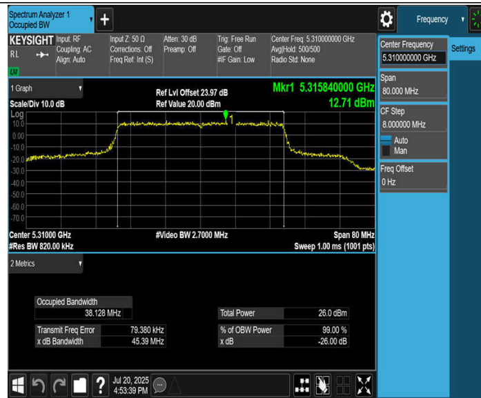
11BE40MIMO_Ant4_5310
