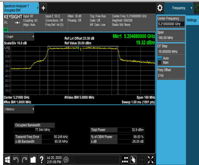
11BE80MIMO_Ant4_5210
