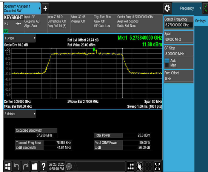
11BE40MIMO_Ant2_5270
