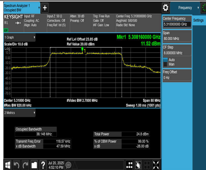
11BE40MIMO_Ant3_5310
