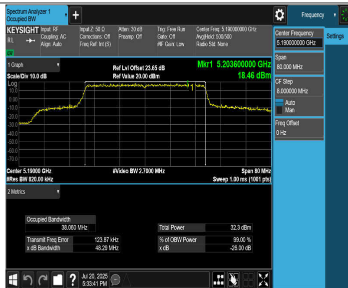
11BE40MIMO_Ant4_5190
