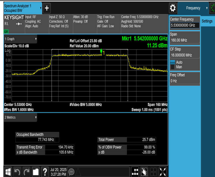
11BE80MIMO_Ant3_5530
