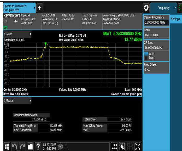
11BE80MIMO_Ant4_5290
