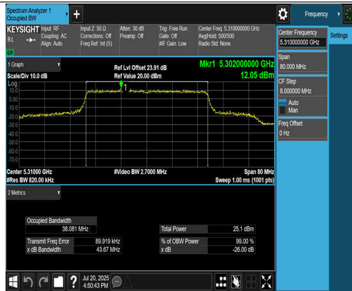
11BE40MIMO_Ant2_5310
