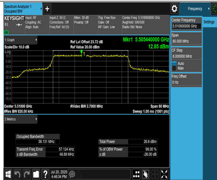
11BE40MIMO_Ant4_5510
