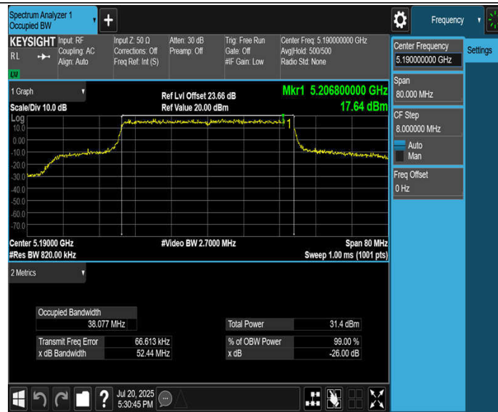
11BE40MIMO_Ant2_5190
