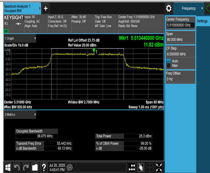
11BE40MIMO_Ant2_5510
