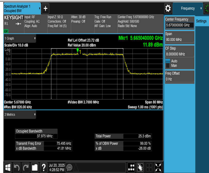
11BE40MIMO_Ant2_5670
