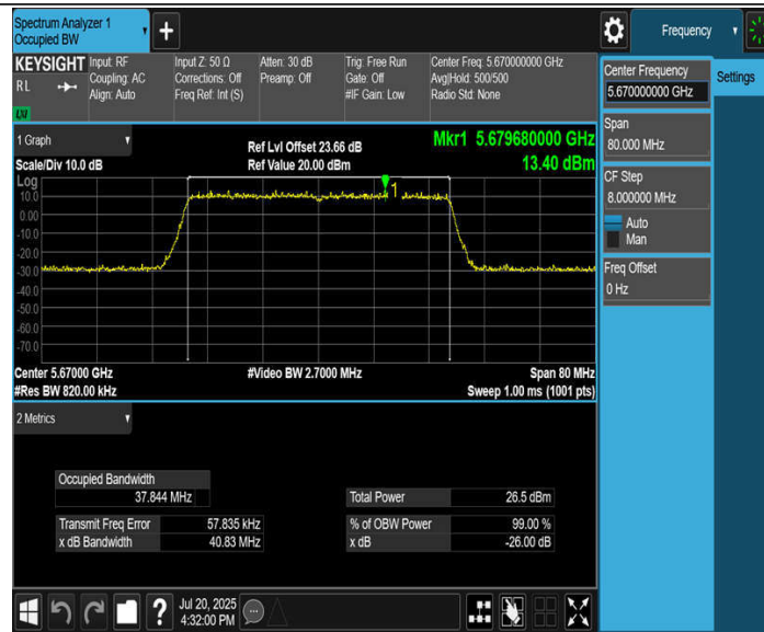
11BE40MIMO_Ant4_5670
