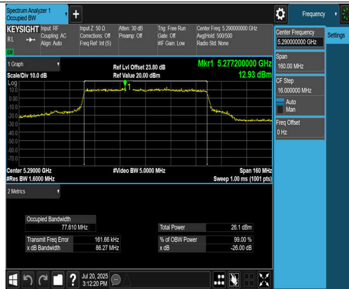
11BE80MIMO_Ant2_5290
