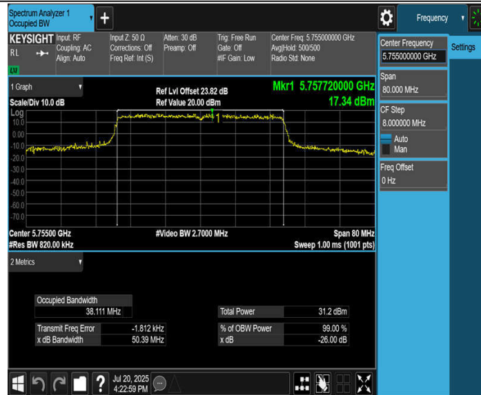
11BE40MIMO_Ant3_5755
