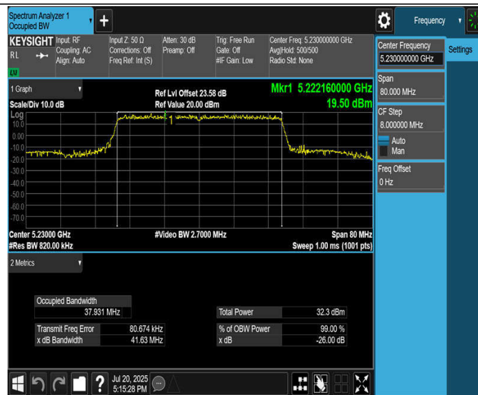
11BE40MIMO_Ant4_5230
