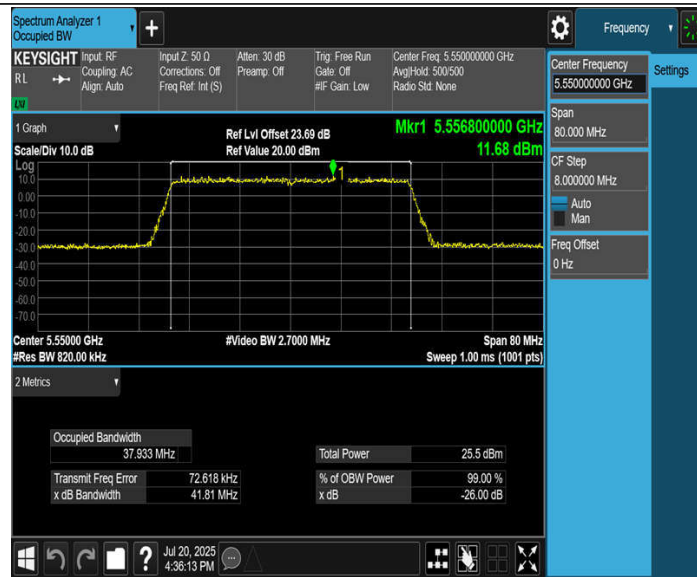
11BE40MIMO_Ant2_5550
