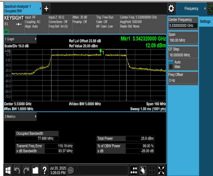
11BE80MIMO_Ant2_5530
