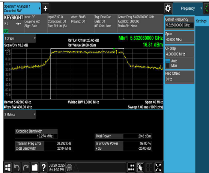
11BE20MIMO_Ant4_5825
