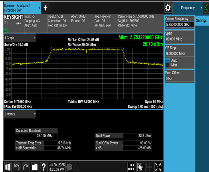
11BE40MIMO_Ant1_5795
