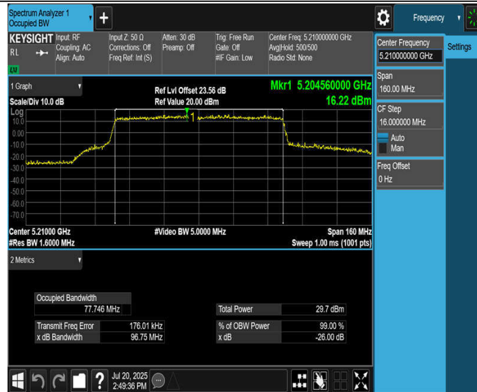
11BE80MIMO_Ant3_5210
