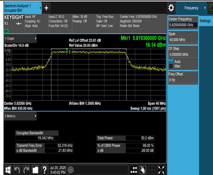
11BE20MIMO_Ant3_5825
