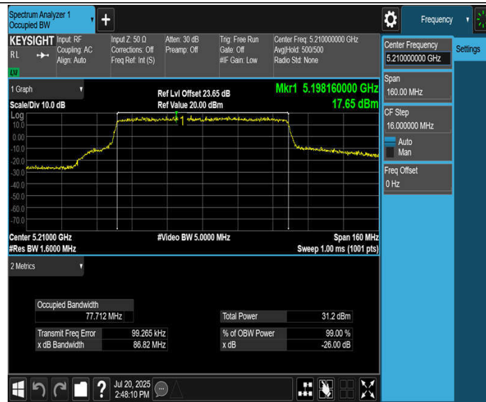
11BE80MIMO_Ant2_5210
