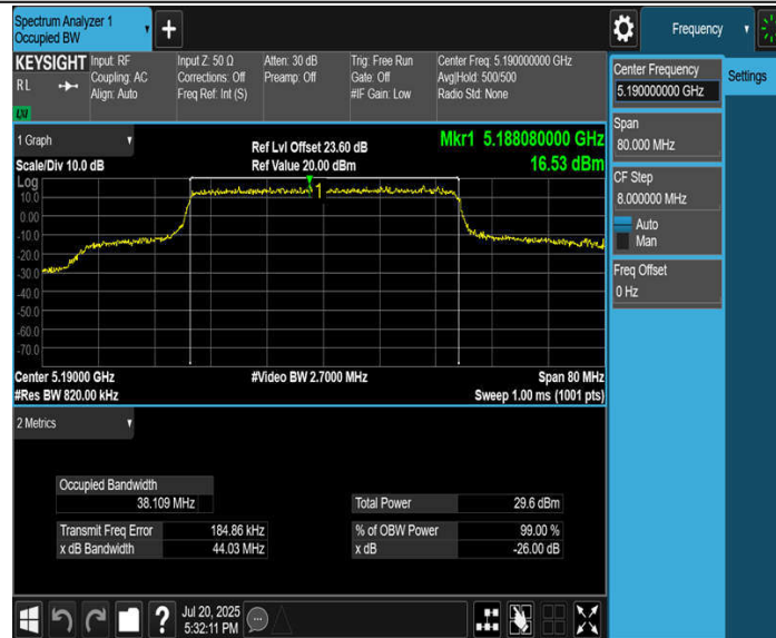
11BE40MIMO_Ant3_5190
