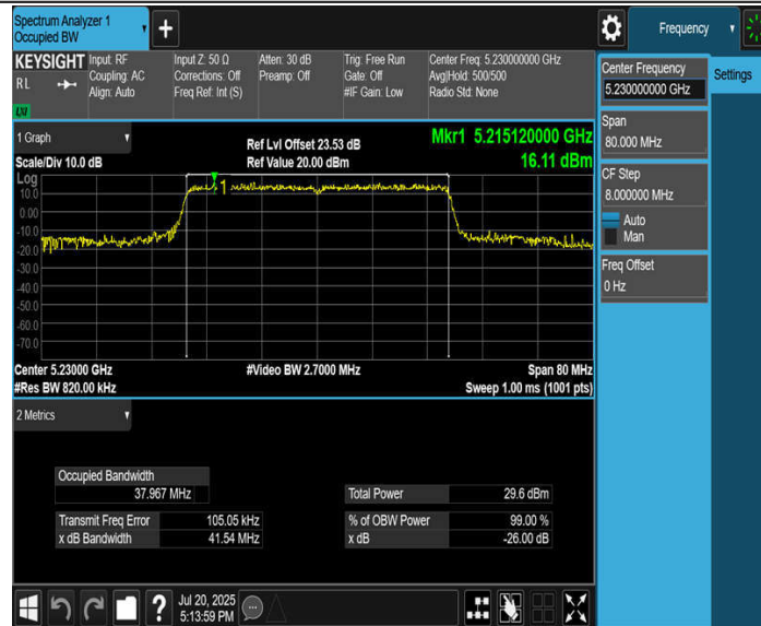
11BE40MIMO_Ant3_5230
