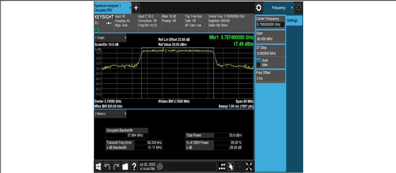
11BE40MIMO_Ant3_5795
