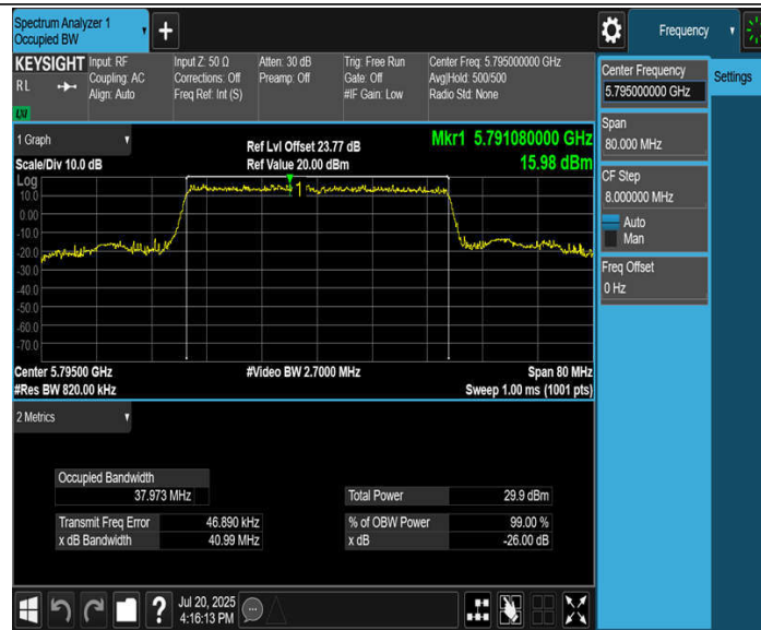
11BE40MIMO_Ant4_5795
