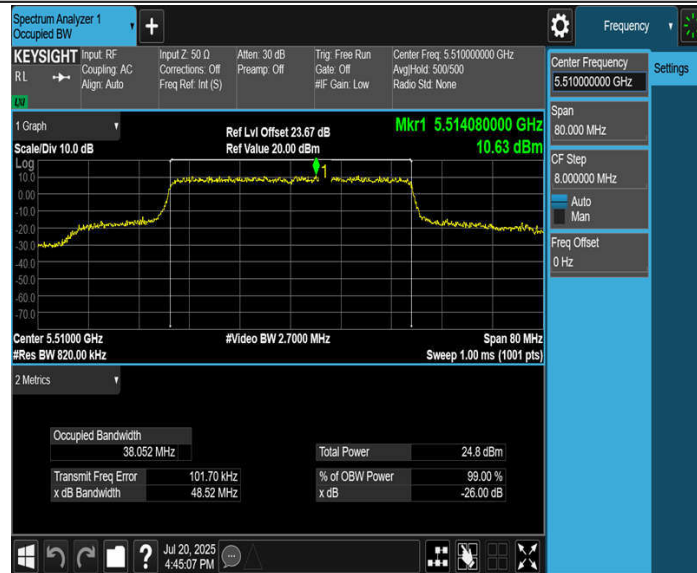
11BE40MIMO_Ant3_5510
