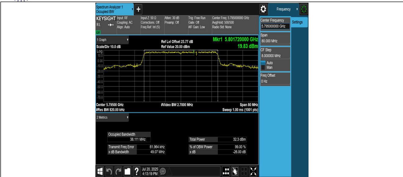
11BE40MIMO_Ant2_5795
