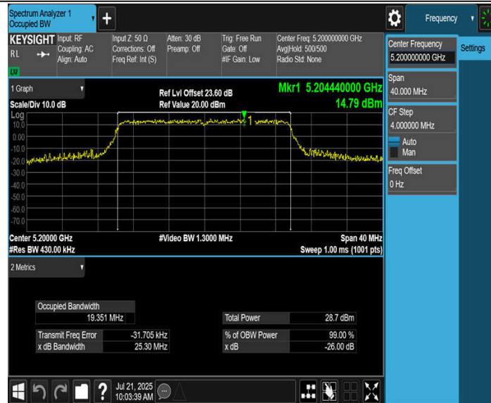
11BE20MIMO_Ant3_5200
