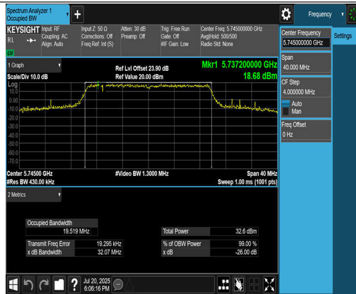
11BE20MIMO_Ant2_5745
