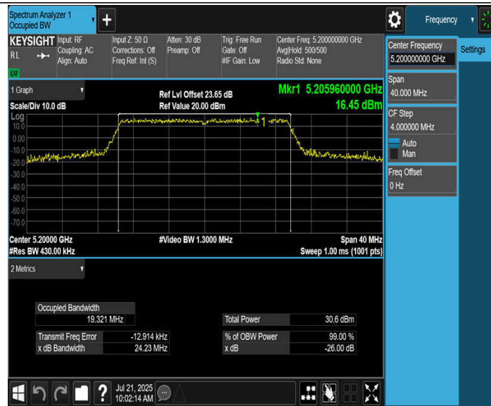
11BE20MIMO_Ant2_5200
