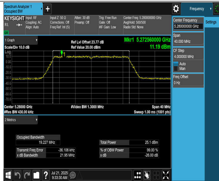
11BE20MIMO_Ant4_5280
