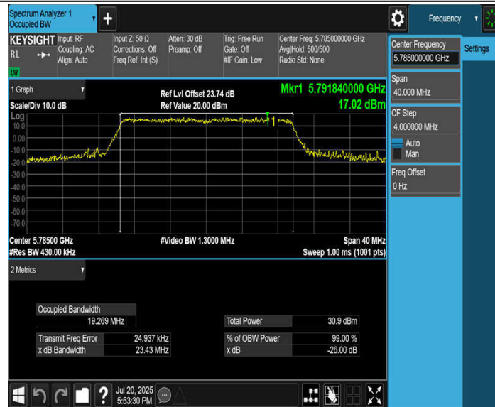
11BE20MIMO_Ant3_5785
