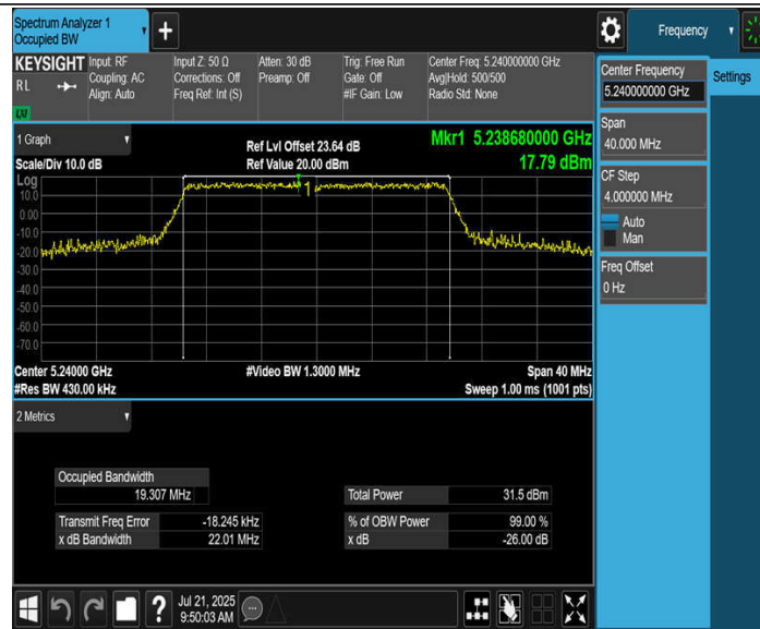
11BE20MIMO_Ant4_5240
