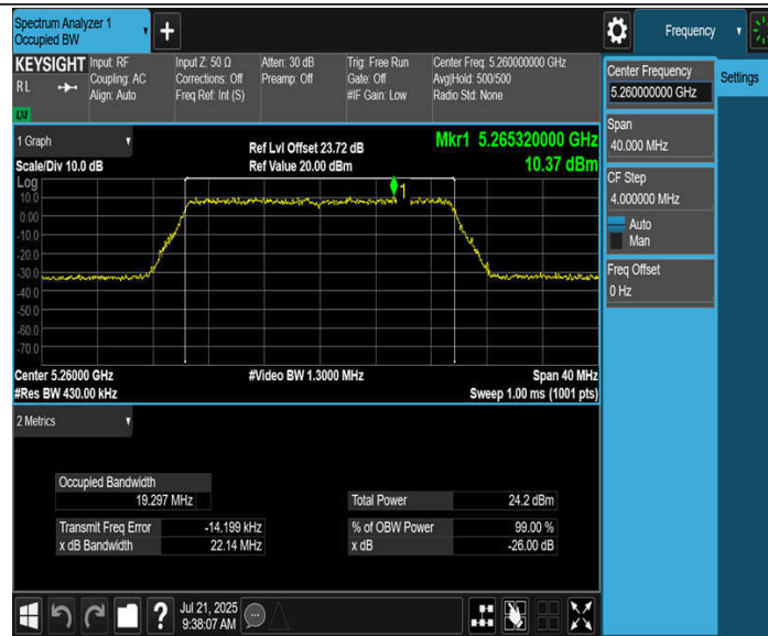
11BE20MIMO_Ant2_5260
