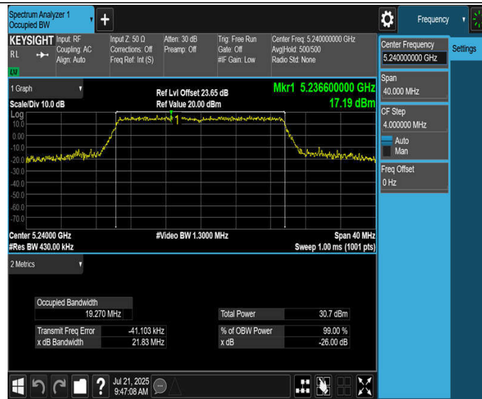
11BE20MIMO_Ant2_5240
