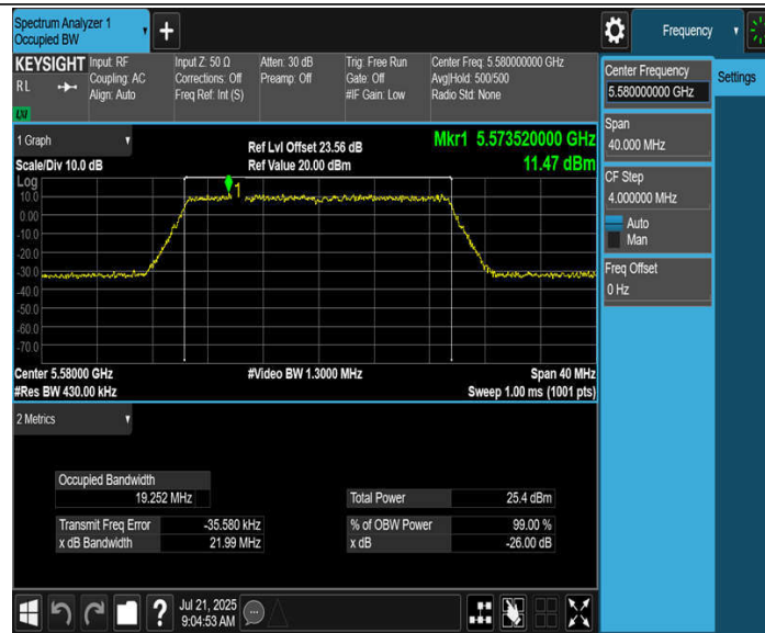
11BE20MIMO_Ant4_5580
