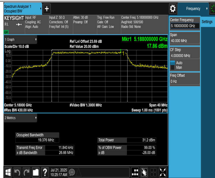
11BE20MIMO_Ant4_5180
