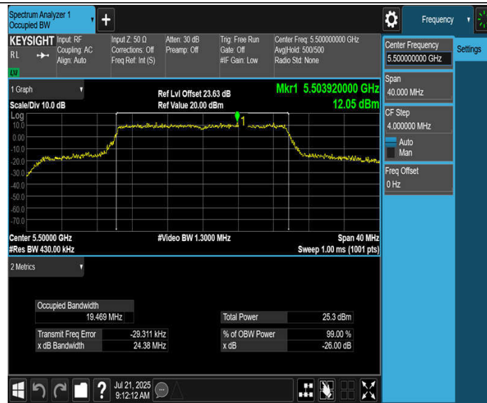
11BE20MIMO_Ant4_5500
