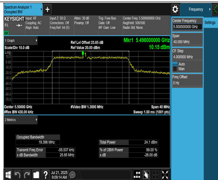
11BE20MIMO_Ant2_5500
