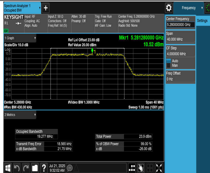
11BE20MIMO_Ant3_5280
