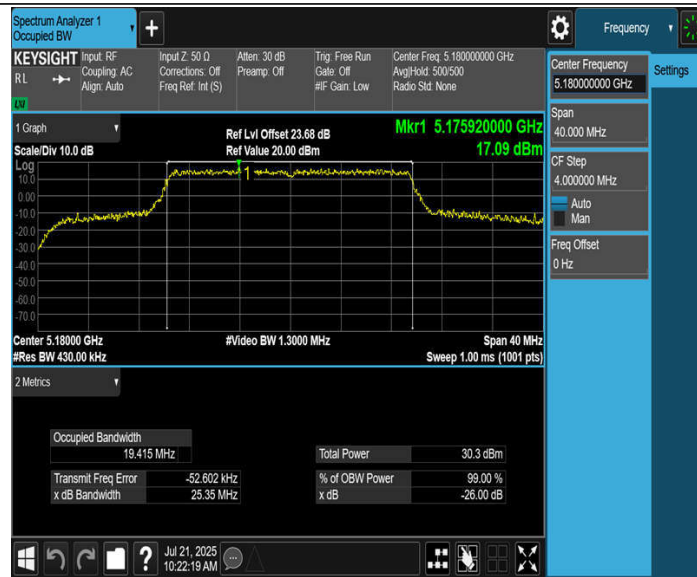
11BE20MIMO_Ant2_5180
