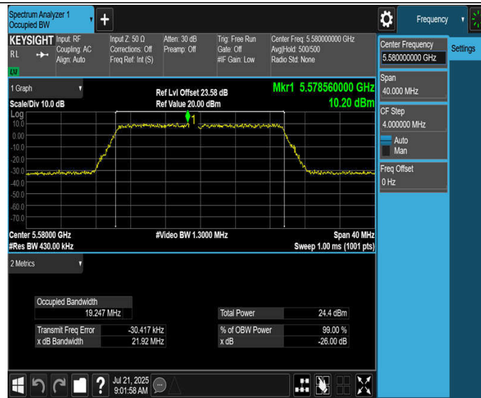
11BE20MIMO_Ant2_5580
