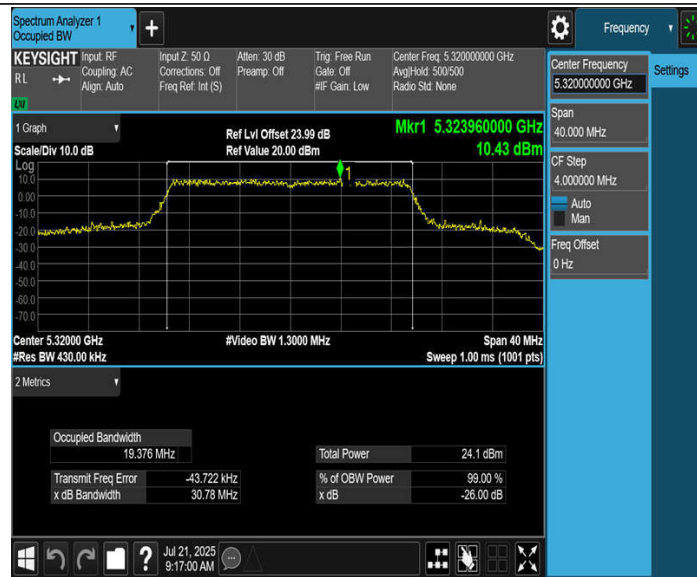
11BE20MIMO_Ant2_5320
