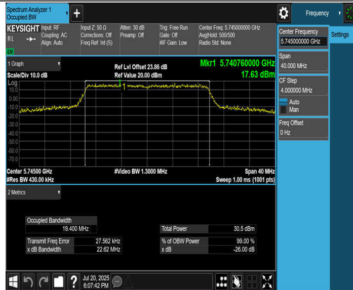
11BE20MIMO_Ant3_5745
