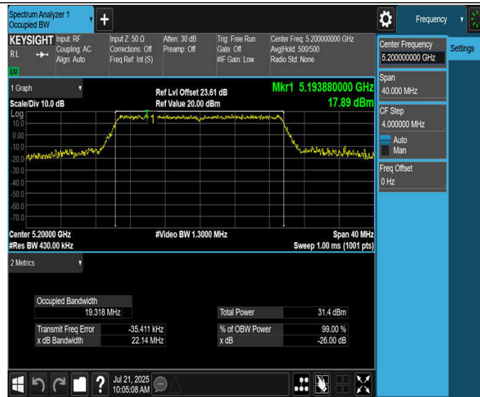
11BE20MIMO_Ant4_5200
