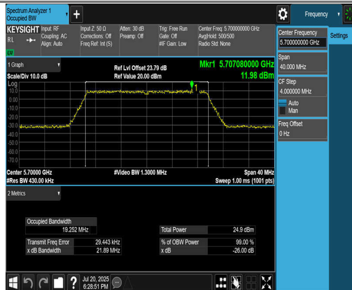
11BE20MIMO_Ant3_5700
