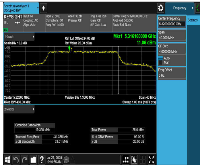
11BE20MIMO_Ant4_5320
