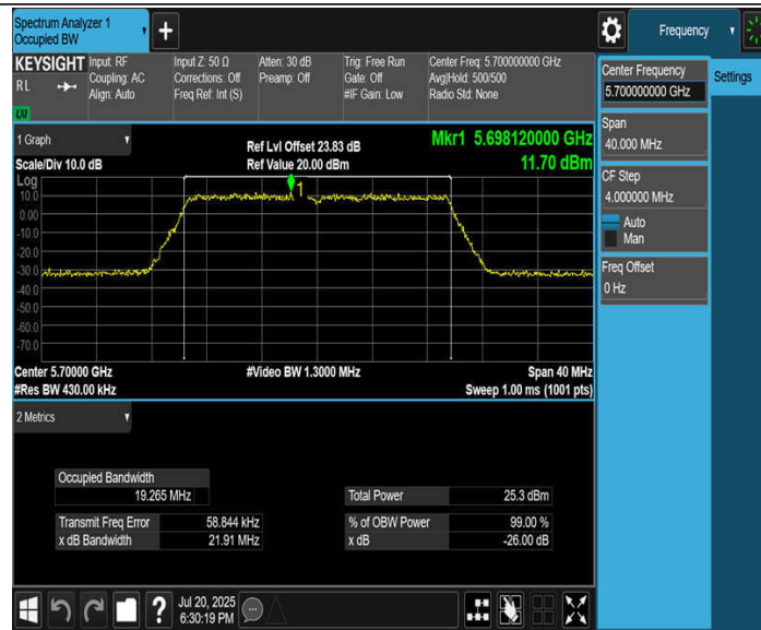
11BE20MIMO_Ant4_5700
