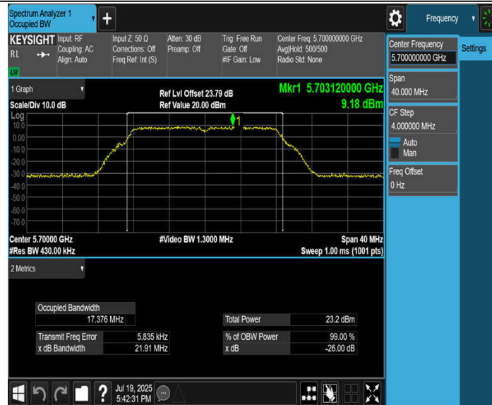
11A-CDD_Ant3_5700
