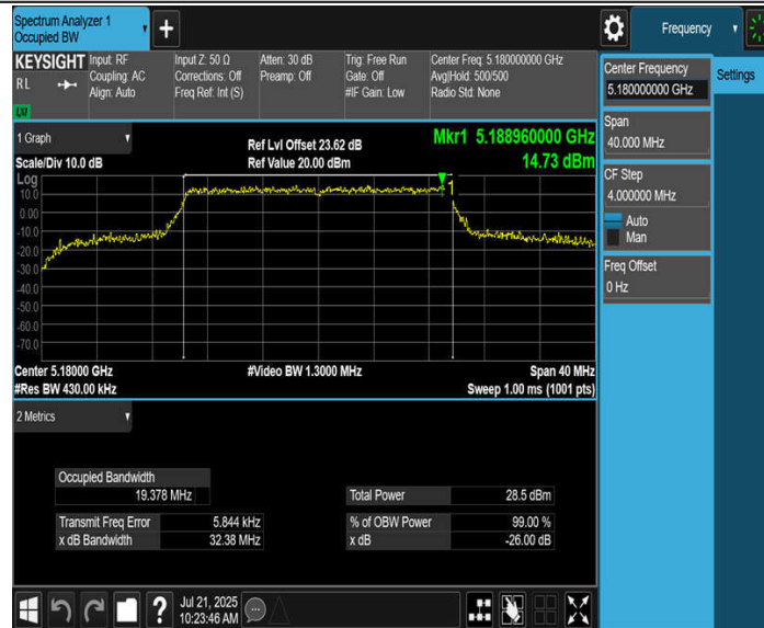
11BE20MIMO_Ant3_5180
