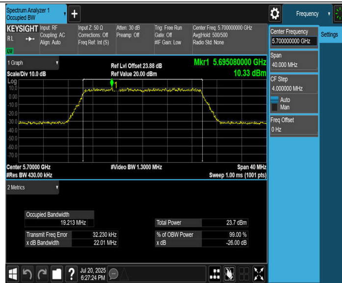
11BE20MIMO_Ant2_5700
