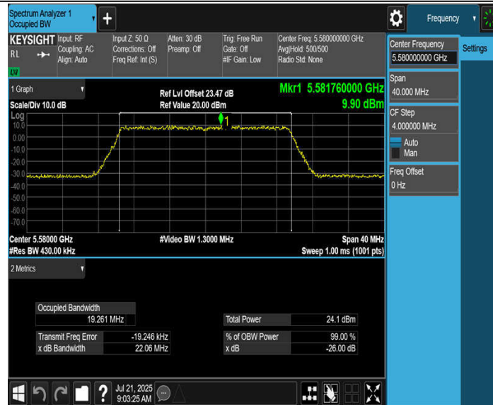
11BE20MIMO_Ant3_5580
