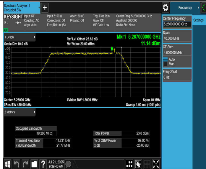
11BE20MIMO_Ant3_5260
