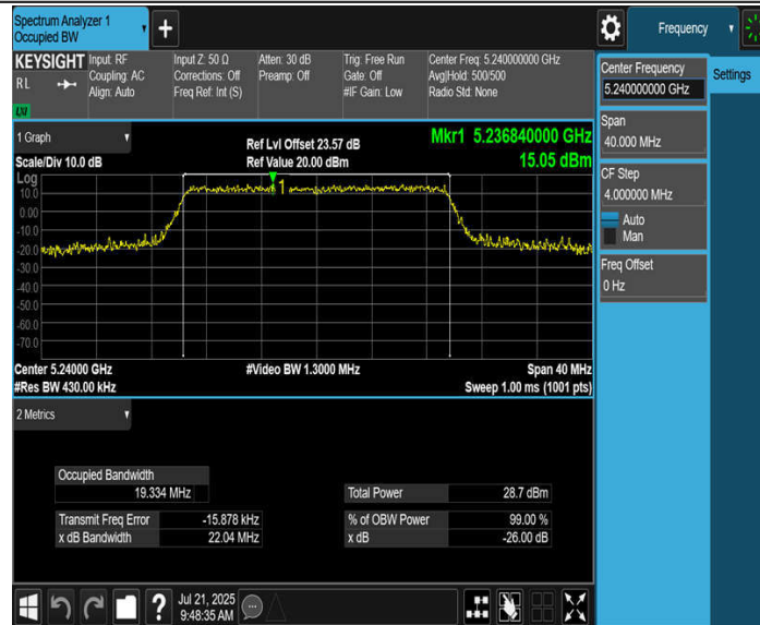
11BE20MIMO_Ant3_5240
