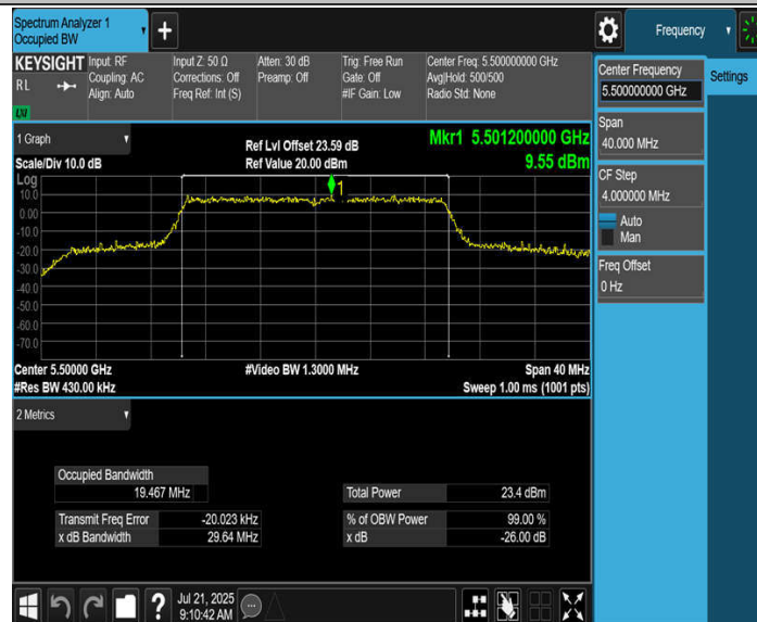
11BE20MIMO_Ant3_5500
