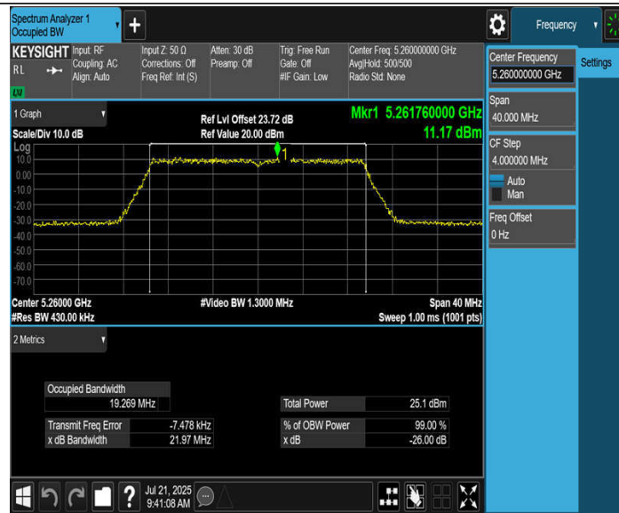
11BE20MIMO_Ant4_5260
