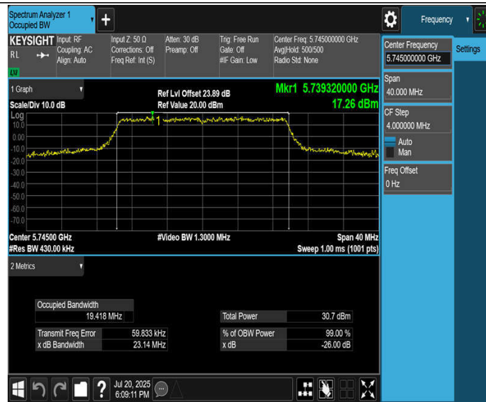
11BE20MIMO_Ant4_5745
