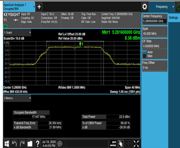
11A-CDD_Ant3_5280
