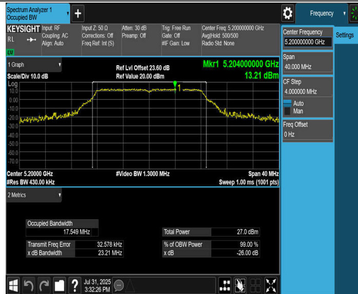
11A-CDD_Ant3_5200
