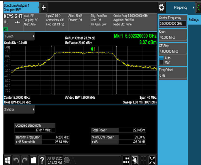
11A-CDD_Ant3_5500
