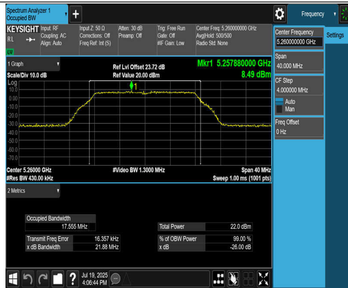
11A-CDD_Ant2_5260
