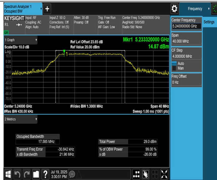
11A-CDD_Ant2_5240
