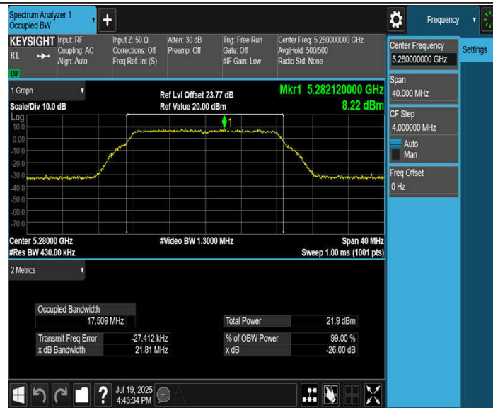
11A-CDD_Ant2_5280
