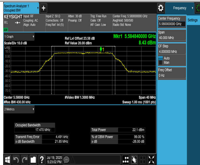
11A-CDD_Ant2_5580
