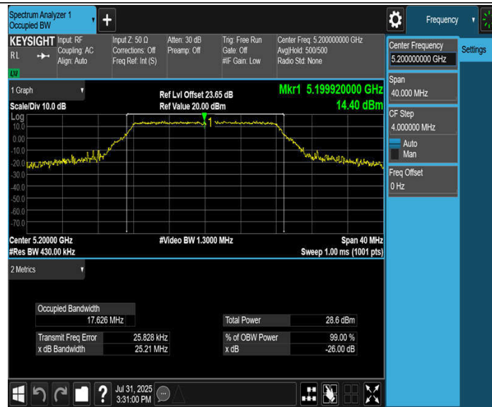
11A-CDD_Ant2_5200
