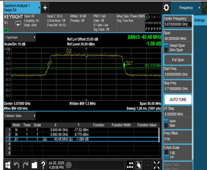
11BE40MIMO_Ant3_5670
