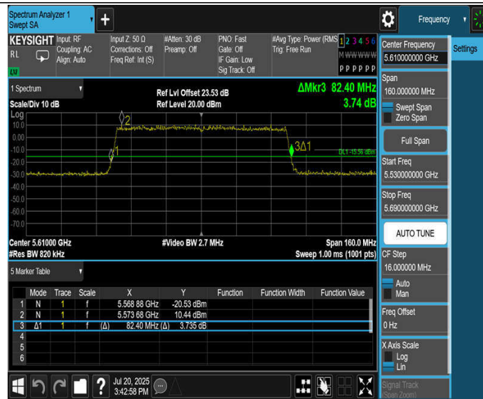
11BE80MIMO_Ant4_5610
