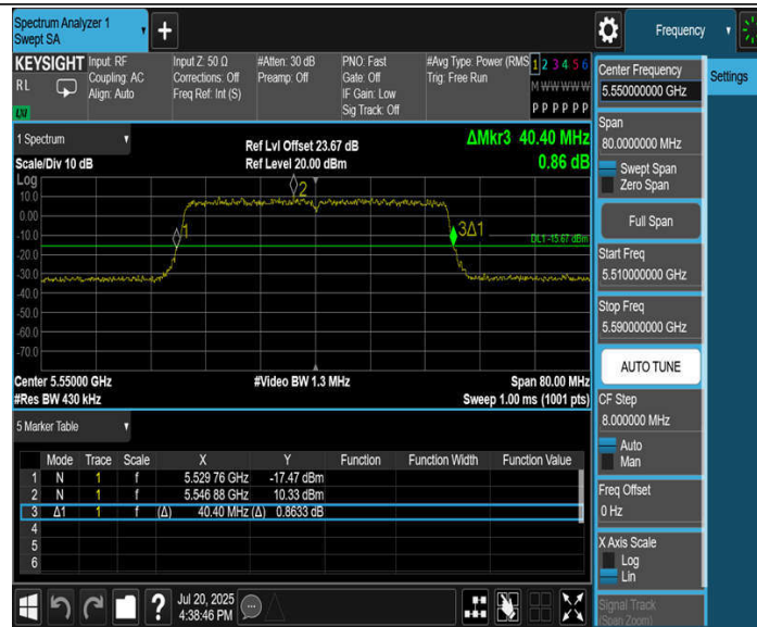
11BE40MIMO_Ant4_5550
