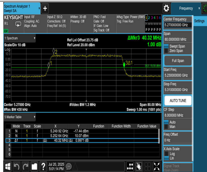
11BE40MIMO_Ant4_5270
