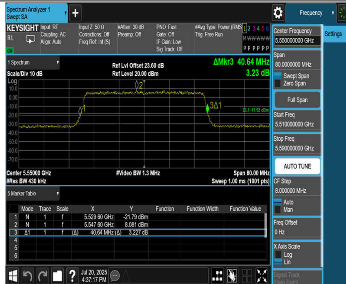
11BE40MIMO_Ant3_5550
