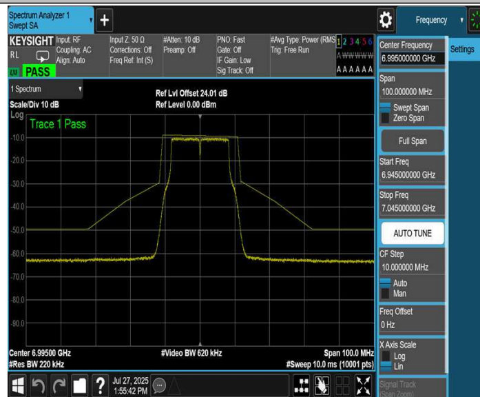
11A-CDD_Ant4_6995
