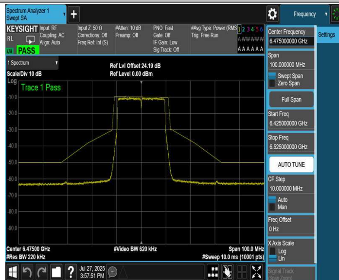
11BE20MIMO_Ant2_6475
