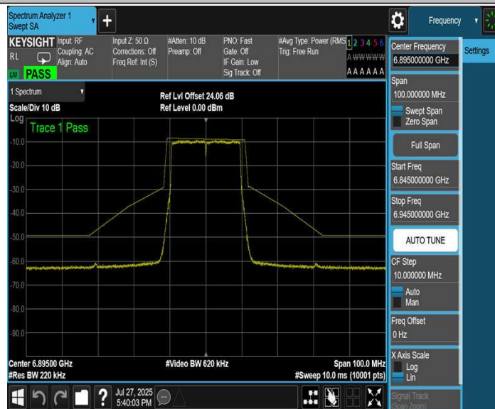
11BE20MIMO_Ant3_6895
