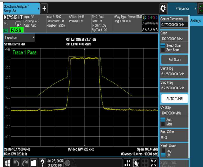
11BE20MIMO_Ant4_6175
