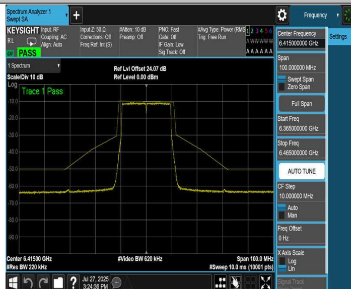
11BE20MIMO_Ant2_6415
