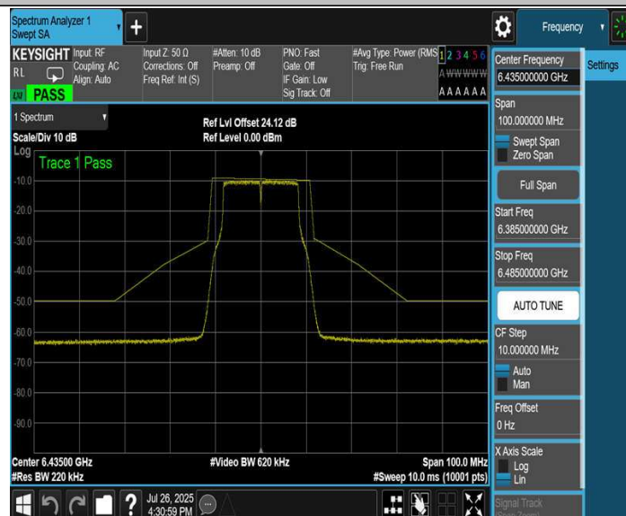
11A-CDD_Ant3_6435
