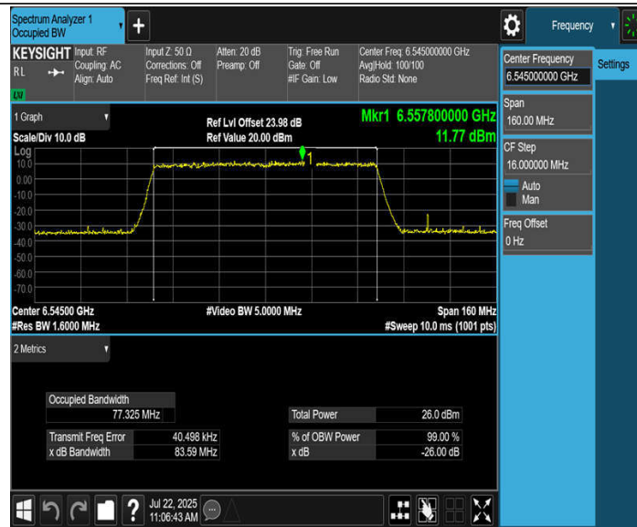
11BE80MIMO_Ant2_6545
