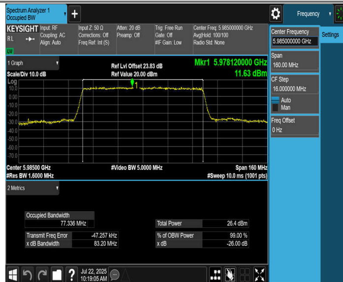
11BE80MIMO_Ant4_5985
