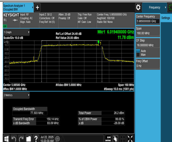
11BE80MIMO_Ant4_5985
