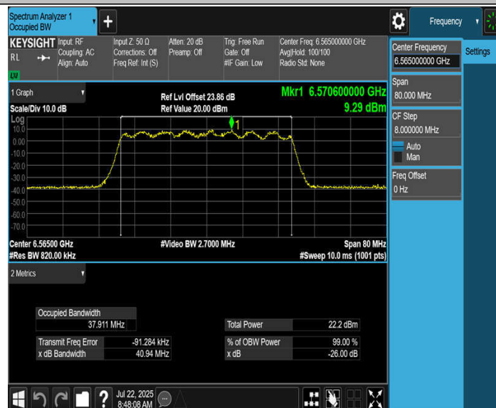
11BE40MIMO_Ant2_6565
