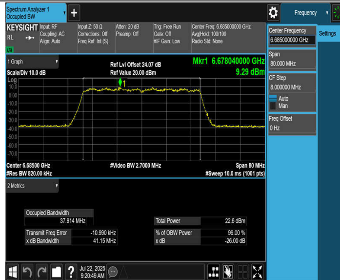
11BE40MIMO_Ant3_6685
