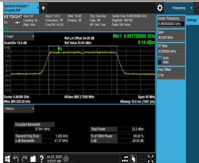
11BE40MIMO_Ant2_6965
