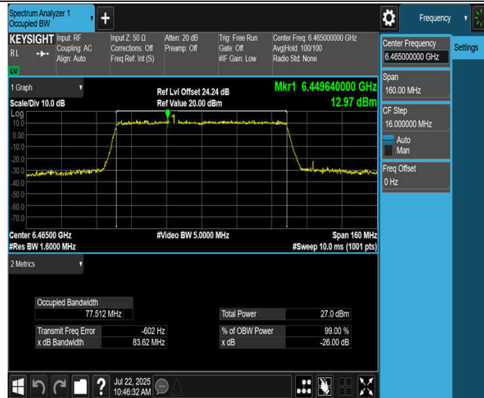
11BE80MIMO_Ant2_6465
