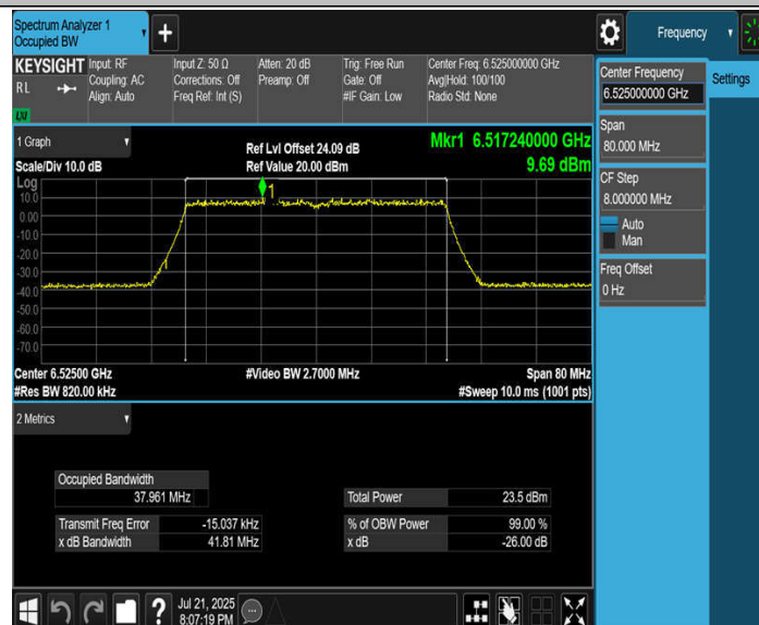
11BE40MIMO_Ant1_6525
