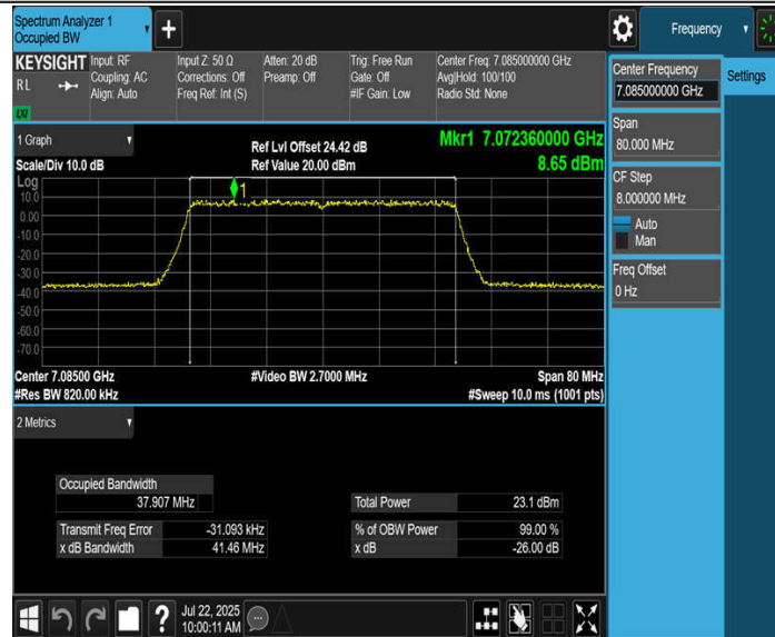
11BE40MIMO_Ant3_7085
