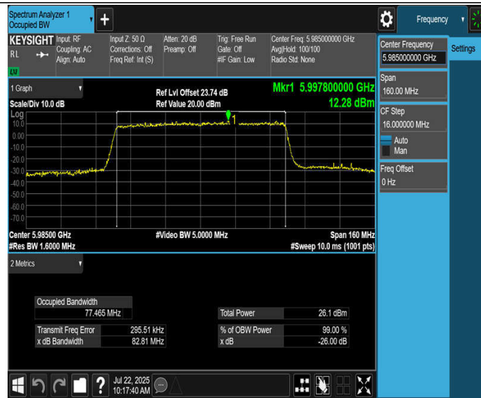
11BE80MIMO_Ant3_5985
