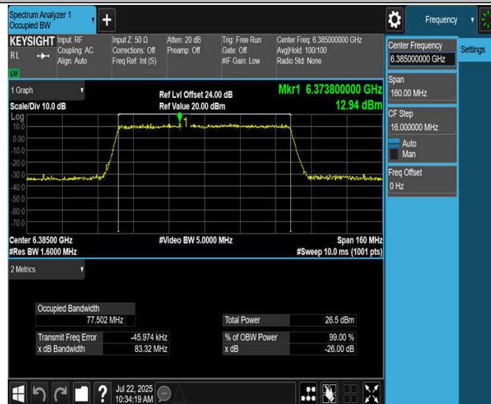
11BE80MIMO_Ant1_6385
