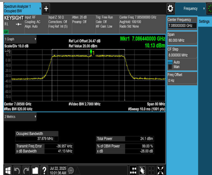
11BE40MIMO_Ant3_7085
