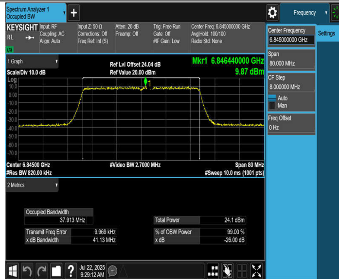
11BE40MIMO_Ant4_6845
