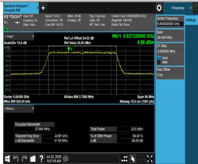
11BE40MIMO_Ant3_6845
