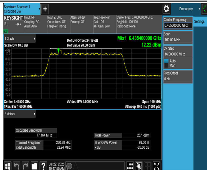
11BE80MIMO_Ant2_6465
