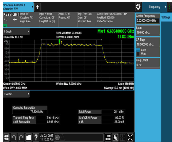
11BE80MIMO_Ant3_6625
