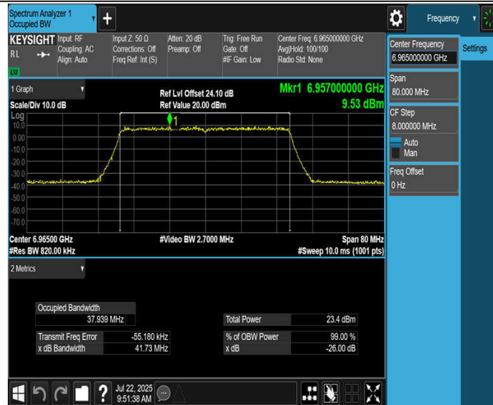
11BE40MIMO_Ant2_6965
