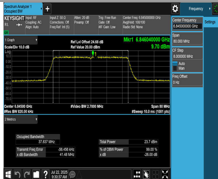
11BE40MIMO_Ant4_6845
