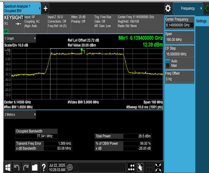
11BE80MIMO_Ant4_6145
