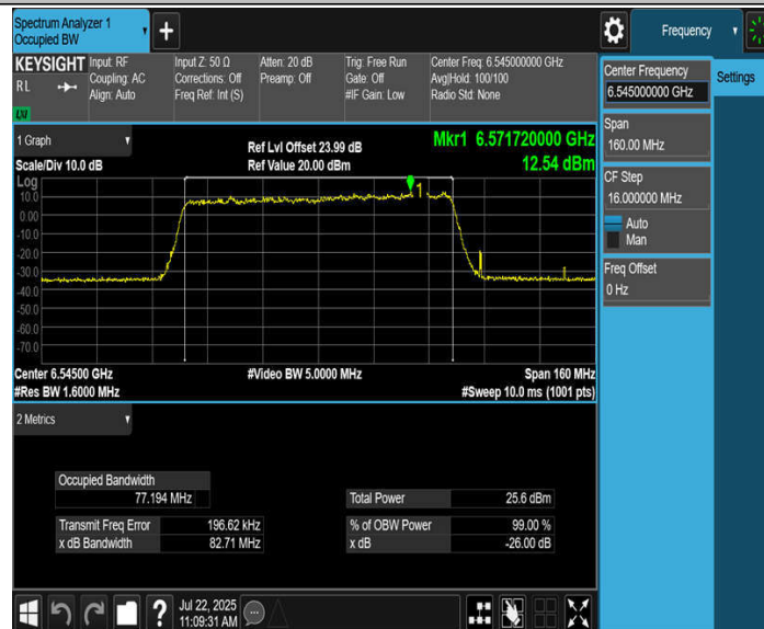
11BE80MIMO_Ant3_6545
