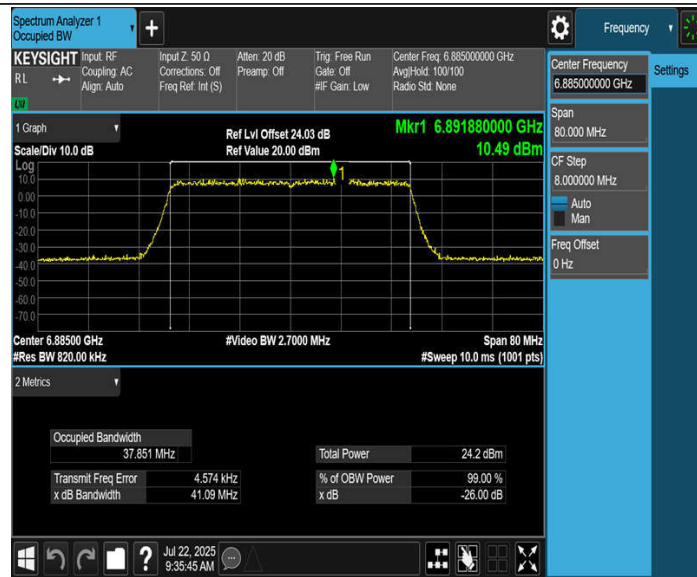
11BE40MIMO_Ant4_6885
