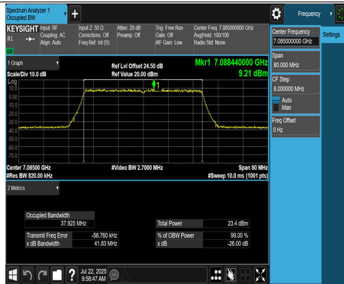
11BE40MIMO_Ant2_7085
