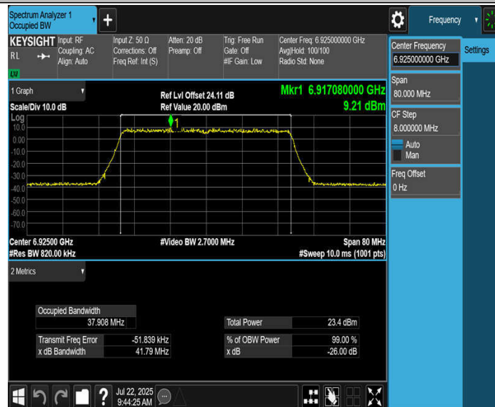
11BE40MIMO_Ant1_6925
