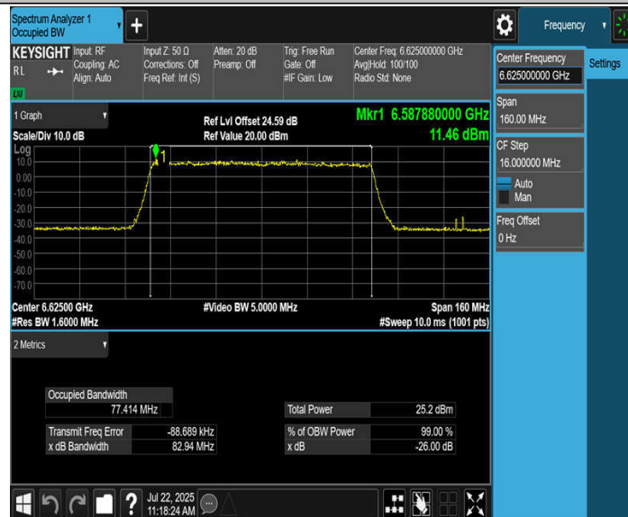
11BE80MIMO_Ant4_6625
