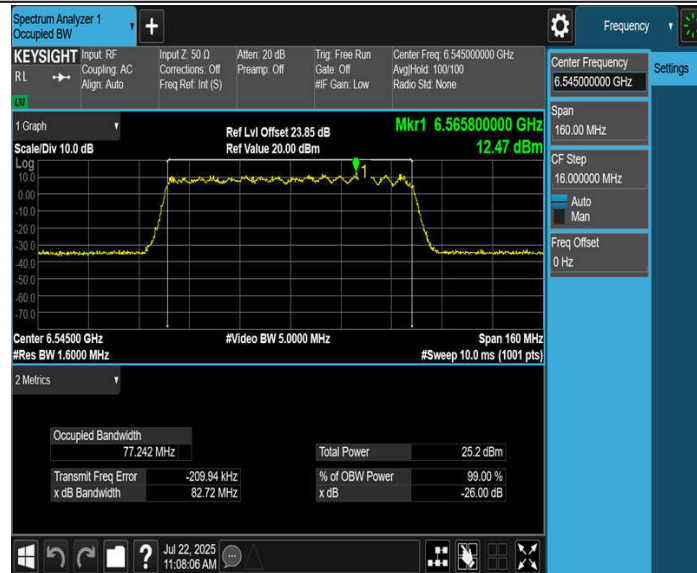
11BE80MIMO_Ant3_6545
