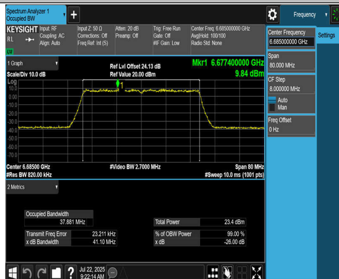
11BE40MIMO_Ant3_6685
