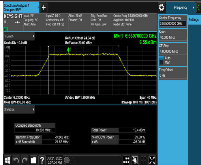
11BE20MIMO_Ant4_6535
