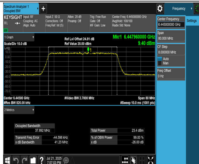
11BE40MIMO_Ant4_6445
