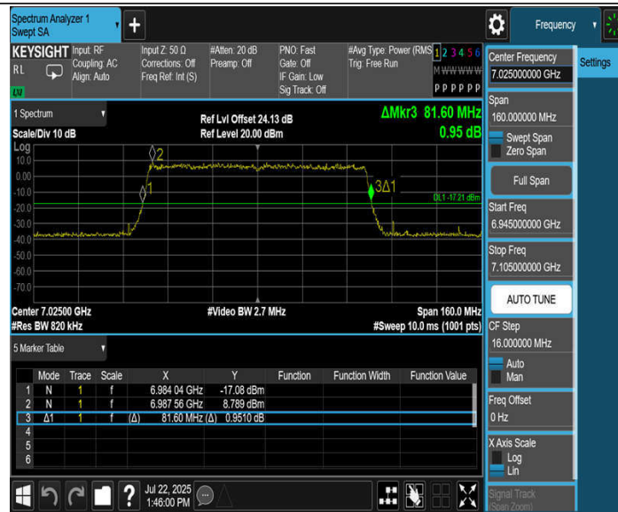
11BE80MIMO_Ant3_7025
