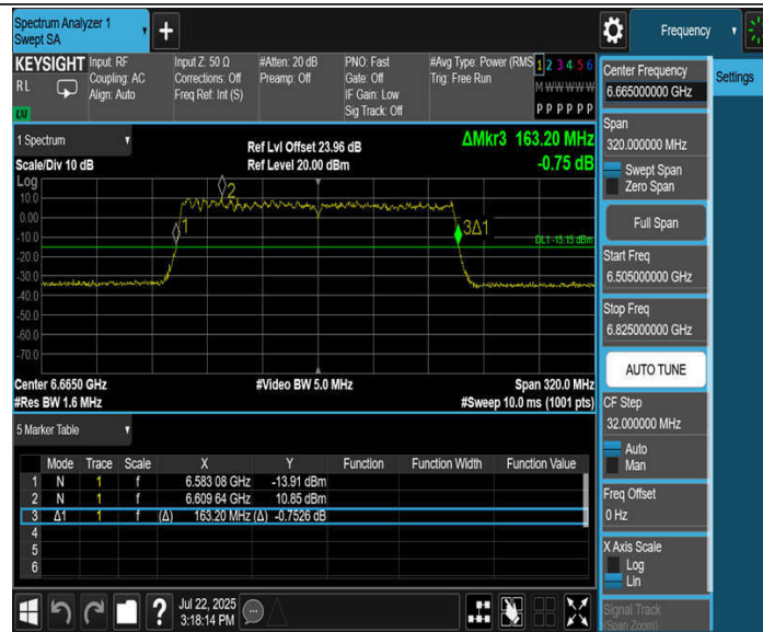
11BE160MIMO_Ant3_6665
