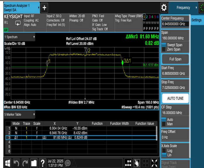
11BE80MIMO_Ant3_6945
