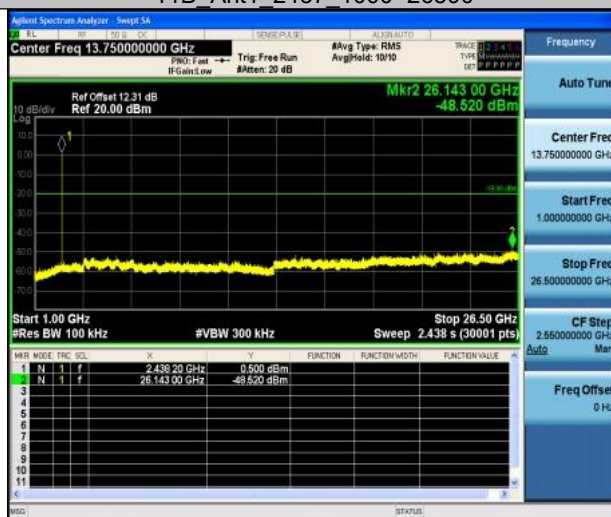
11B_Ant1_2437_1000~26500
