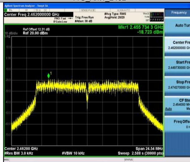
11G_Ant1_2462
