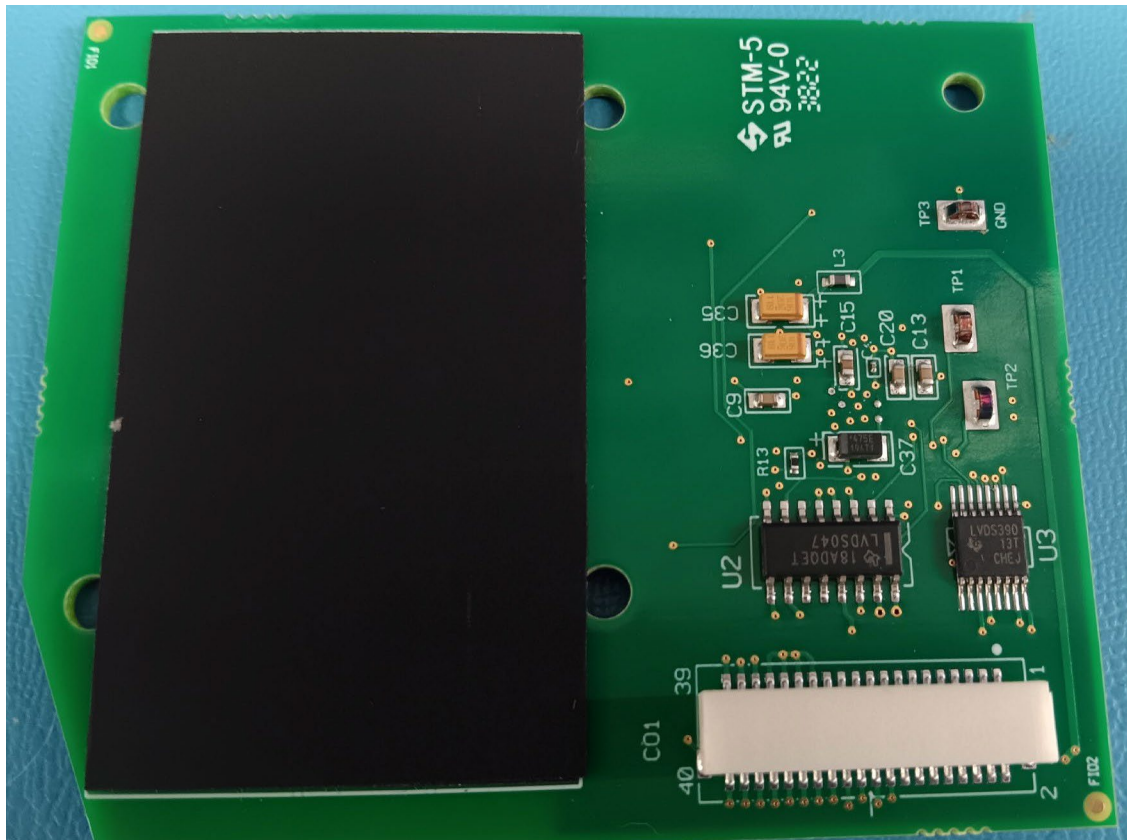
NFC Side 2
