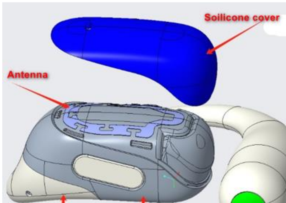
Fig. 9 Antenna
