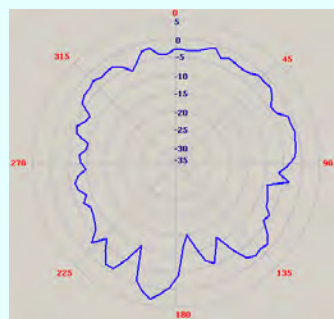
horizontal xy-plane
