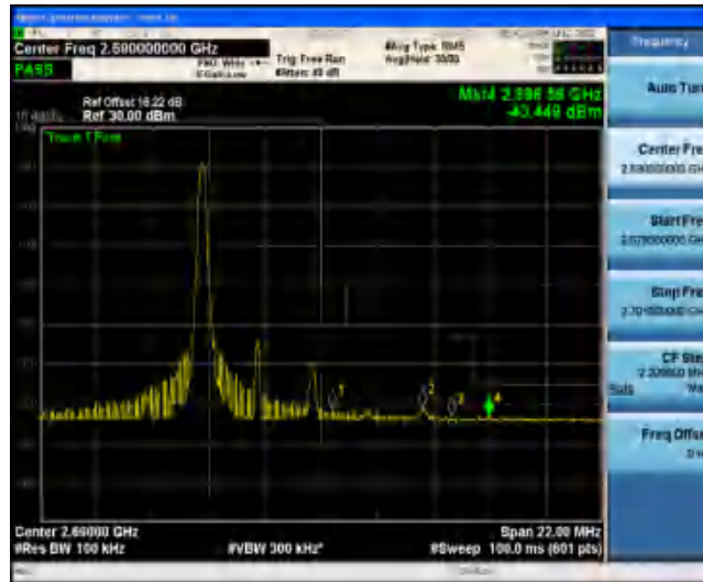
Band41-5MHz-16QAM-41565-1RB#24
