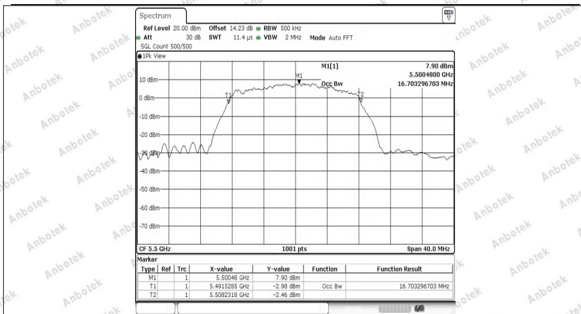
11A-Ant1-5500
