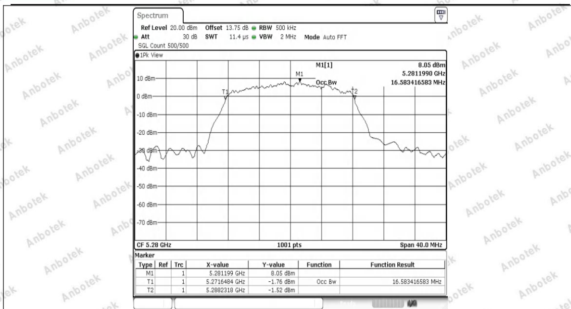
11A-Ant1-5280
