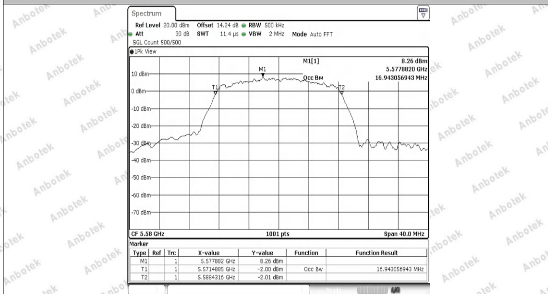
11A-Ant1-5580
