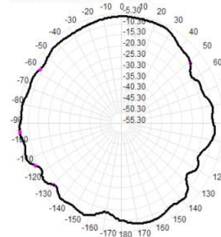
2410.0MHz Total(E1), Max=-5.99dBi
