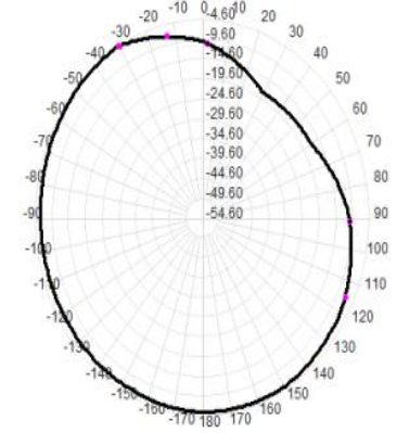
2400.0MHz Total(H), Max=-4.60dBi
