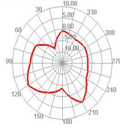
Bluetooth 19 TRP E1
