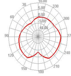
Bluetooth 19 TRP E2
