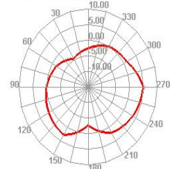
Bluetooth 0 TRP E2
