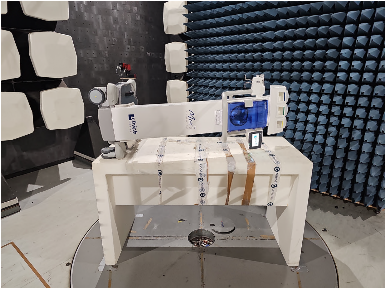
Fig. Mea.: 2 : EUT lying on side
