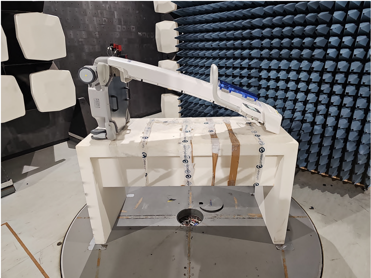
Fig. Mea.: 1 : EUT lying on back
