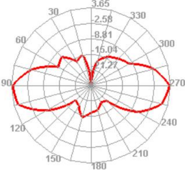
2450.000MHz E1
