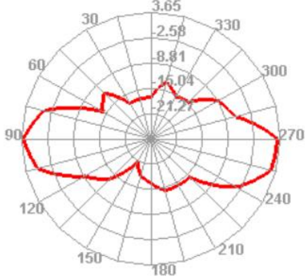
2450.000MHz E2
