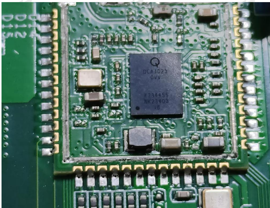
EUT Photo 7
