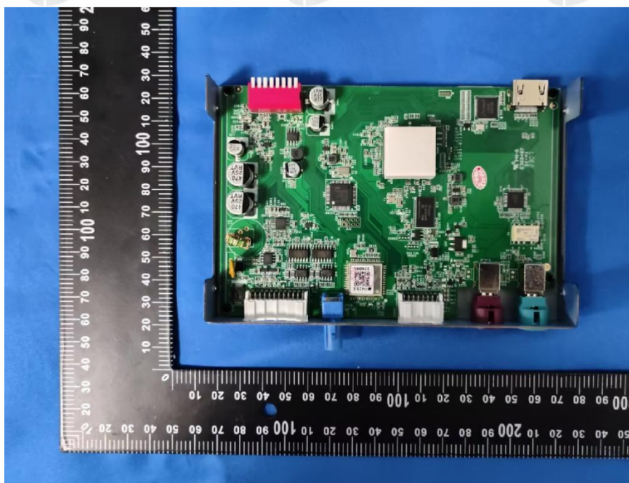
EUT Photo 2
