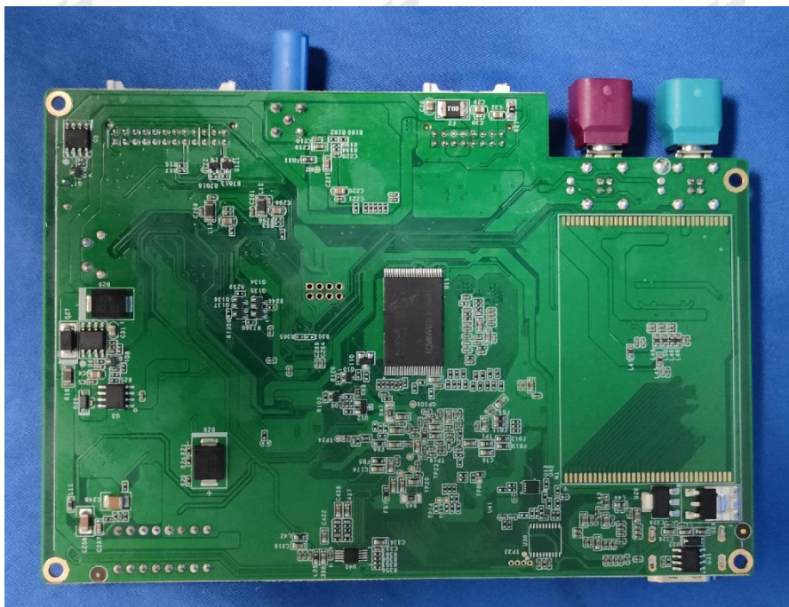
EUT Photo 6
