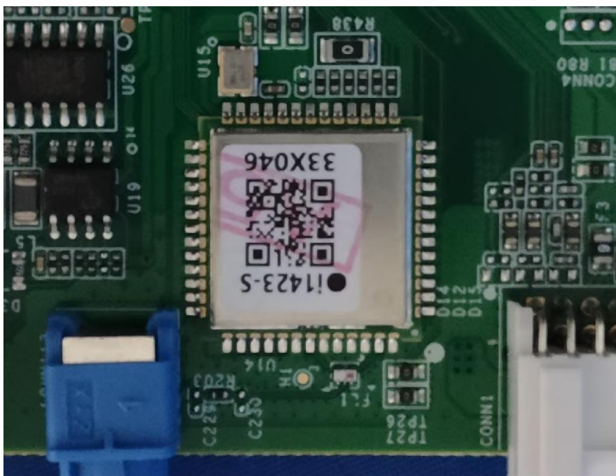
EUT Photo 6
