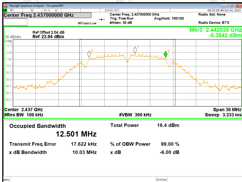
-6dB Bandwidth NTVN b 2437MHz Ant1
