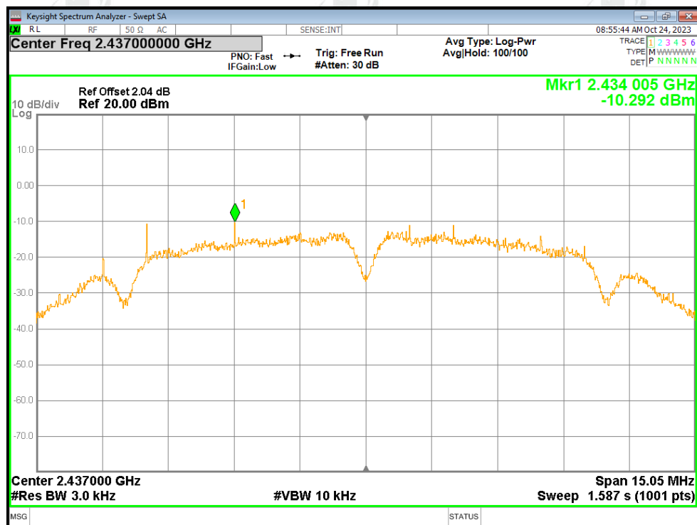
PSD NTVN b 2437MHz Ant1
