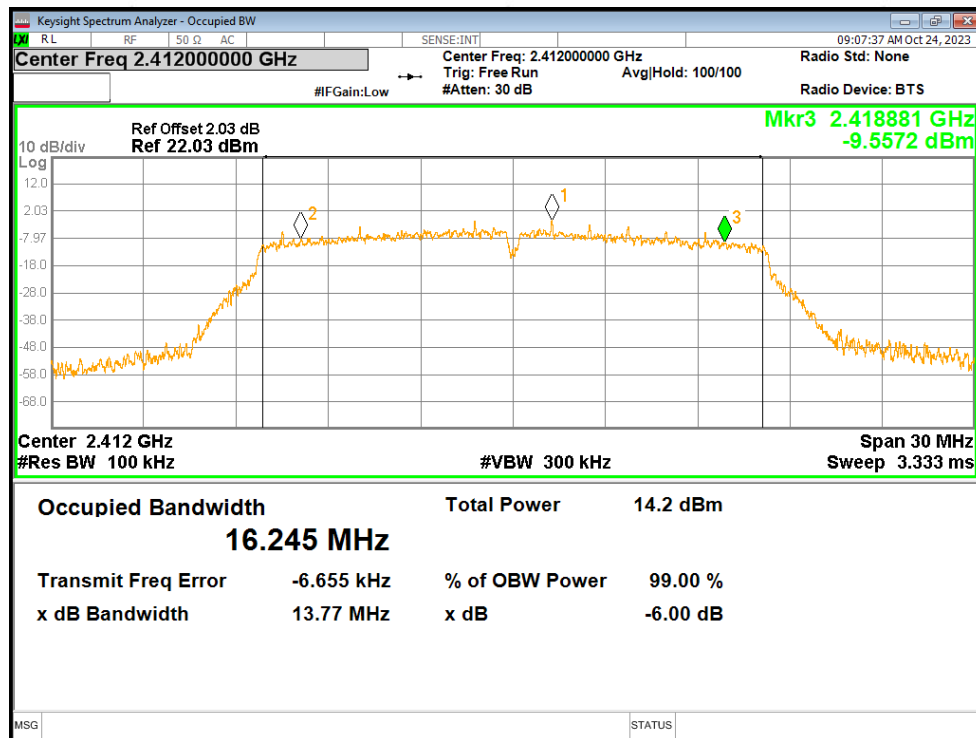
-6dB Bandwidth NTVN g 2412MHz Ant1
