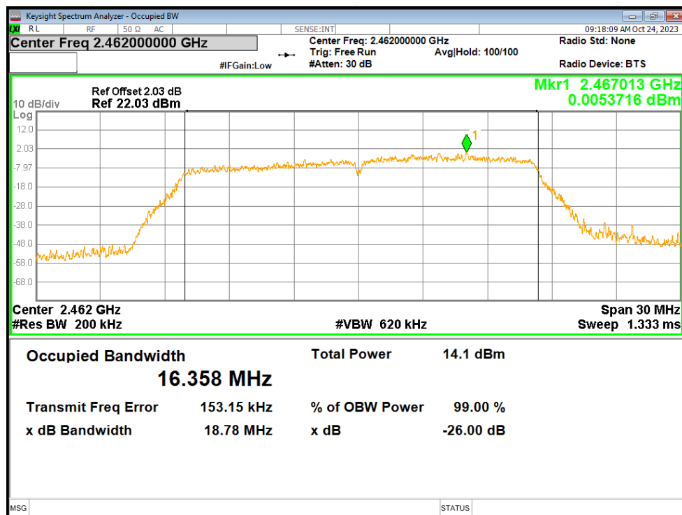
OBW NTVN g 2462MHz Ant1
