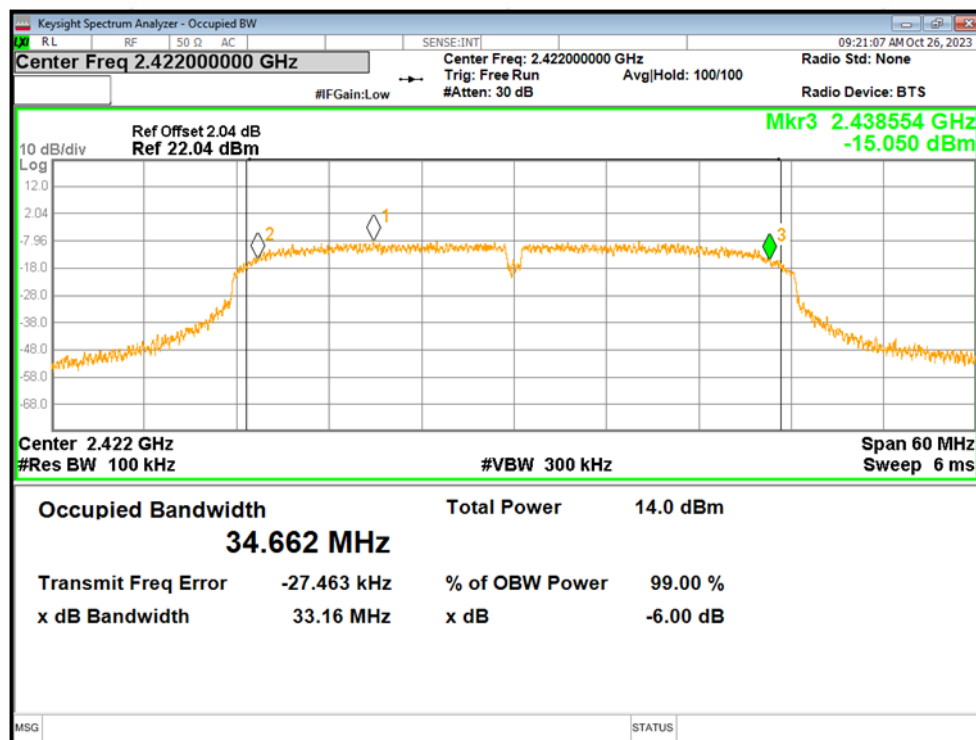
-6dB Bandwidth NTNv n40 2422MHz Ant1
