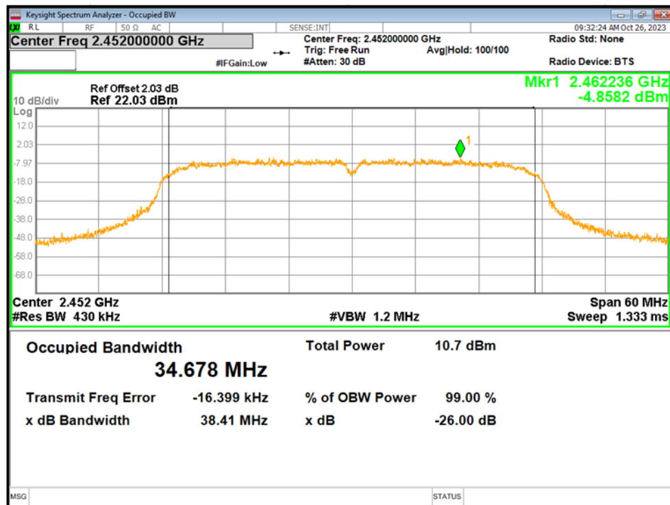
OBW NTV n40 2452MHz Ant1
