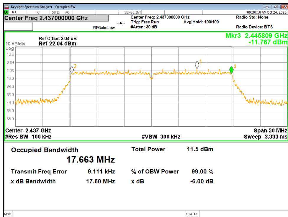
-6dB Bandwidth NTNv n20 2437MHz Ant1
