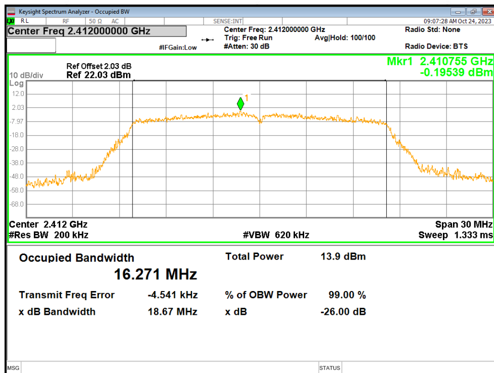
OBW NTVN g 2412MHz Ant1
