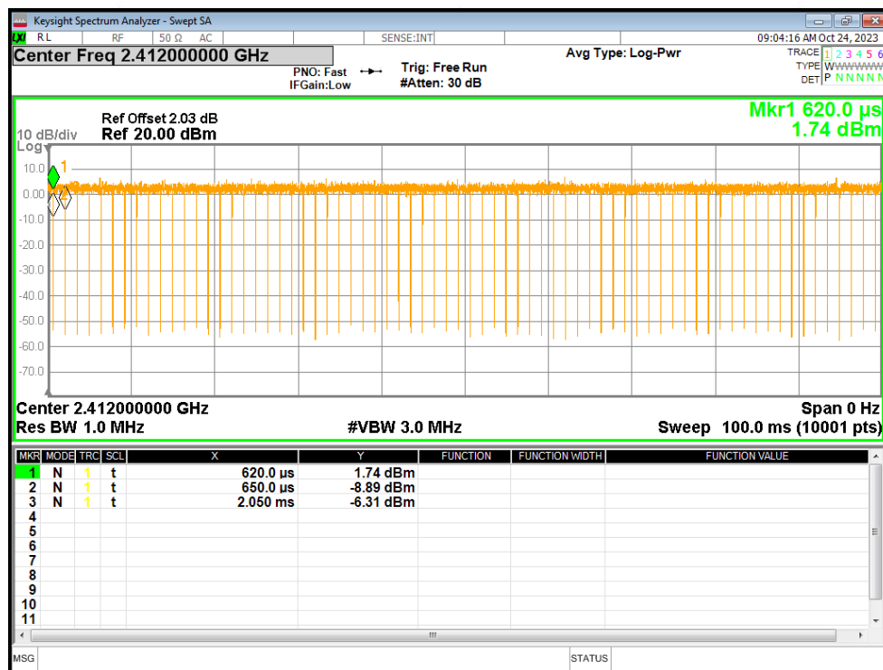
Duty Cycle NTVN g 2412MHz Ant1
