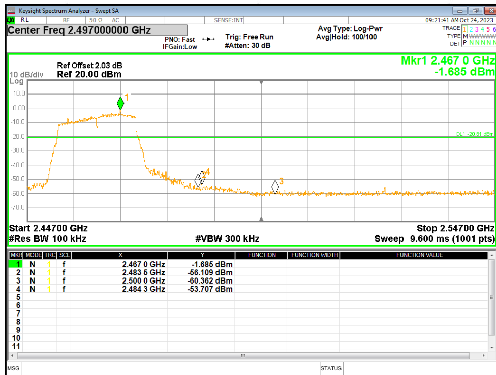
Band Edge NTVN g 2462MHz Ant1 Emission
