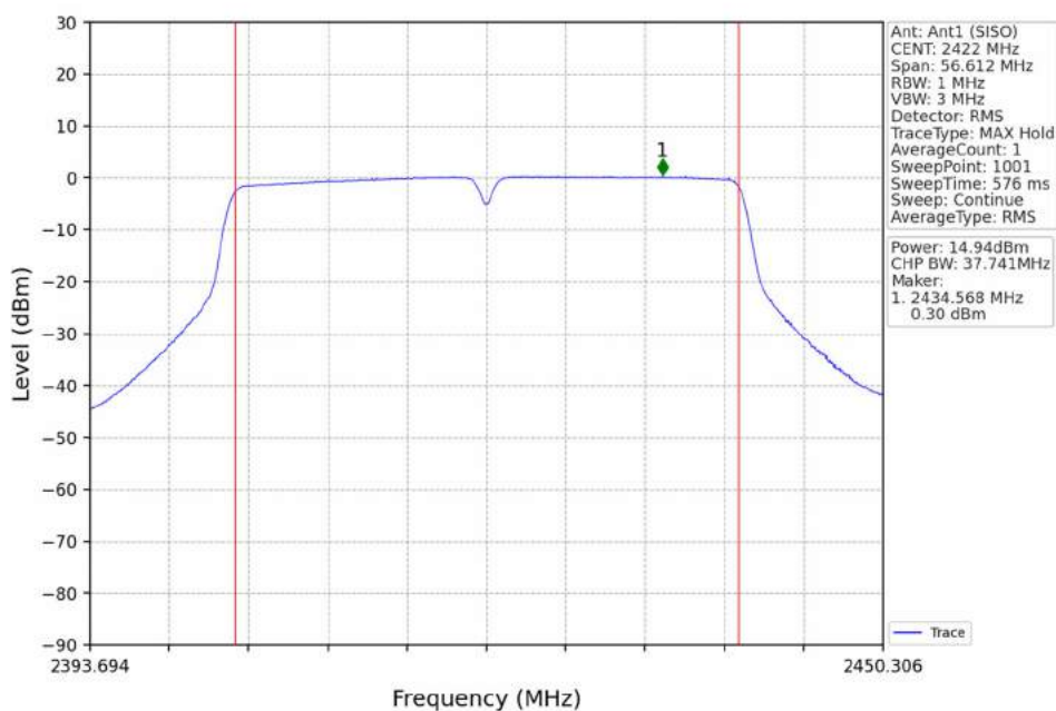
802.11ac(VHT40)_LCH_2422MHz_Ant1 (SISO)_NTNV
