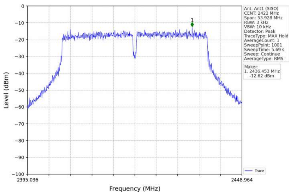
802.11ac(VHT40)_LCH_2422MHz_Ant1 (SISO)_NTNV
