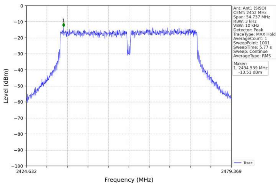
802.11ac(VHT40)_HCH_2452MHz_Ant1 (SISO)_NTNV
