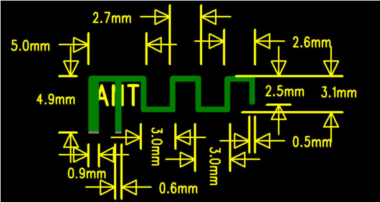
PCB ANT
