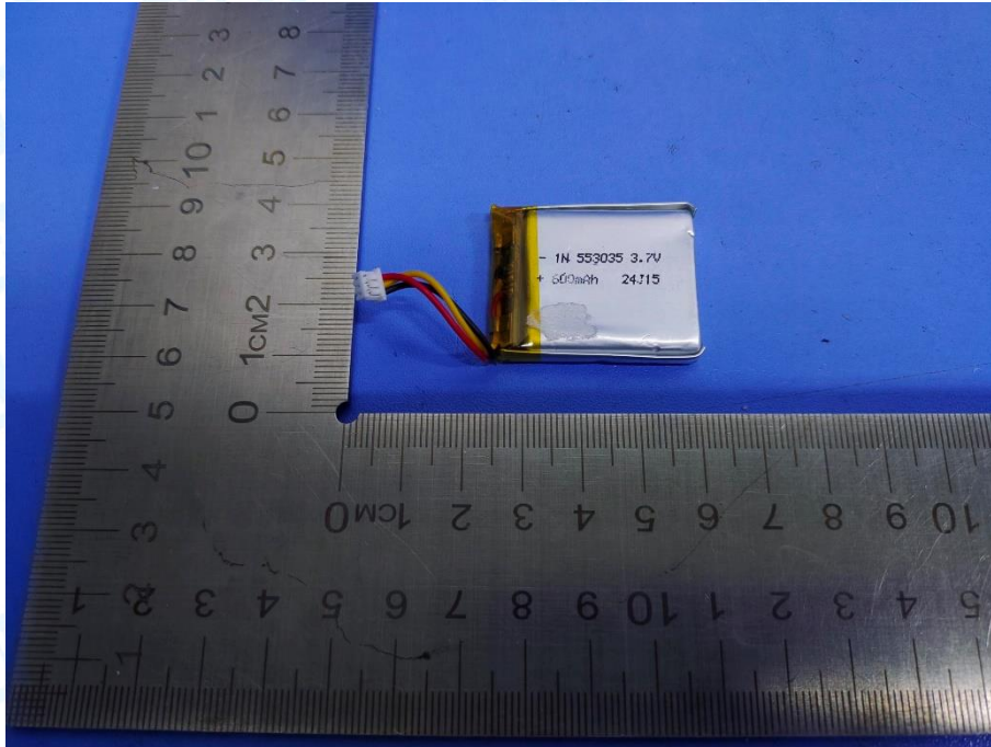
Photo 13 Battery parameters
