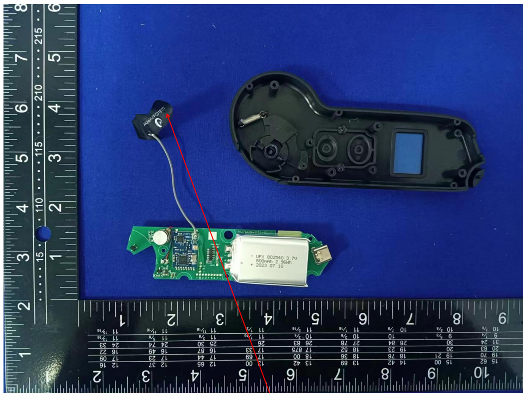
2.4G ANT 1
