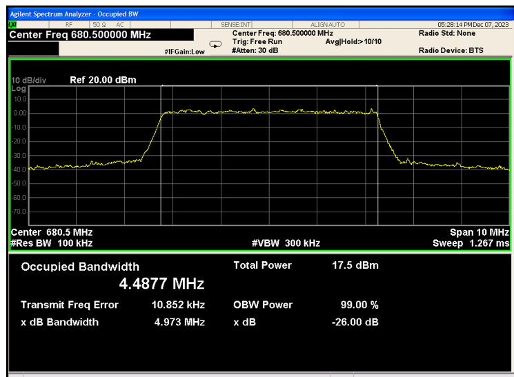
Band71-5MHz-QPSK-133447-25RB#0
