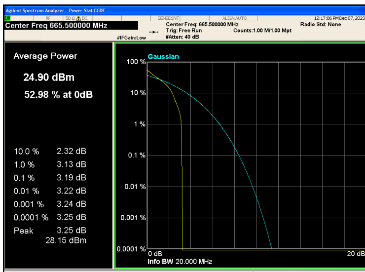
Band71-5MHz-QPSK-133147-25RB#0
