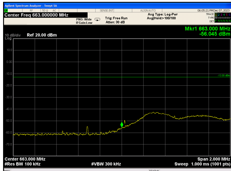
Band71-5MHz-QPSK-133147-25RB#0
