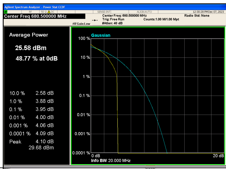
Band71-5MHz-QPSK-133297-1RB#0
