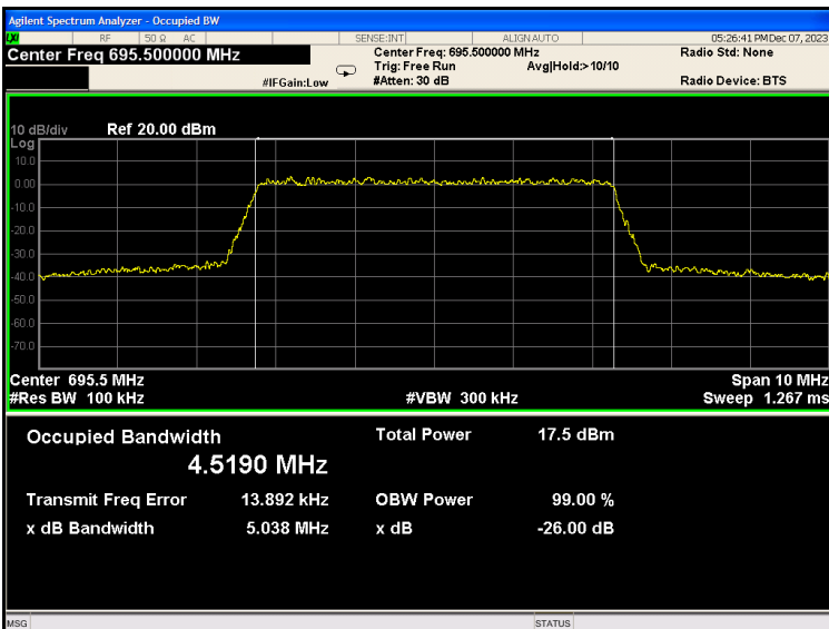
Band71-5MHz-QPSK-133447-25RB#0
