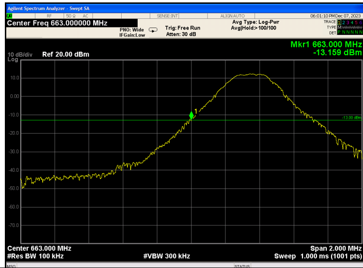
Band71-5MHz-QPSK-133147-1RB#24
