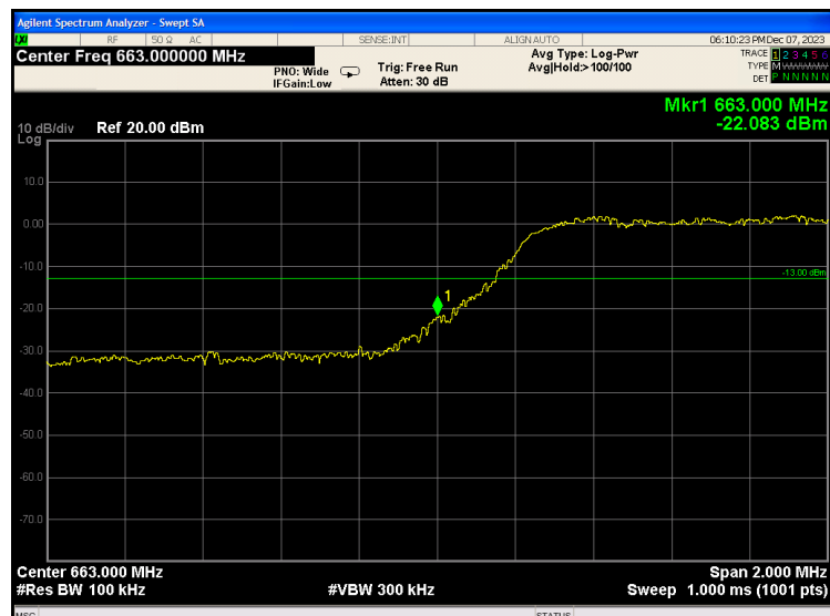
Band71-5MHz-QPSK-133147-25RB#0
