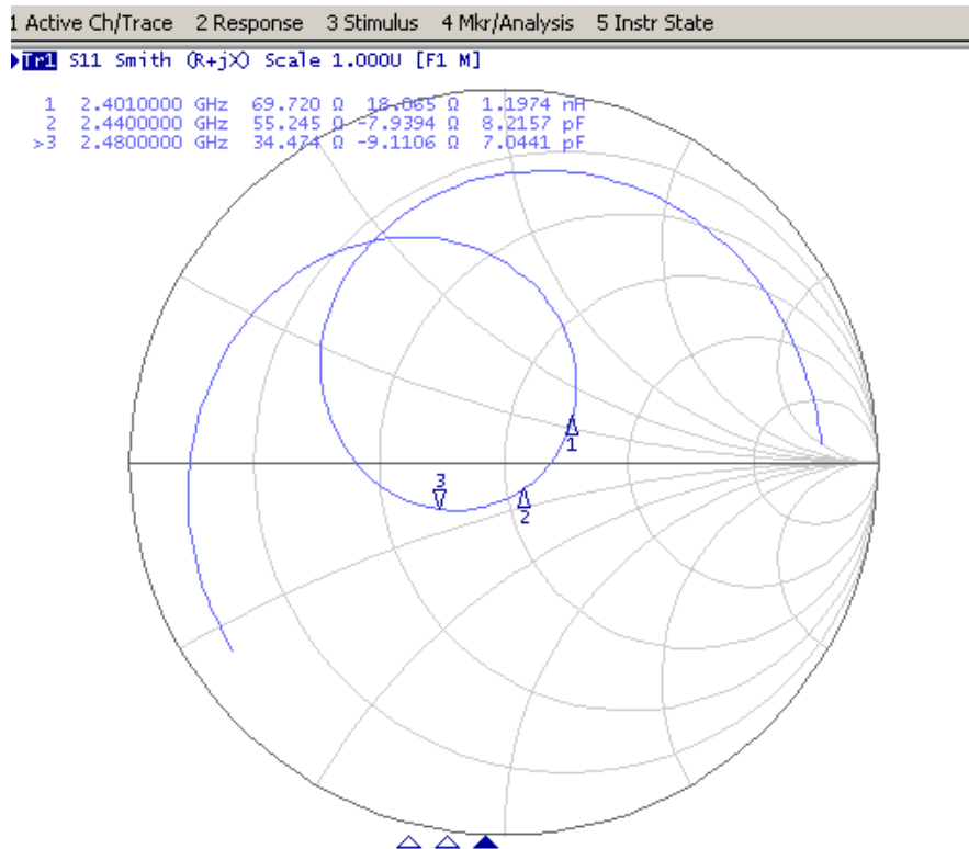
Smith Chart(S11)
