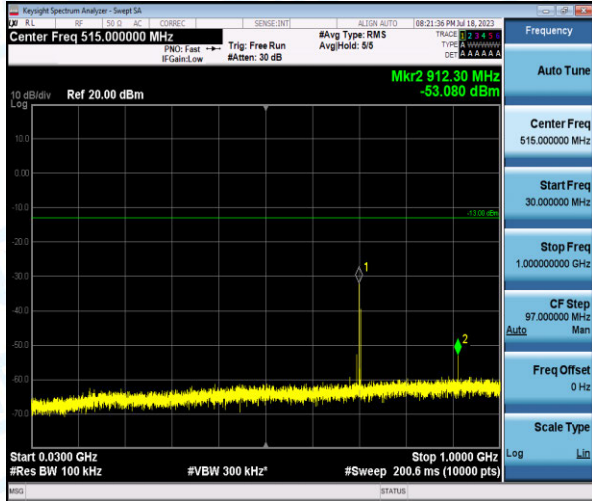
Band12-3MHz-QPSK-23095-1-0-Low-30-1000--53.08-PASS
