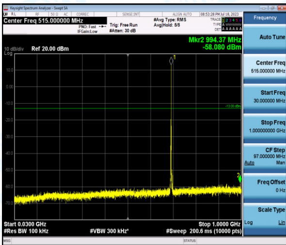
Band12-5MHz-QPSK-23035-1-0-Low-30-1000--58.08-PASS
