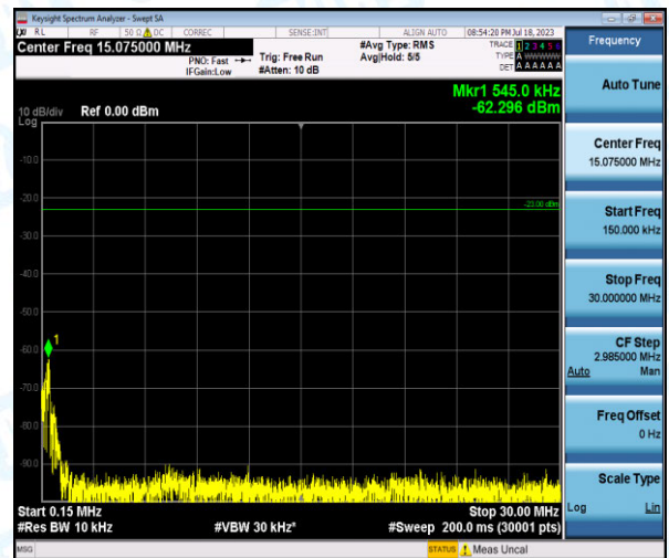
Band12-5MHz-QPSK-23095-1-0-Low-0.15-30--62.3-PASS
