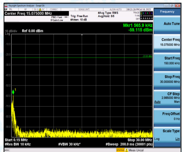
Band12-3MHz-QPSK-23095-1-0-Low-0.15-30--59.12-PASS
