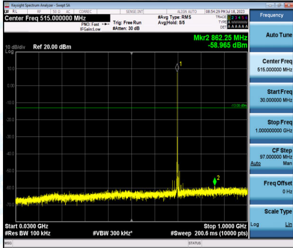
Band12-5MHz-QPSK-23095-1-0-Low-30-1000--58.97-PASS
