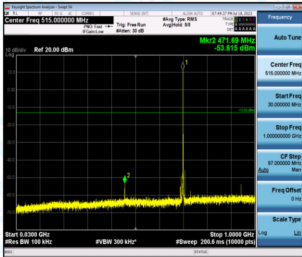
Band12-1.4MHz-QPSK-23095-1-0-Low-30-1000--53.82-PASS
