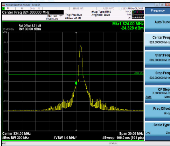
Band26-15MHz-QPSK-26865-1-0-Low--24.33-PASS
