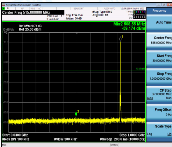
Band26-3MHz-QPSK-26805-1-0-Low-30-1000--59.17-PASS
