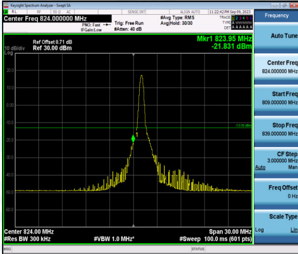
Band26-15MHz-16QAM-26865-1-0-Low--21.83-PASS
