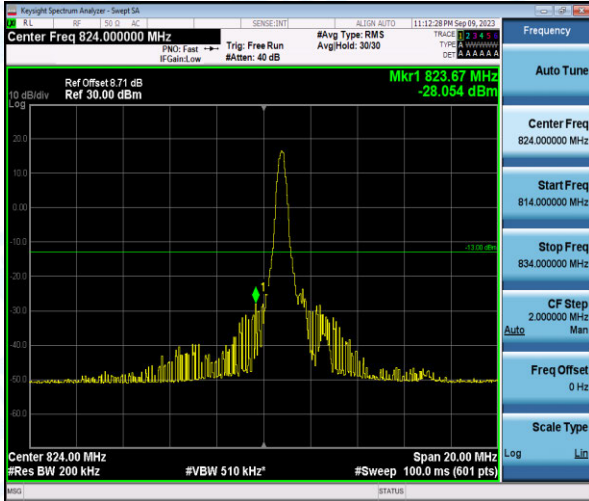
Band26-10MHz-QPSK-26840-1-0-Low--28.05-PASS
