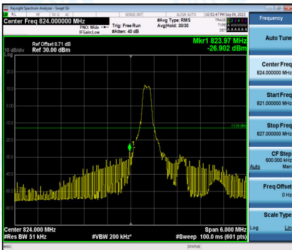
Band26-3MHz-QPSK-26805-1-0-Low--26.90-PASS
