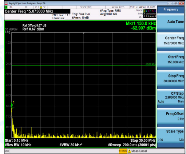
Band26-10MHz-QPSK-26740-1-0-Low-0.15-30--63-PASS
