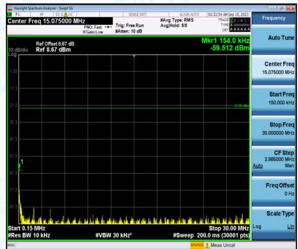
Band26-5MHz-QPSK-26740-1-0-Low-0.15-30--59.51-PASS
