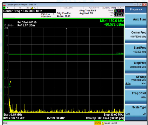
Band26-3MHz-16QAM-26740-1-0-Low-0.15-30--60.57-PASS
