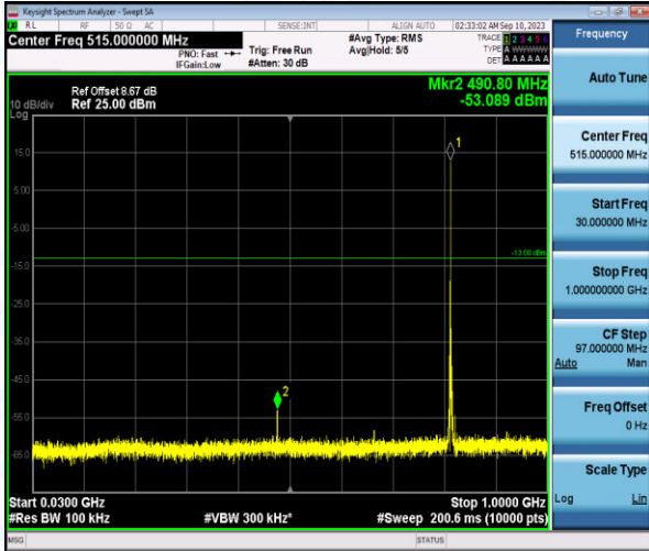
Band26-5MHz-QPSK-26740-1-0-Low-30-1000--53.09-PASS
