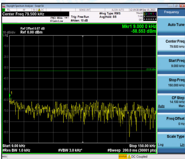
Band26-3MHz-QPSK-26740-1-0-Low-0.009-0.15--58.55-PASS
