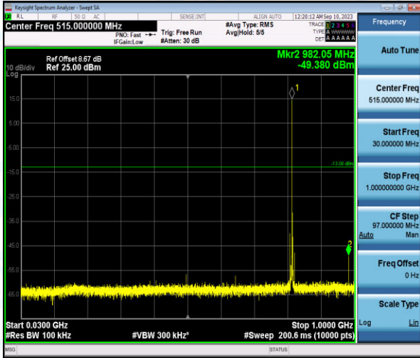
Band26-3MHz-16QAM-26740-1-0-Low-30-1000--49.38-PASS
