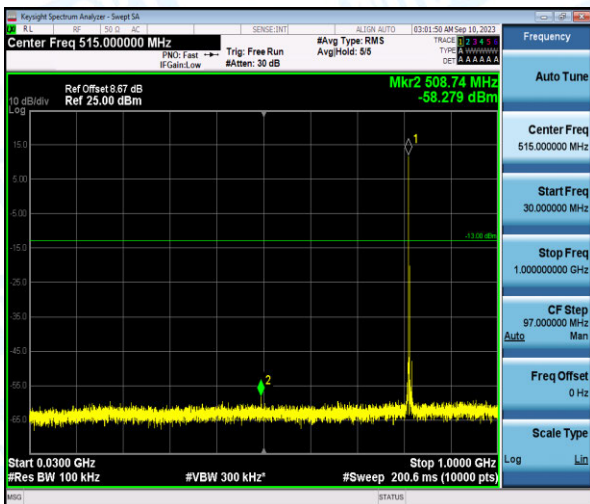
Band26-10MHz-QPSK-26740-1-0-Low-30-1000--58.28-PASS
