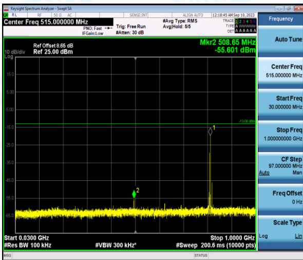
Band26-3MHz-QPSK-26705-1-0-Low-30-1000--55.6-PASS
