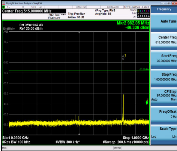
Band26-3MHz-QPSK-26740-1-0-Low-30-1000--46.34-PASS
