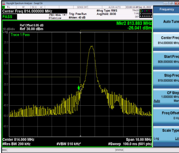
Band26-10MHz-QPSK-26740-1-0-Low--26.84,-26.04-PASS
